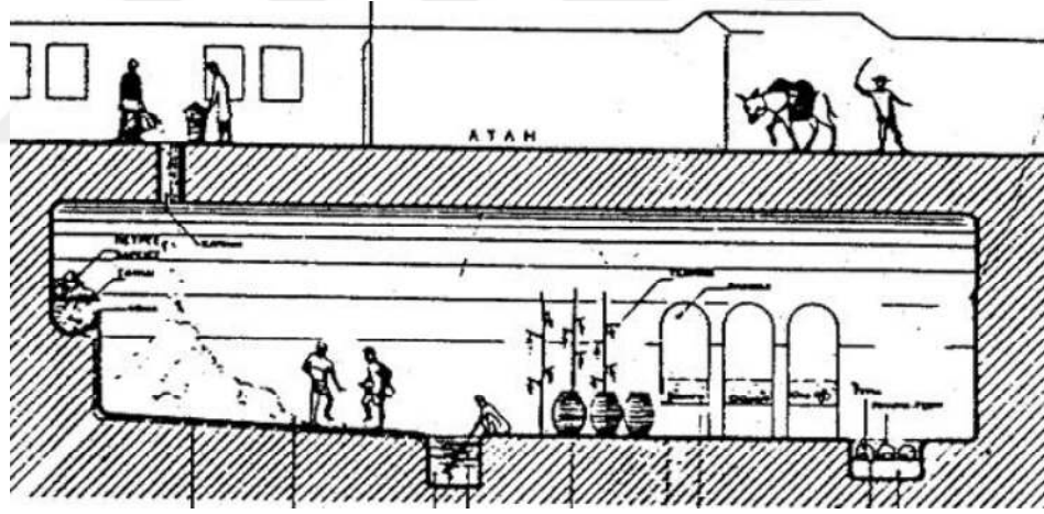
ŞEKİL 59. Bir şirahane kesiti (Sinasos in Cappadocia, 1924)
