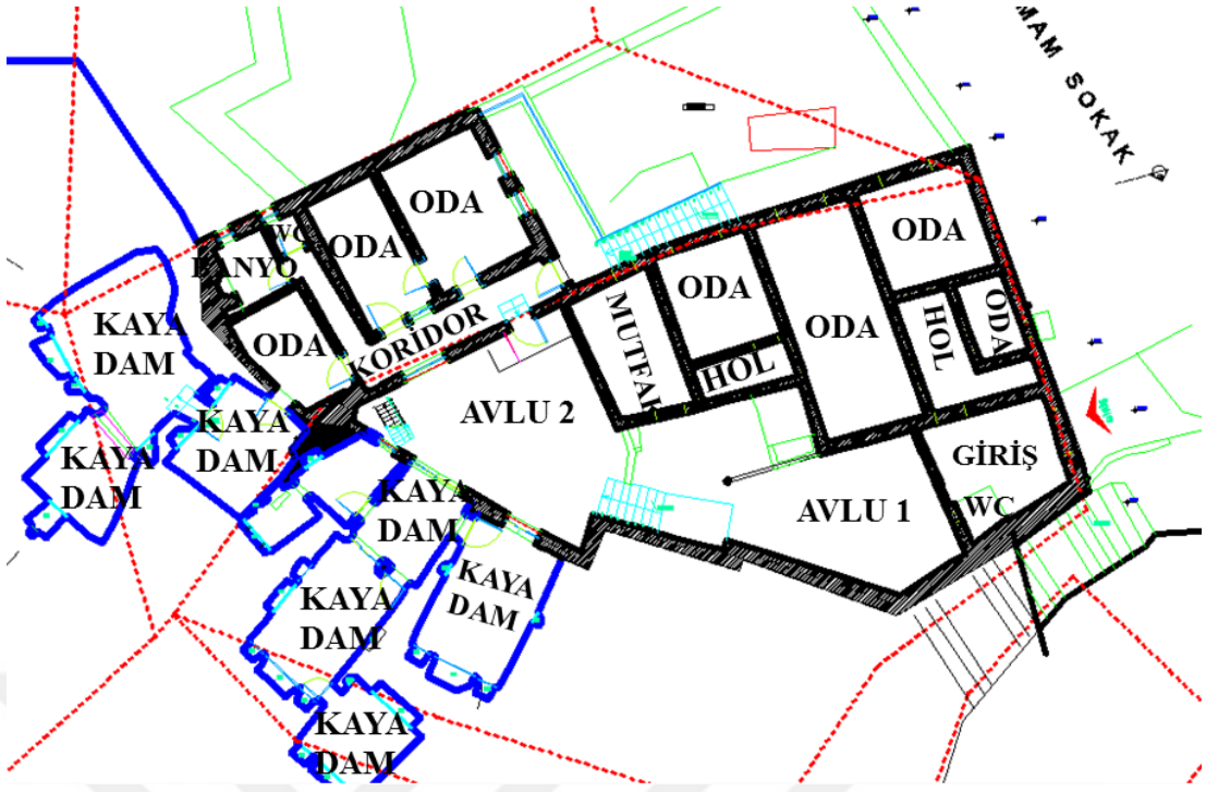
ŞEKİL 74.A. Erdoğan Yaman Evi-Restorasyon öncesi (Kabaltı Mimarlık Ltd. Şti. 2015)
