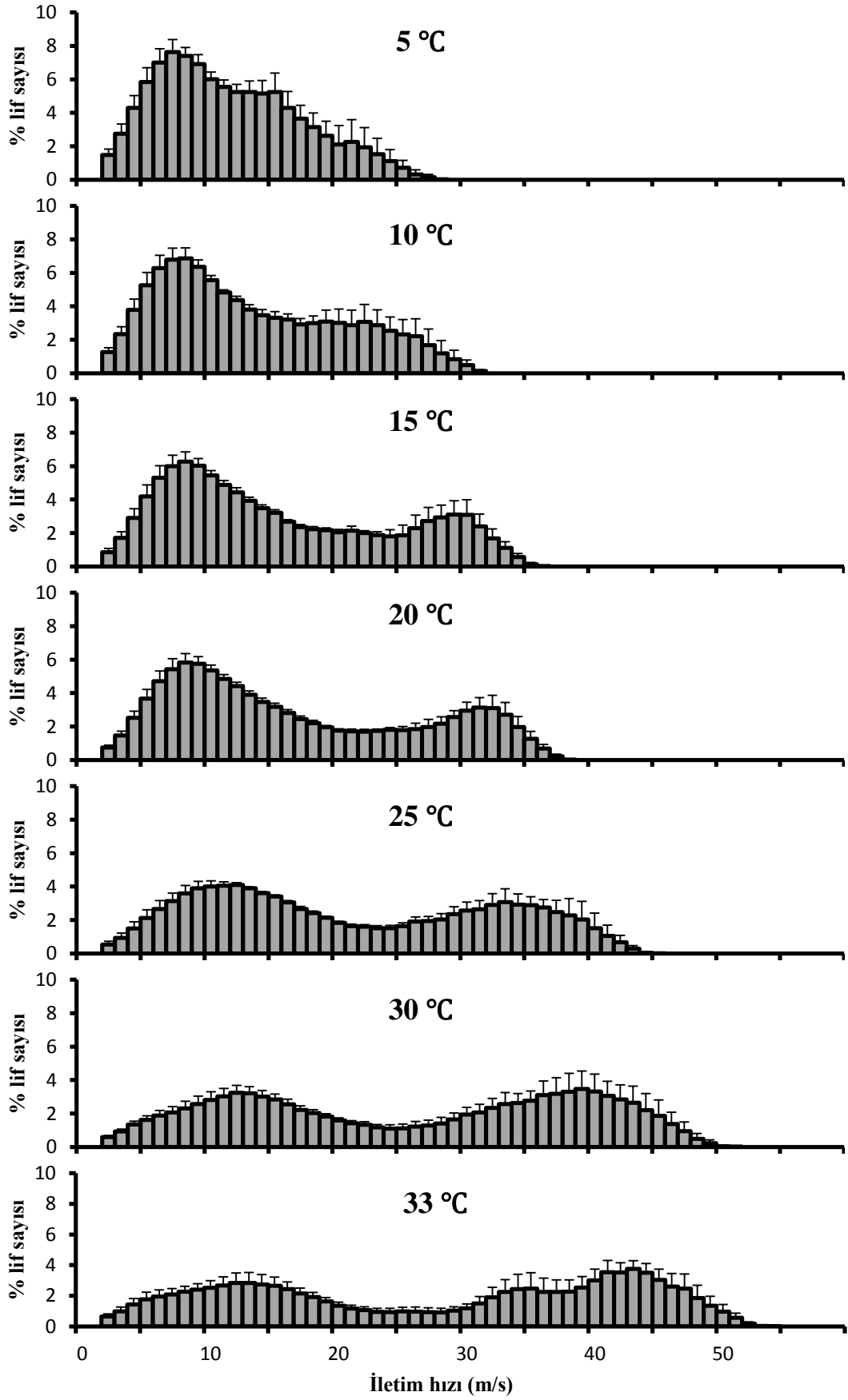
Şekil 4.7. Barker metoduyla elde edilen farklı sıcaklıklardaki iletim hızı dağılımları.
