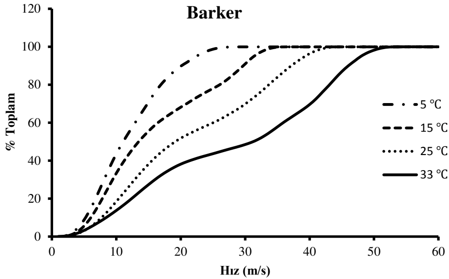
Şekil 4.8. Barker metoduyla elde edilen farklı sıcaklıklardaki iletim hızı kümülatif dağılımları.
