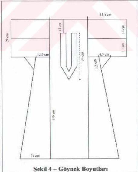
Şekil 4 – Göynek Boyutları
