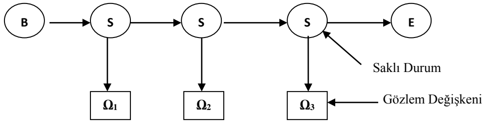
Şekil 2.7 Saklı Markov Modelinin Genel Yapısı
