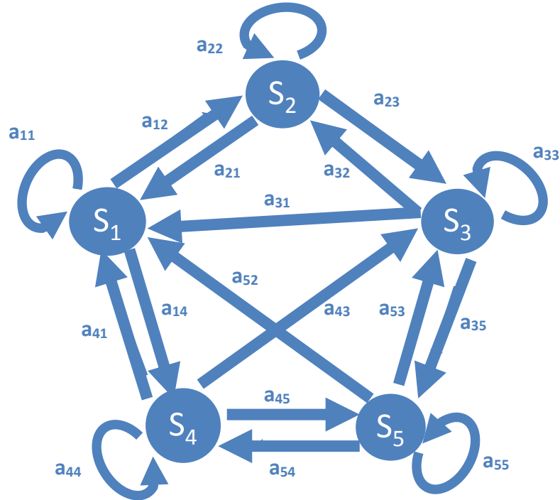
Şekil 2.2 Durumlu Bir Markov Zinciri Örneği Kaynak : (Semerci, 2006)
