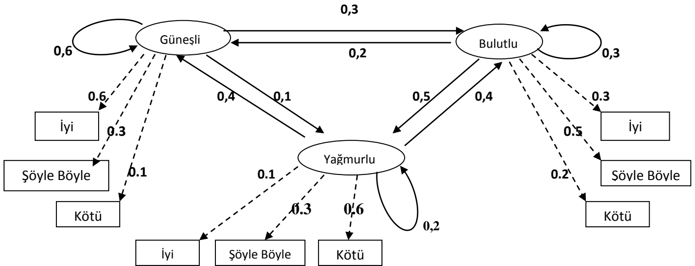
Şekil 2.6 Saklı Markov Model Örneği Kaynak : (Ibe, 2009)
