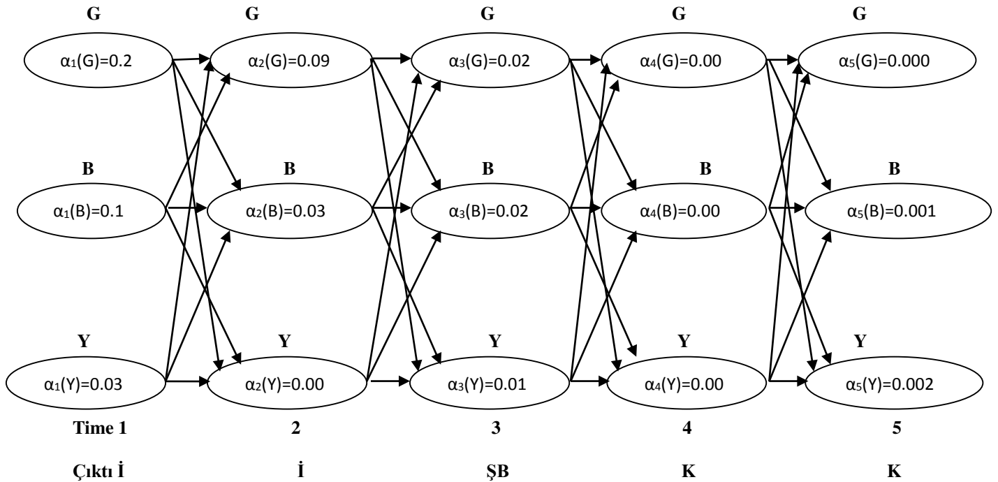
Şekil 2.11 Şekil 2.6'daki Örneğin Kafes İşi
