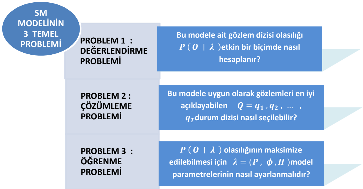
Şekil 2.8 Saklı Markov Modelinin 3 Temel Problemi
