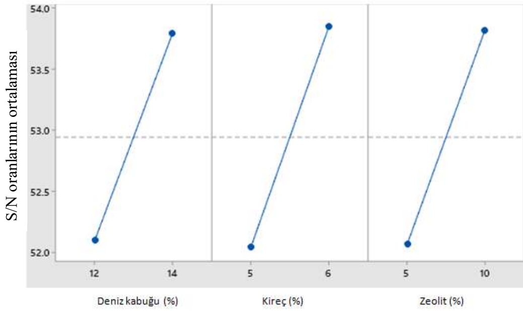
Şekil 51. 1 günlük serbest basınç mukavemeti sonuçlarının katkı yüzdeleri – S/N oranlarının ortalaması analizi
