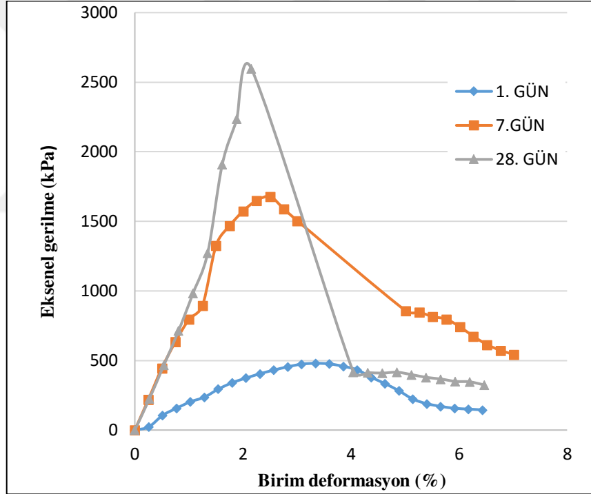
Şekil 46. SD12K6Z10 karışımının eksenel gerilme- birim deformasyon grafiği
