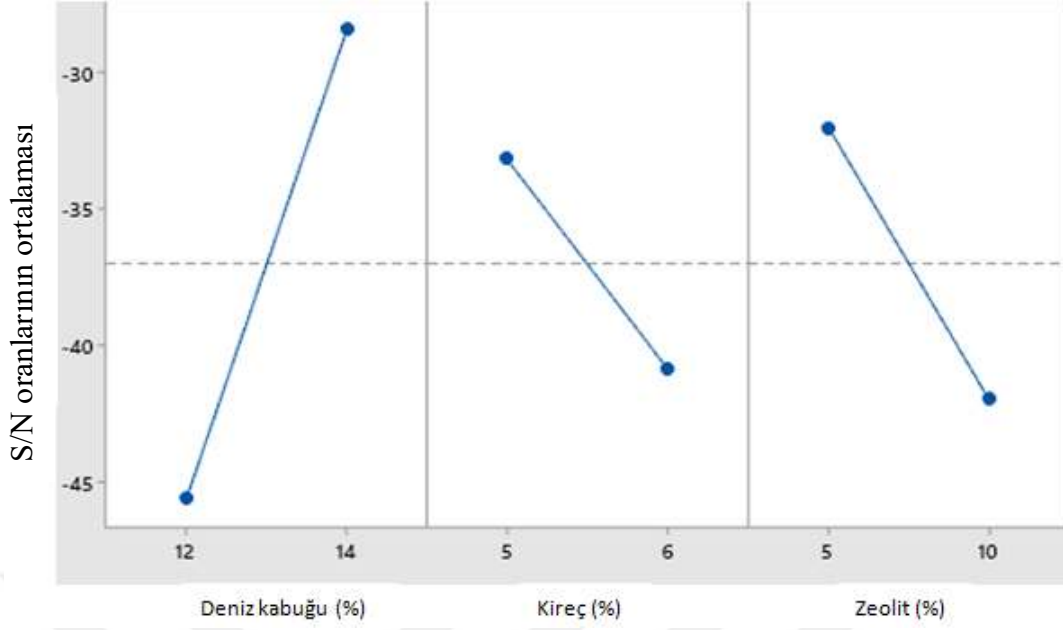
Şekil 55. Şişme basıncı sonuçlarının katkı yüzdeleri – S/N oranlarının ortalaması analizi
