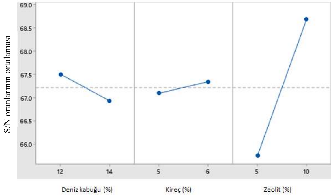
Şekil 53. 28 günlük serbest basınç mukavemeti sonuçlarının katkı yüzdeleri - S/N oranlarının ortalaması analizi
