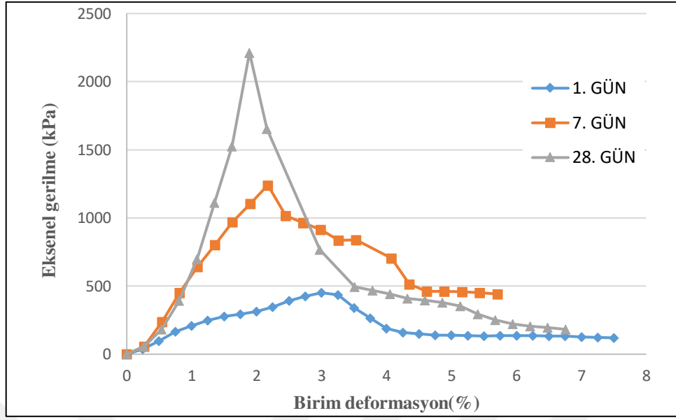
Şekil 49. SD14K5Z10 karışımının eksenel gerilme- birim deformasyon grafiği
