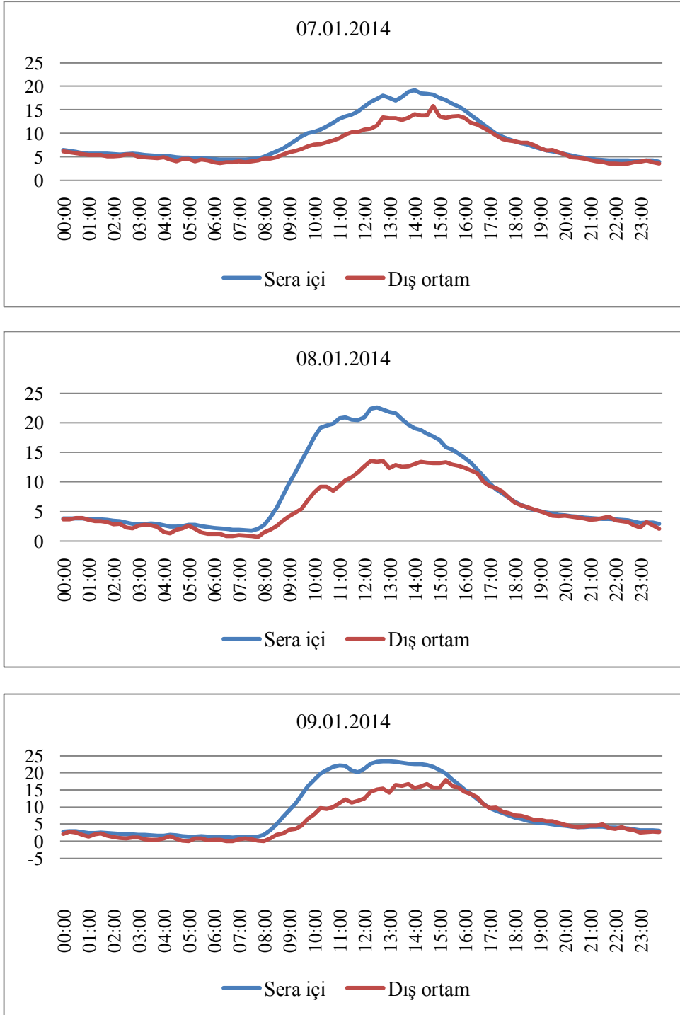
Şekil 4.2. Günlere göre saatlik sera ve dış ortam sıcaklık değişimi (devam)
