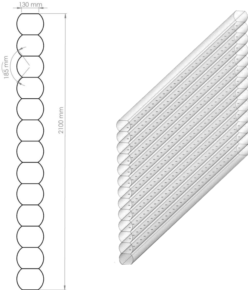
Şekil 3.10. Düşey düzlem örtüleri model ve kesit görünümü
