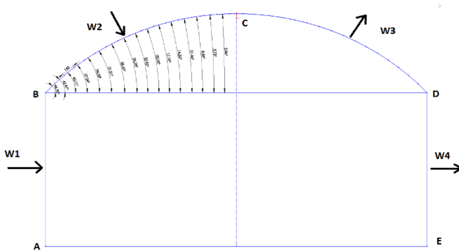
Şekil 3.30. Sera üzerine gelen rüzgâr yükleri
