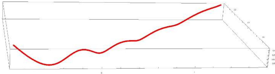
Şekil 5.1: \gamma timelike rektifiyan eğrisinin, Minkowski 3-uzayına stereografik izdüşümü
