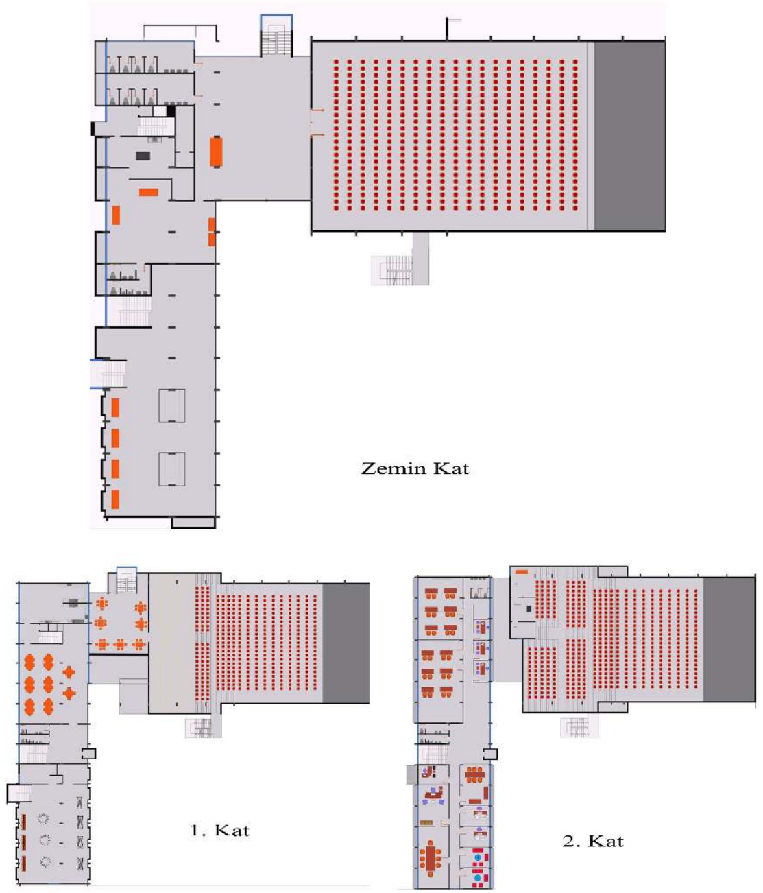
Görsel 85. Emek Sineması'nın Kat Planları, 2022 (Uğur Tuztaş'ı Koleksiyonu).
