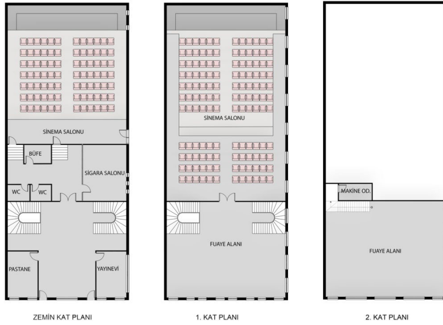
Görsel 13. Tan Sineması Kat Krokileri, 2022 (Uğur Tuztaş Koleksiyonu).
