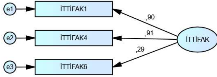
Şekil 8. İttifak ve Dönüşüm Ölçeği DFA Şeması
