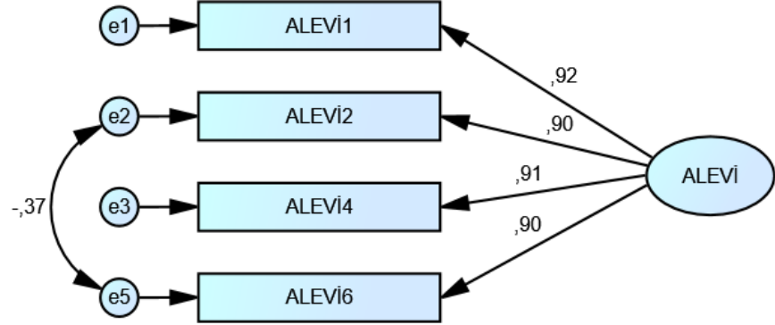
Şekil 9. Alevi Açılımı ve Dönüşüm Ölçeği DFA Şeması
