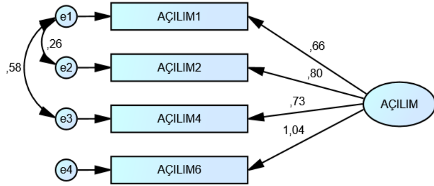
Şekil 5. Açılım ve Dönüşüm Ölçeği DFA Şeması
