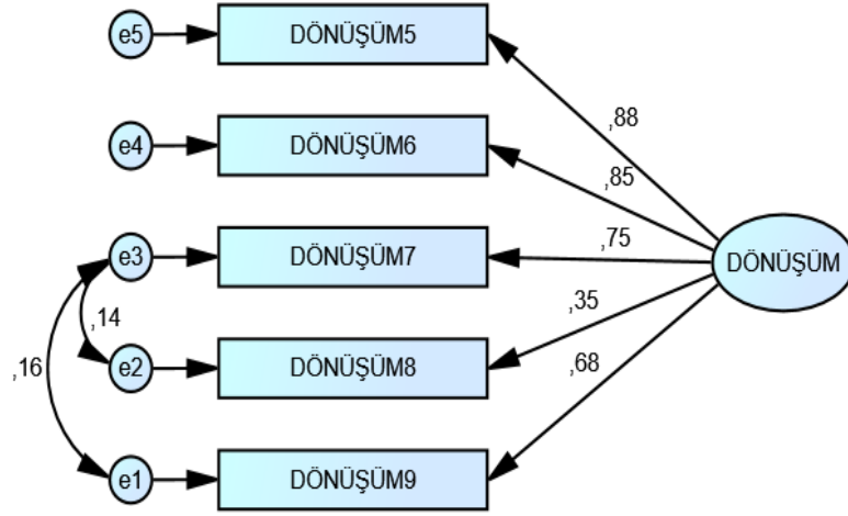
Şekil 1. Dönüşüm Algısı Ölçeği DFA Şeması
