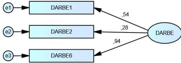
Şekil 6. Darbe ve Dönüşüm Ölçeği DFA Şeması
