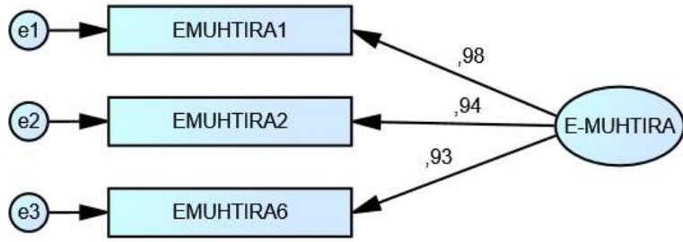
Şekil 2. E-Muhtıra ve Dönüşüm Ölçeği DFA Şeması
