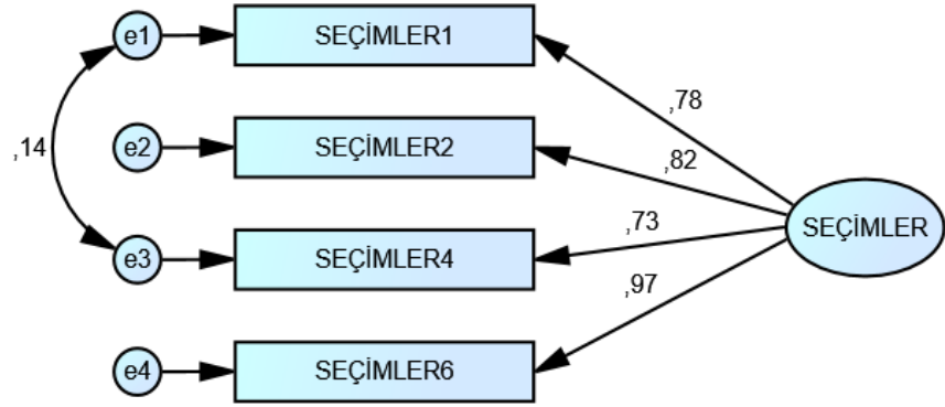
Şekil 4. 2015 Haziran Seçimleri ve Dönüşüm Ölçeği DFA Şeması
