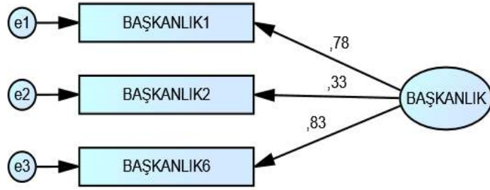
Şekil 7. Başkanlık ve Dönüşüm Ölçeği DFA Şeması
