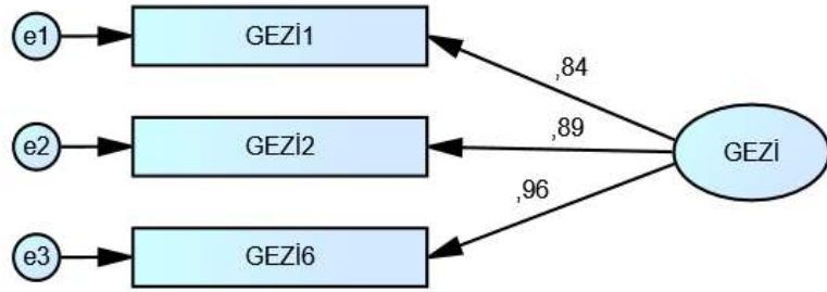
Şekil 3. Gezi ve Dönüşüm Ölçeği DFA Şeması
