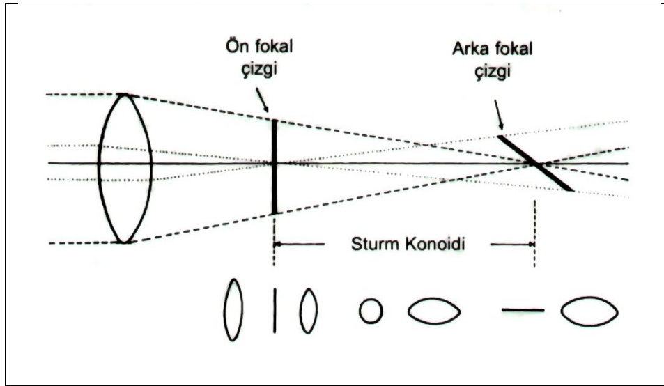
Şekil 4: Sturm Konoidi (3).
