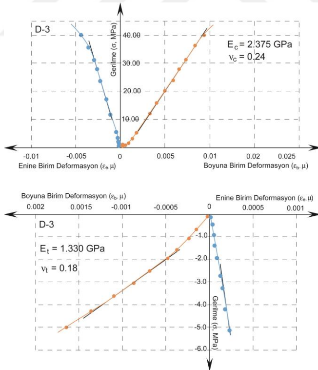
Şekil 6.14. D-3 numaralı örneklere ait \sigma - \varepsilon grafikleri
