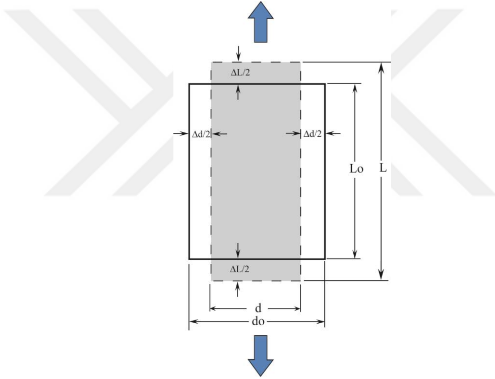
Şekil 5.10. Doğrudan çekme dayanımı deneyi sırasında meydana gelen boyuna ve enine deformasyonların şematik gösterimi
