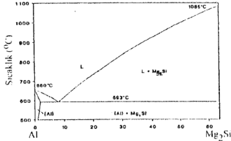
Şekil 4.4. Al-Mg 2 Si faz diyagramı [118].
