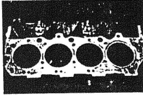
Şekil 2.4. Partikül takviyeli Al matrisli kompozit malzemedan üretilmiş silindir gömleklerine sahip Al motor bloğu(Allison,1993).
