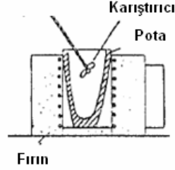
Şekil 5.1 Takviye partiküllerin sıvı matrise karıştırılması için kullanılan düzeneğin şematik resmi.
