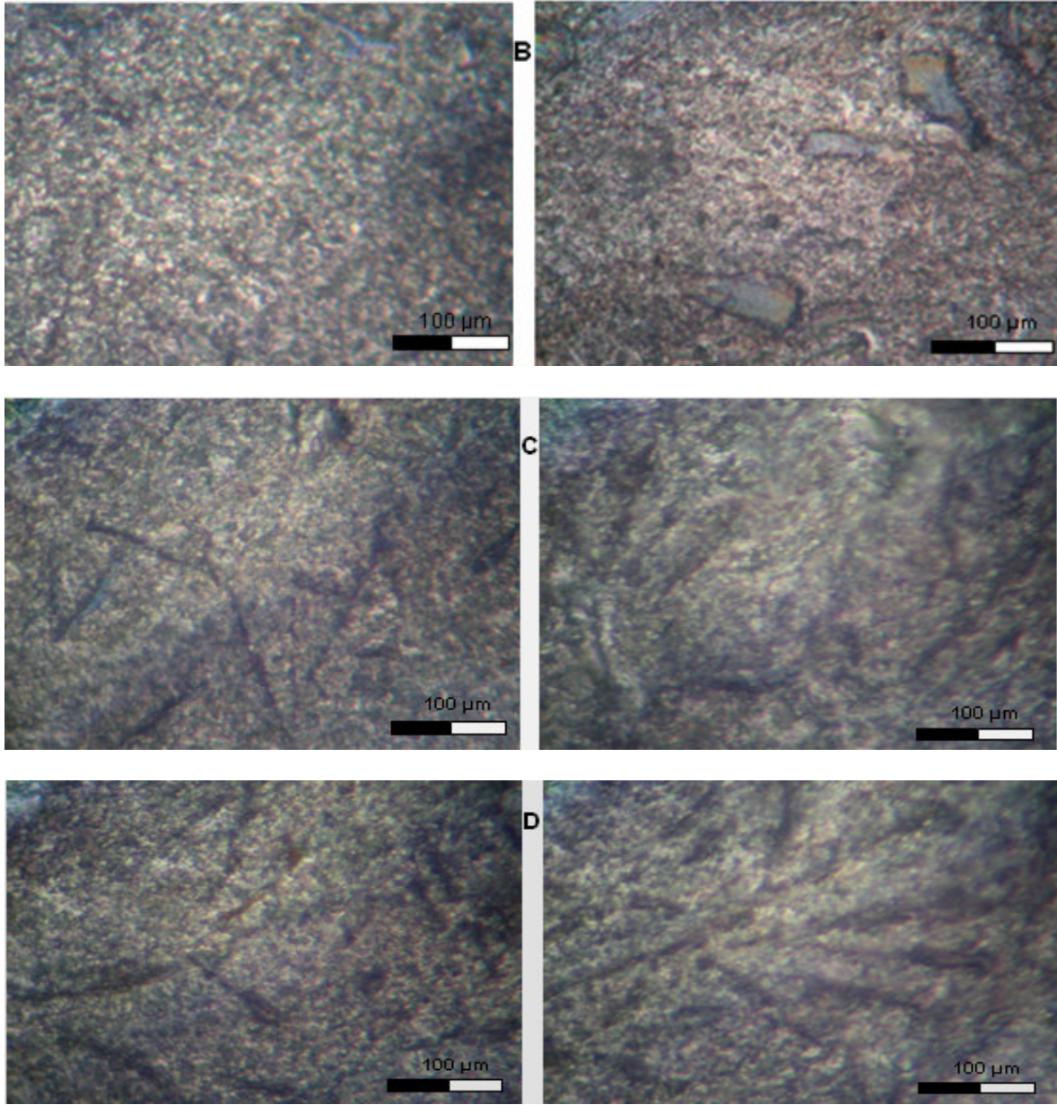
Şekil 6.8 100 µm % 5, 10, 15, 20 hacim oranlarına sahip numunelerin mikroyapı fotoğrafları.
