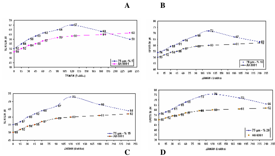
Şekil 6.16 75 µm boyutunda takviyeye sahip numunelerin homojenizasyon sırasında sertlik değişimleri.
