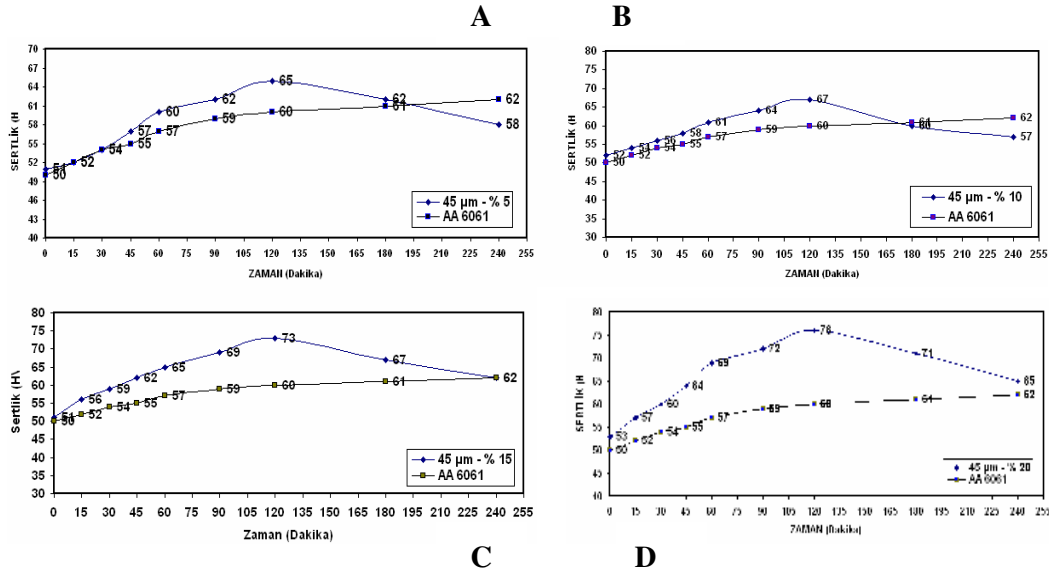
Şekil 6.15 45 µm boyutunda takviyeye sahip numunelerin homojenizasyon sırasında sertlik değişimleri.
