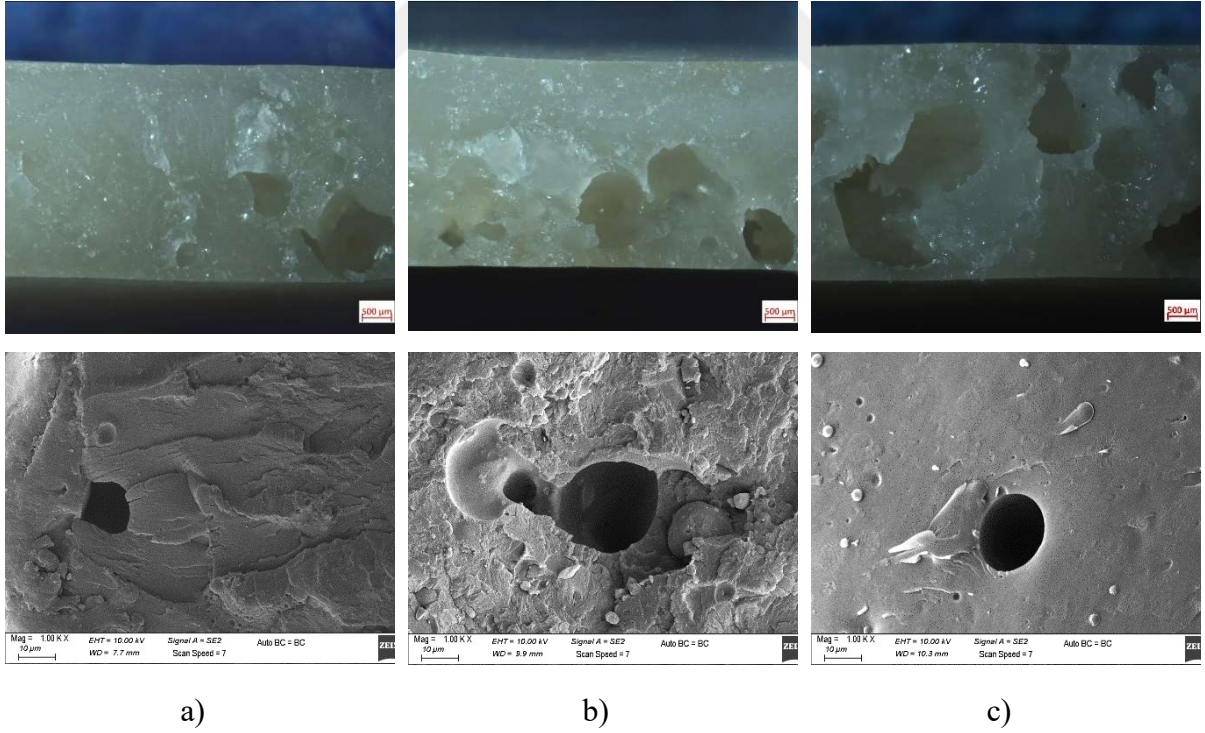
Şekil 3.43 : a) PLA/PA6 (70:30)+%1 KKA, b) PLA/PA6 (70:30)+%1,5 KKA ve c) PLA/PA6 (70:30)+%2 KKA karışımlarının stereo mikroskop ve SEM görüntüleri.
