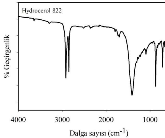
Şekil 2.5 : “Hydrocerol 822” kodlu köpürtücü ajanın FT-IR spektrumu.
