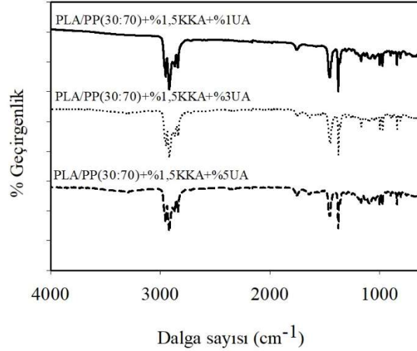
Şekil 3.51 : Farklı oranlarda UA içeren PLA/PP+%1,5 KKA karışımların FT-IR spektrumları.
