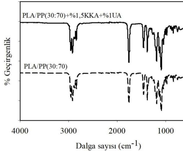
Şekil 3.63 : PLA/PP (30:70) ve köpürtücü ile uyumlaştırıcı ajan katkılı PLA/PP (30:70) karışımlarının FT-IR spektrumları.
