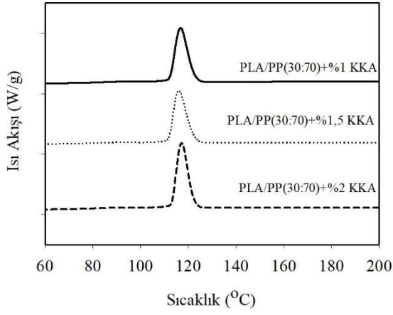
Şekil 3.29 : Farklı oranlarda KKA içeren PLA/PP (30:70) karışımlarının, a) birinci ısıtma, b) soğutma ve c) ikinci ısıtma geçişlerine ilişkin DSC termogramları.
