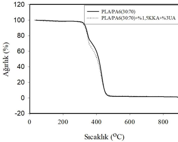
Şekil 3.70 : PLA/PA6 (30:70) ve köpürtücü ile uyumlaştırıcı ajan katkılı PLA/PA6 (30:70) karışımlarının TGA termogramları.
