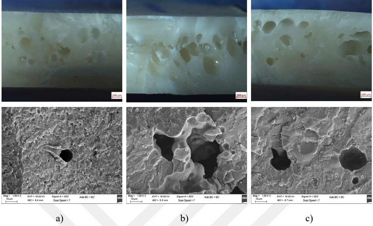
Şekil 3.42 : a) PLA/PA6 (30:70)+%1 KKA, b) PLA/PA6 (30:70)+%1,5 KKA ve c) PLA/PA6 (30:70)+%2 KKA karışımlarının stereo mikroskop ve SEM görüntüleri.
