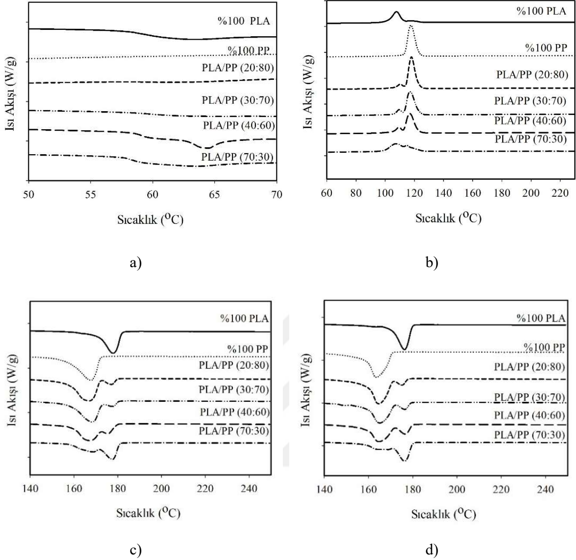
Şekil 3.6 : PLA/PP karışımlarının a) camı geçiş, b) kristalizasyon, c) birinci erime ve d) ikinci erime geçişlerine ilişkin DSC termogramları.
