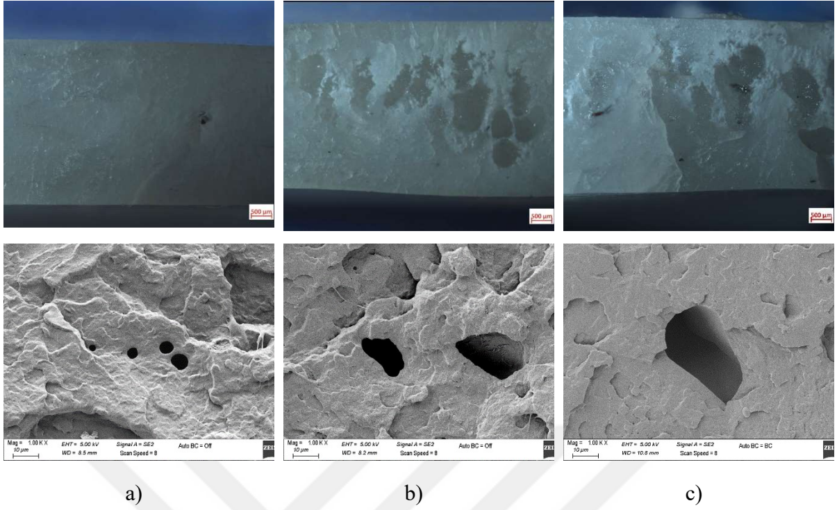
Şekil 3.38 : a) PP+%1 KKA, b) PP+%1,5 KKA ve c) PP+%2 KKA karışımlarının stereo mikroskop ve SEM görüntüleri.
