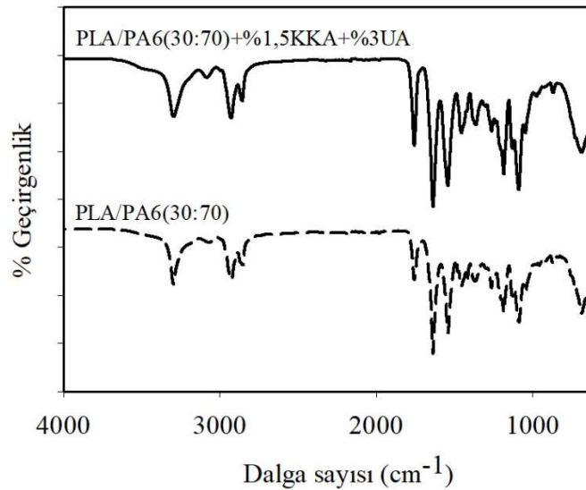
Şekil 3.64 : PLA/PA6 (30:70) ve köpürtücü ile uyumlaştırıcı ajan katkılı PLA/PA6 (30:70) karışımlarının FT-IR spektrumları.
