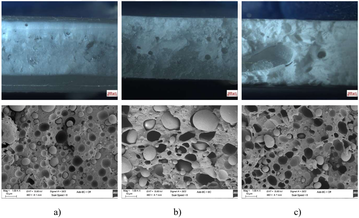
Şekil 3.39 : a) PLA/PP (30:70)+%1 KKA, b) PLA/PP (30:70)+%1,5 KKA ve c) PLA/PP (30:70)+%2 KKA karışımlarının stereo mikroskop ve SEM görüntüleri.
