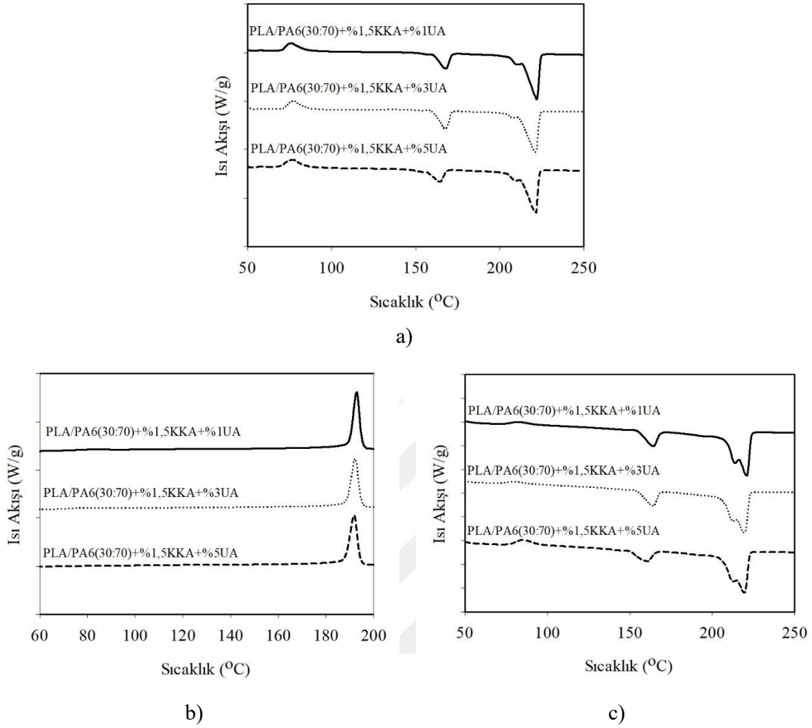
Şekil 3.56 : Farklı oranlarda UA içeren KKA katkılı PLA/PA6 karışımlarının, a) birinci ısıtma, b) soğutma ve c) ikinci ısıtma geçişlerine ilişkin DSC termogramları.
