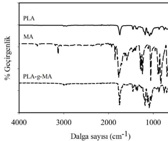
Şekil 2.10 : PLA, MA ve PLA-g-MA'ye ilişkin FT-IR spektrumları.
