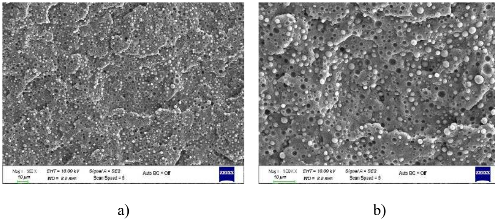
Şekil 3.10 : PLA/PP (20:80) polimer karışımının a) \times 500 ve b) \times 1000 büyütme oranlarında elde edilen SEM görüntüleri.
