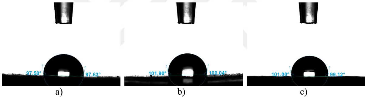
Şekil 3.61 : Farklı oranlarda UA katkılı köpürtülmüş PLA/PP + %1,5 KKA karışımlarının temas açısı ölçüm görüntüleri: a) %1 b) %3 ve c) %5.
