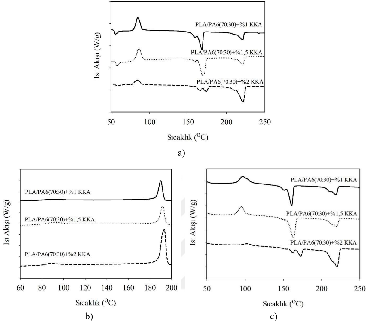
Şekil 3.33 : Farklı oranlarda KKA içeren PLA/PA6 (70:30) karışımlarının, a) birinci ısıtma, b) soğutma ve c) ikinci ısıtma geçişlerine ilişkin DSC termogramları.
