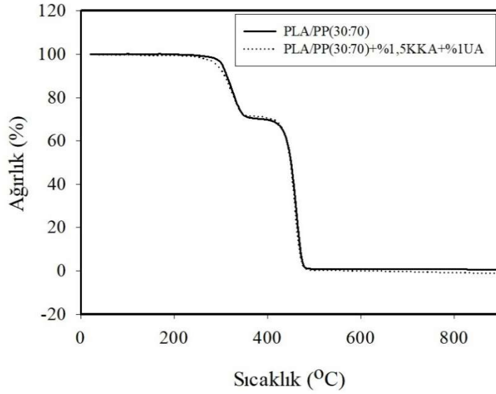
Şekil 3.69 : PLA/PP (30:70) ve köpürtücü ile uyumlaştırıcı ajan katkılı PLA/PP (30:70) karışımlarının TGA termogramları.
