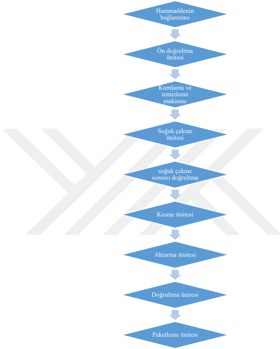
Şekil 4.1. Malzeme akış şeması
