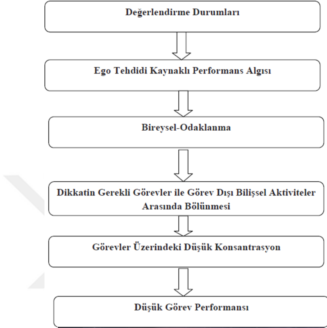
Şekil 3 : Bilişsel-Dikkat Modeli
