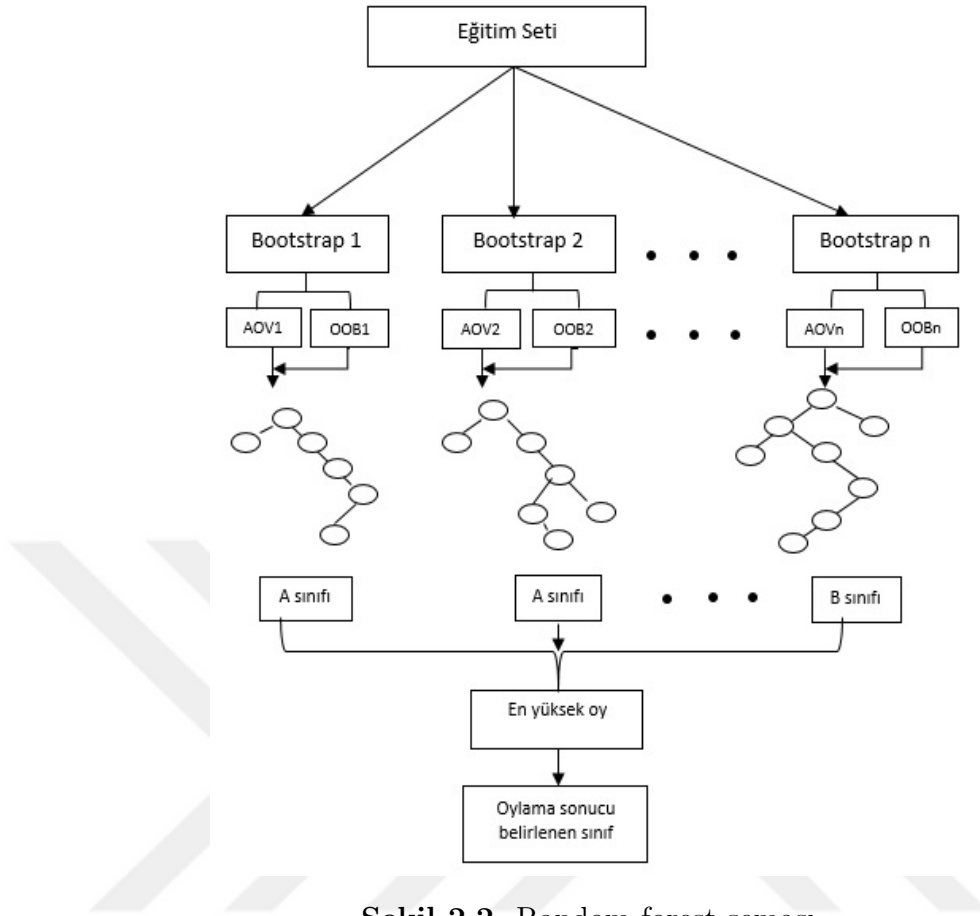
Şekil 2.2. Random forest şeması
