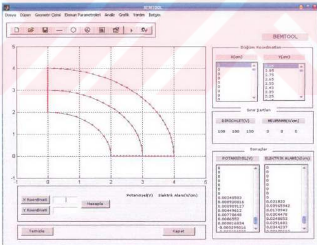
Şekil 6.9 Çeyrek kesitli koaksiyel kablonun analizi
