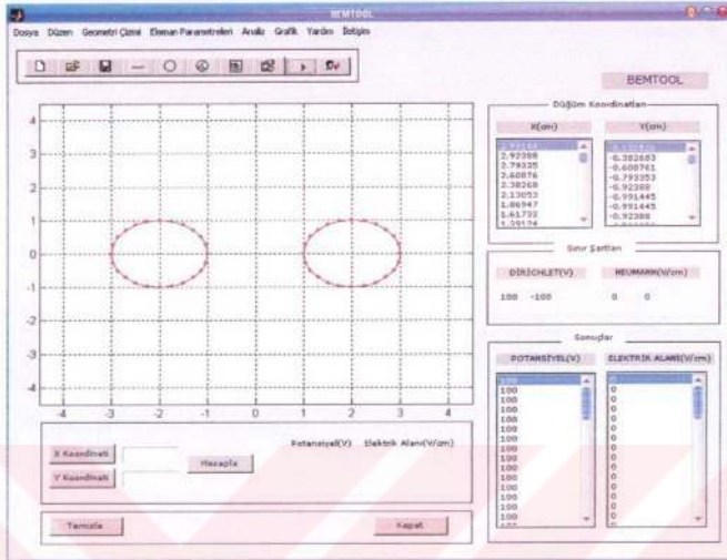
Şekil 6.14 Küre – küre elektrot sisteminin analizi
