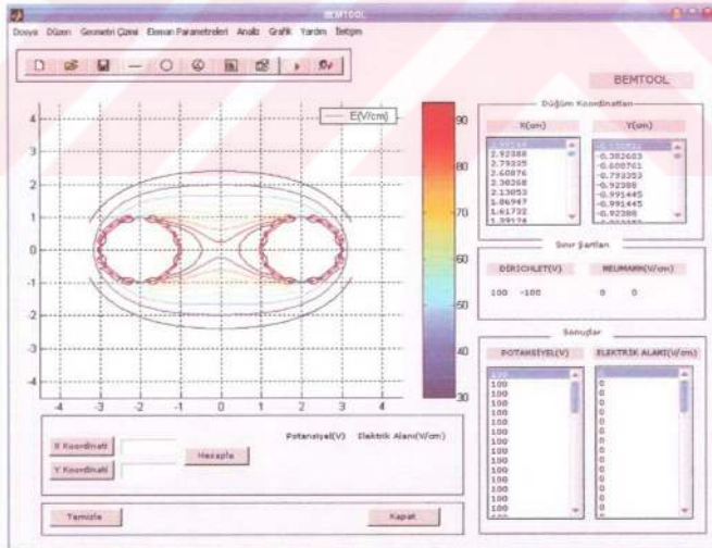
Şekil 6.15 Küre – küre elektrot sisteminin elektrik alanı çizimleri grafiği
