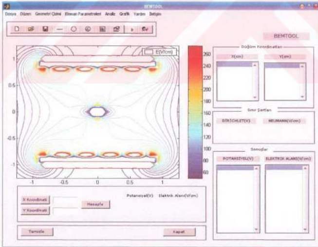
Şekil 6.18 Düzlem-küre-düzlem elektrot sisteminin elektrik alanı çizimleri grafiği
