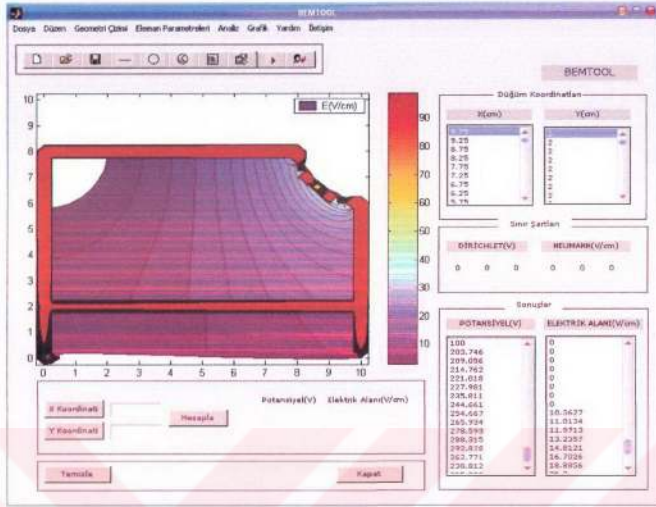
Şekil 6.8 Silindir – Düzlem elektrot sisteminin dolgu elektrik alanı çizgileri grafiği
