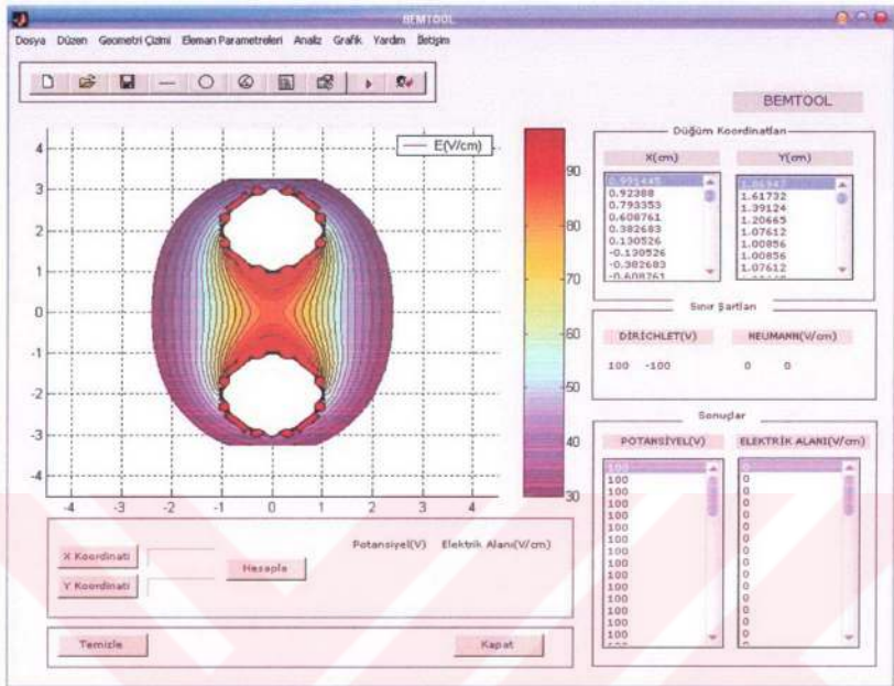
Şekil 5.25 Küre-küre elektrot modelinin dolgu elektrik alanı çizgileri grafiği
