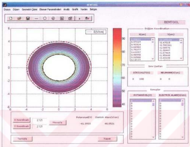
Şekil 6.3 Koaksiyel kablunun dolgu elektrik alanı çizgilere grafiği
