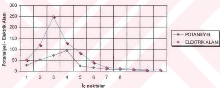
Şekil 6.11 İç noktalarındaki potansiyel ve elektrik alanı dağılımı
