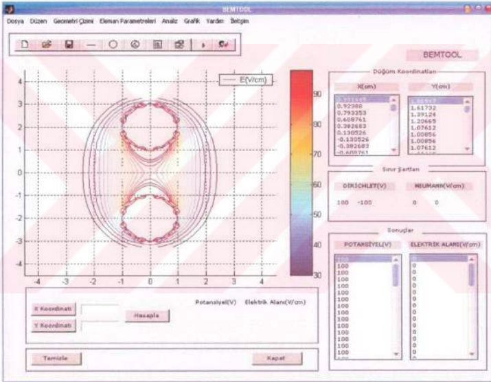
Şekil 5.24 Küre-küre elektrot modelinin elektrik alanı çizgileri grafiği
