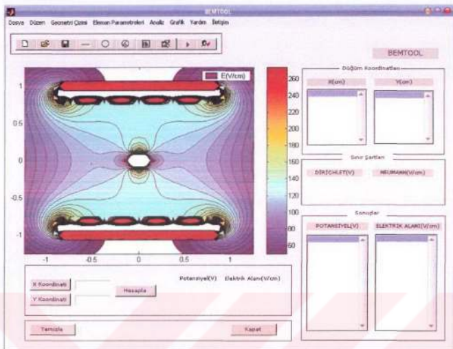
Şekil 6.18 Düzlem-küre-düzlem elektrot sisteminin dolgulu elektrik alanı çizimleri grafiği
