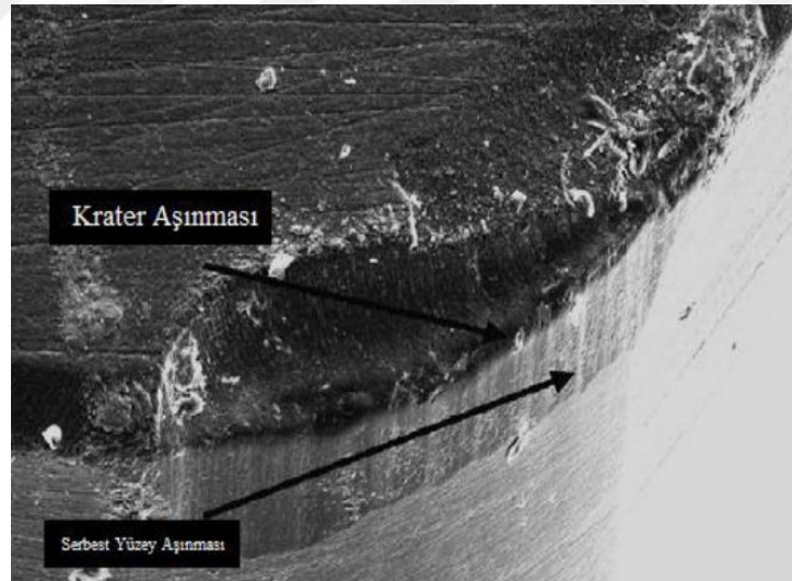
Şekil 4.15. Krater aşınması [75]
