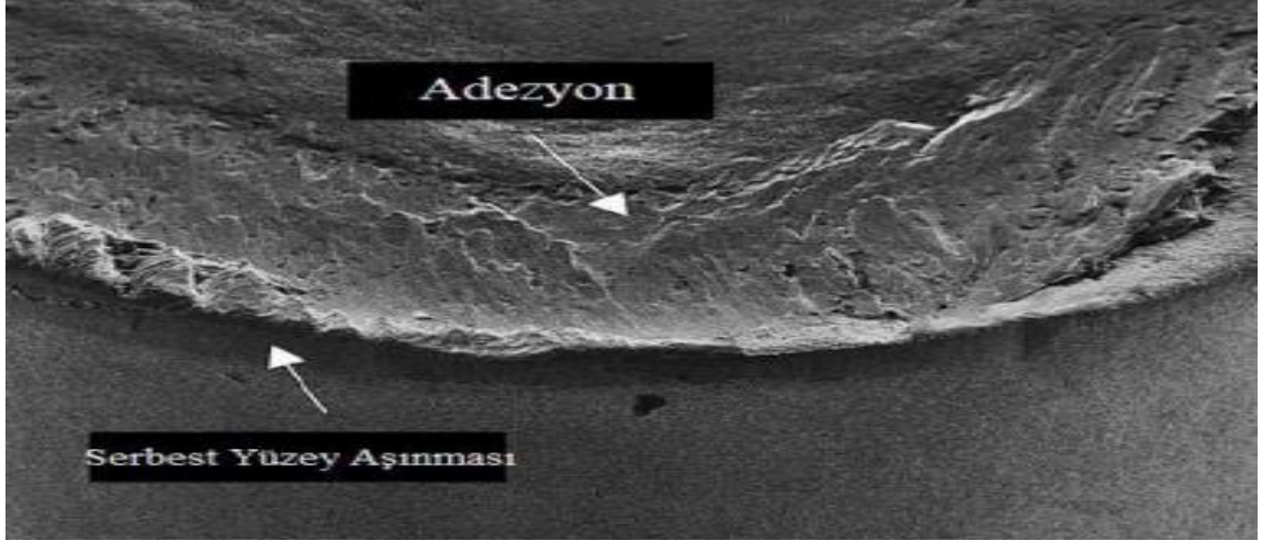
Şekil 4.24. Adhezif aşınma [75]
