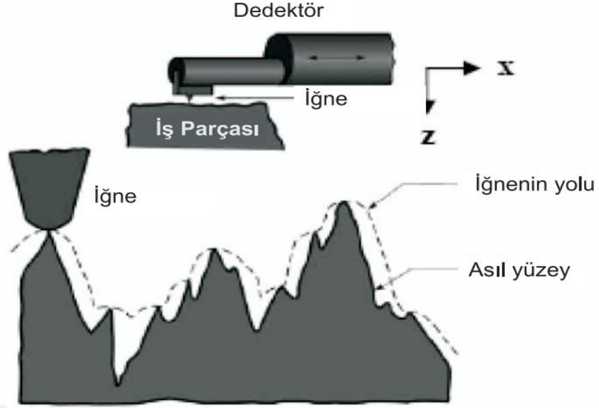
Şekil 4.27. Temas uçlu ölçme yöntemi [47]
