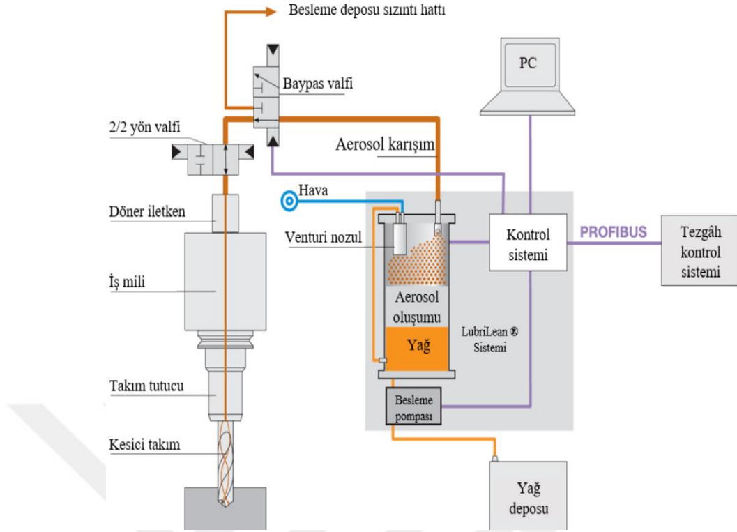
Şekil 5.6. Kesici takımın içinden uygulanan minimum miktarda yağlama yöntemi [65]
