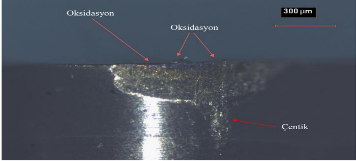
Şekil 4.25. Oksidasyon aşınması [40]
