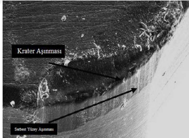
Şekil 4.15. Krater aşınması [75]
