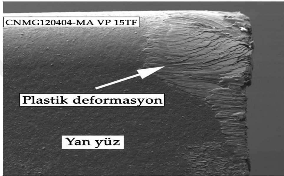
Şekil 4.20. Plastik deformasyon [38]
