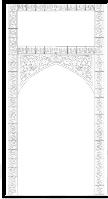
Şekil 33 Kaymakam Sait Bey Çeşmesi Kuzey Yönü Karo Planı Kenar Karo Restitüsyon Çizim Çalışması (Burak ÜNER-22.05.2020-Bursa-TÜRKİYE)
