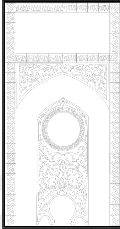
Şekil 9 Kaymakam Sait Bey Çeşmesi Kuzey Yönü Karo Planı Restitüsyon Çizim Çalışması (Burak ÜNER-22.05.2020-Bursa-TÜRKİYE)
