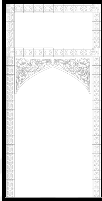
Şekil 158 Kaymakam Sait Bey Çeşmesi Doğu Yönü Kenar Karo Restitüsyon Çizim Çalışması (Burak ÜNER-22.05.2020-Bursa-TÜRKİYE)
