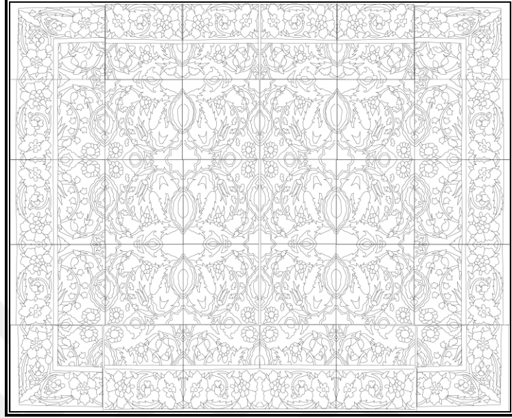
Şekil 223 Hamidiye Camii Doğu Yönünde Bulunan Çinilerin Restitüsyon Çizimi (Burak ÜNER-02.06.2020-Bursa-TÜRKİYE)
