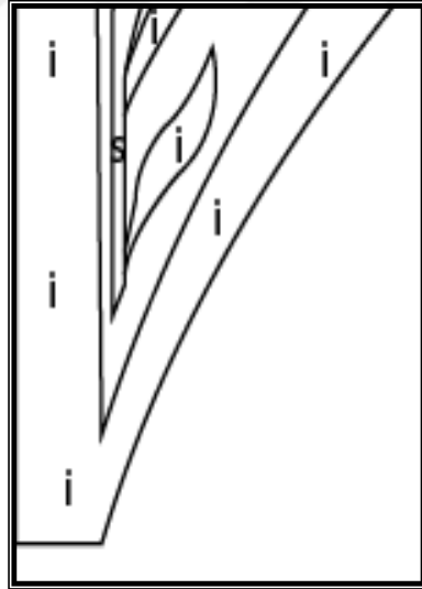
Resim 135 ,Şekil 180 Kaymakam Sait Bey Çeşmesi Doğu Yönü 53. Karo Restitüsyon Çizim Çalışması (Burak ÜNER-22.05.2020-Bursa-TÜRKİYE)
