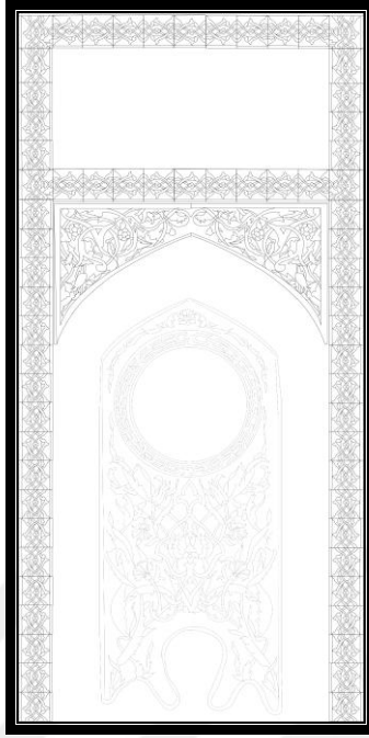
Şekil 89 Kaymakam Sait Bey Çeşmesi Batı Yönü Karo Planı Restitüsyon Çizim Çalışması (Burak ÜNER-22.05.2020-Bursa-TÜRKİYE)
