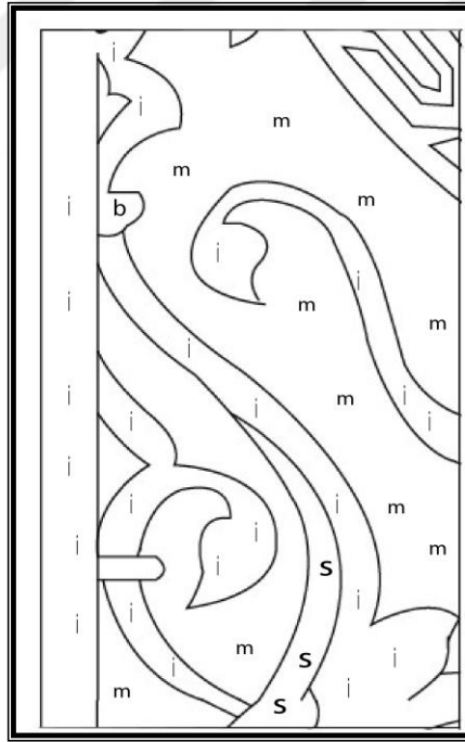
Resim 60, Şekil 13 Kaymakam Sait Bey Çeşmesi Kuzey Yönü 85.Karo Detay Fotoğrafı ve Restitüsyon Çizim Çalışması (Burak ÜNER-22.05.2020-Bursa-TÜRKİYE)
