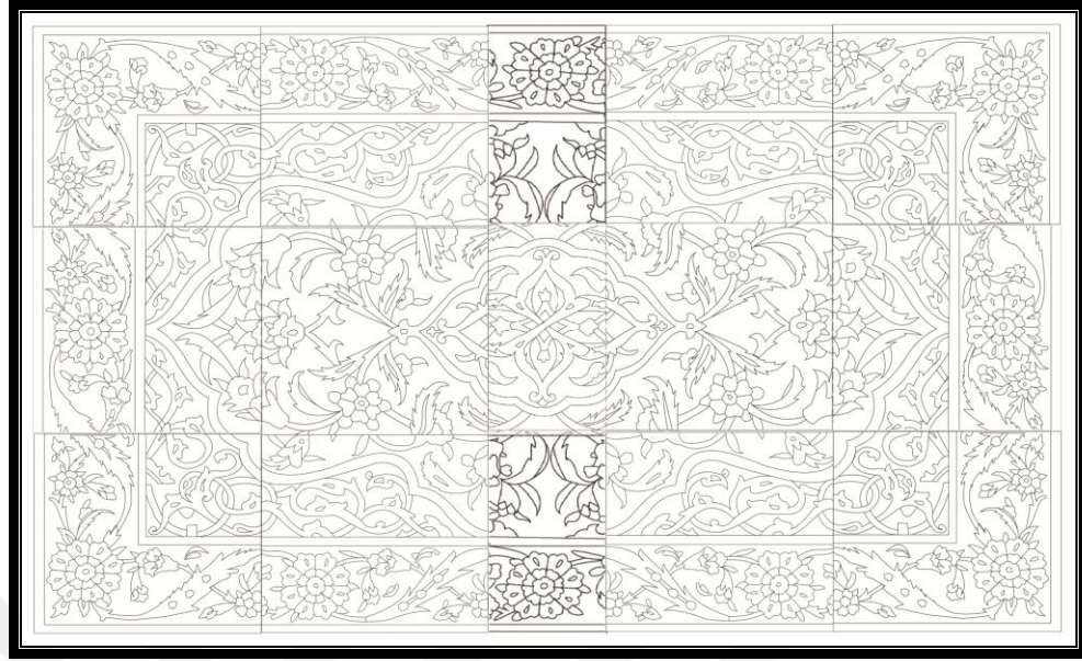
Şekil 203 Dar'ul Eytam Giriş Kapısı Üzerinde Sağ ve Sol Tarafında Bulunan Pano Karo Planı Restitüsyon Çalışması (Burak ÜNER-22.02.2020-Bursa-TÜRKİYE)
