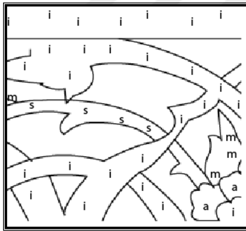
Resim 108, Şekil 121 Kaymakam Sait Bey Çeşmesi Batı Yönü 31.Karo Detay Fotoğrafi Restitüsyon Çizim Çalışması (Burak ÜNER-22.05.2020-Bursa-TÜRKİYE)
