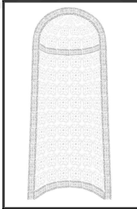
Şekil 2 Ertuğrul Gazi Türbesi Mihrap Röleve Çizimi (Burak ÜNER-22.05.2020 Bursa-TÜRKİYE)
