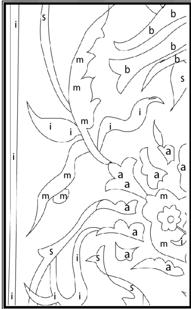
Resim 120, Şekil 148 Kaymakam Sait Bey Çeşmesi Doğu Yönü 89. Karo ve Restitüsyon Çizim Çalışması (Burak ÜNER-22.05.2020-Bursa-TÜRKİYE)
