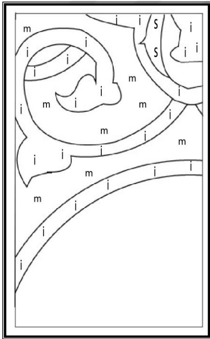
Resim 65 Şekil 23 Kaymakam Sait Bey Çeşmesi Kuzey Yönü 95.Karo Detay Fotoğrafi ve Restitüsyon Çizim Çalışması (Burak ÜNER-22.05.2020-Bursa-TÜRKİYE)
