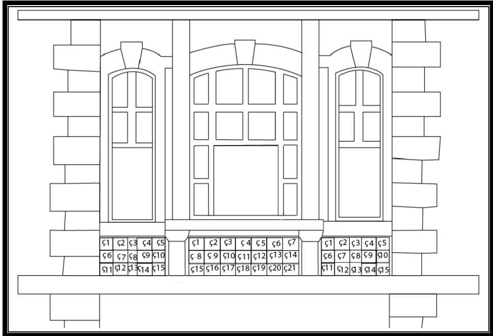
Şekil 182 Dar'ul Eytam Giriş Kapısı Üzerinde Bulunan Pano Karo Plan Çalışması (Burak ÜNER-22.02.2020-Bursa-TÜRKİYE)
