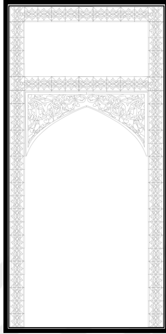
Şekil 109 Kaymakam Sait Bey Çeşmesi Batı Yönü Karo Planı Kenar Karo Restitüsyon Çizim Çalışması (Burak ÜNER-22.05.2020-Bursa-TÜRKİYE)
