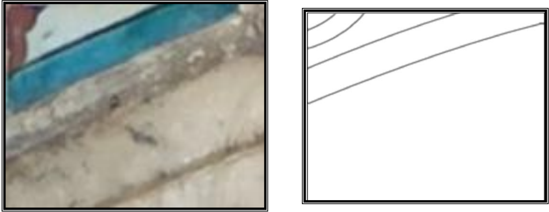
Resim 79 Şekil 52 Kaymakam Sait Bey Çeşmesi Kuzey Yönü 43. Karo Detay Fotoğrafı ve Restitüsyon Çizim Çalışması (Burak ÜNER-22.05.2020-Bursa-TÜRKİYE)
