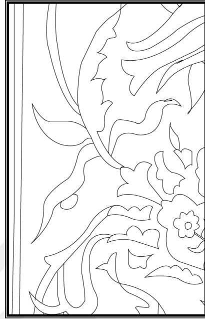
Resim 120, Şekil 148 Kaymakam Sait Bey Çeşmesi Doğu Yönü 89. Karo ve Restitüsyon Çizim Çalışması (Burak ÜNER-22.05.2020-Bursa-TÜRKİYE)
