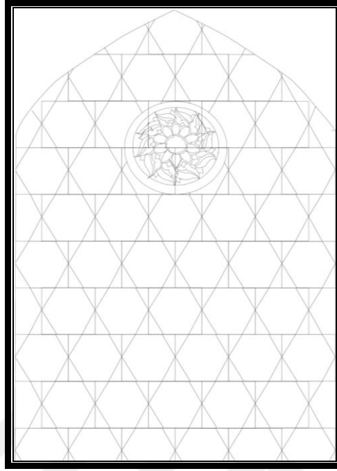
Şekil 61 Kaymakam Sait Bey Çeşmesi Güney Yönü Karo Planı Orta Karo Restitüsyon Çizim Çalışması (Burak ÜNER-22.05.2020-Bursa-TÜRKİYE)
