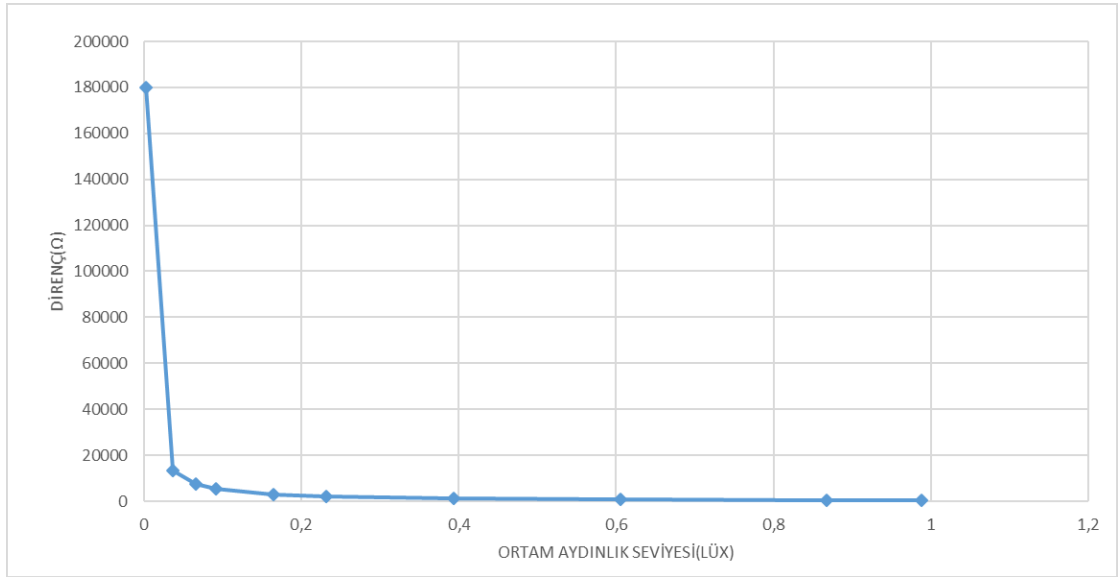
řekil 6.13. Ortam aydınlık seviyesi, diren deęiřim grafięi.
