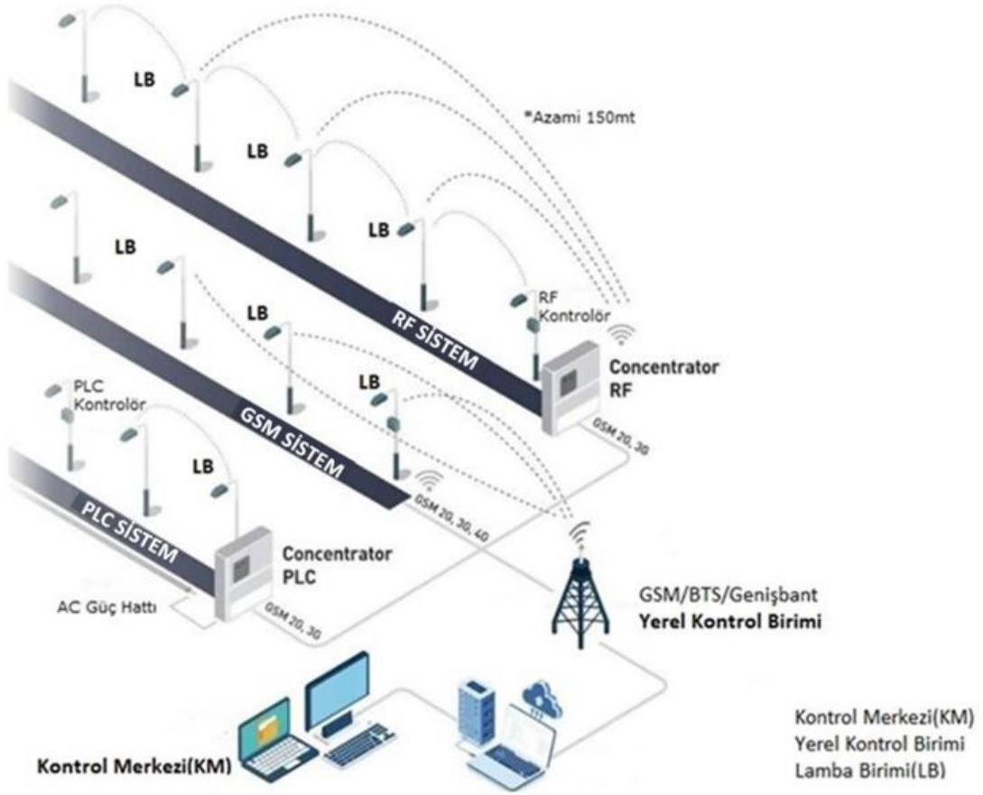
Şekil 5.2. Hibrit haberleşme sistemi.
