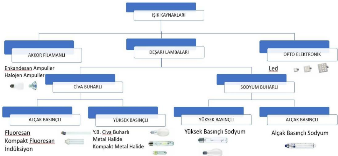
Şekil 2.1. Işık kaynakları.
