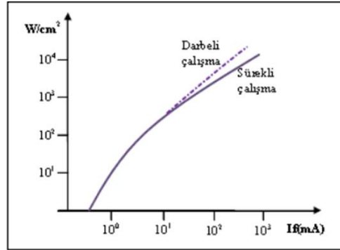
Şekil 3.8. Led'in akım-ışık karakteristiği (Göçmen, 2014).
