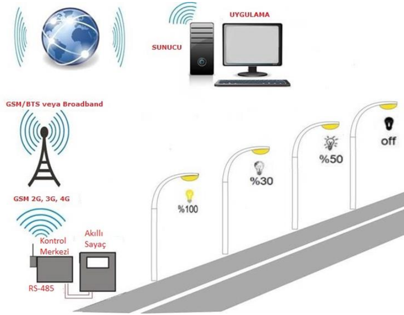
Şekil 6.1. LASAS sistem mimarisi.
