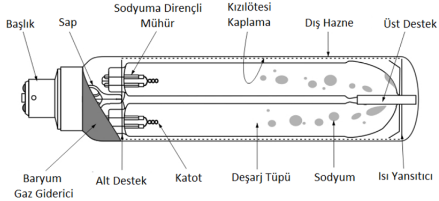
Şekil 3.4. Alçak basınçlı sodyum buharlı lambanın yapısı (Kaya, 2018).
