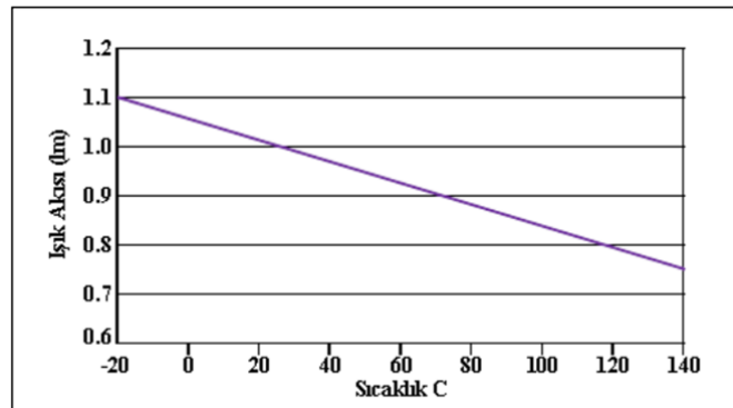
Şekil 3.9. Led'in sıcaklık ışık akısı değişim grafiği (Göçmen, 2014).
