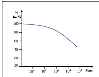
Şekil 3.7. Led'in verim-zaman karakteristiği (Göçmen, 2014).
