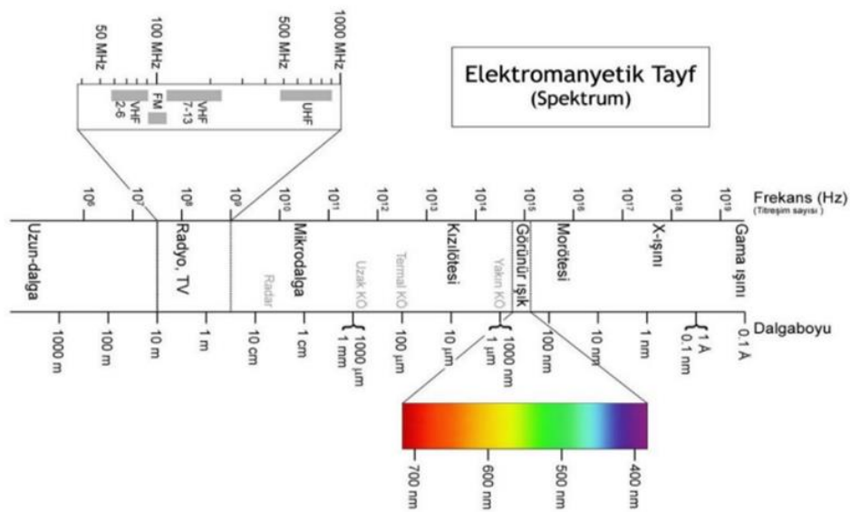
Şekil 2.2. Elektromanyetik dalga ve görünür ışık tayfı (Demir, 2020).
