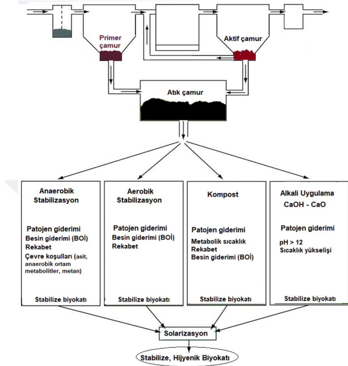
Şekil 2.2. Arıtma tesislerinde arıtma çamurunun ortaya çıkışı, stabilizasyonu ve bu çalışmada önerilen ileri patojen giderimi yöntemi; solarizasyon.
