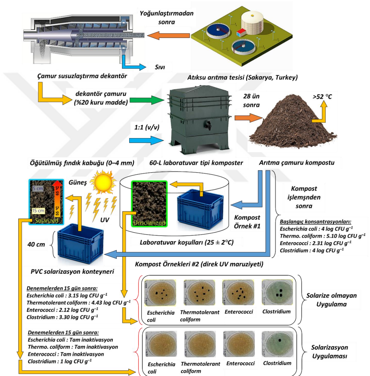
Şekil 3.1. Mikrobiyal dezenfeksiyon için çamur kompostuna yapılan güneş enerjisi uygulamalarının şematik gösterimi.
