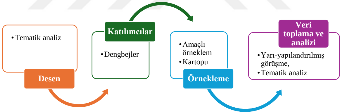
Şekil 3.2. Araştırma süreci
