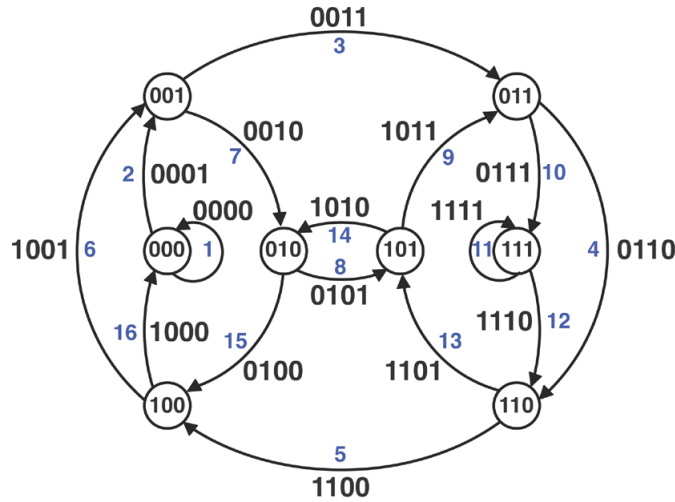
Şekil 2.6. 2 harfli \Sigma = \{0, 1\} alfabesi üzerinde 3 boyutlu De Bruijn çizgesi (Compeau vd. 2011).
