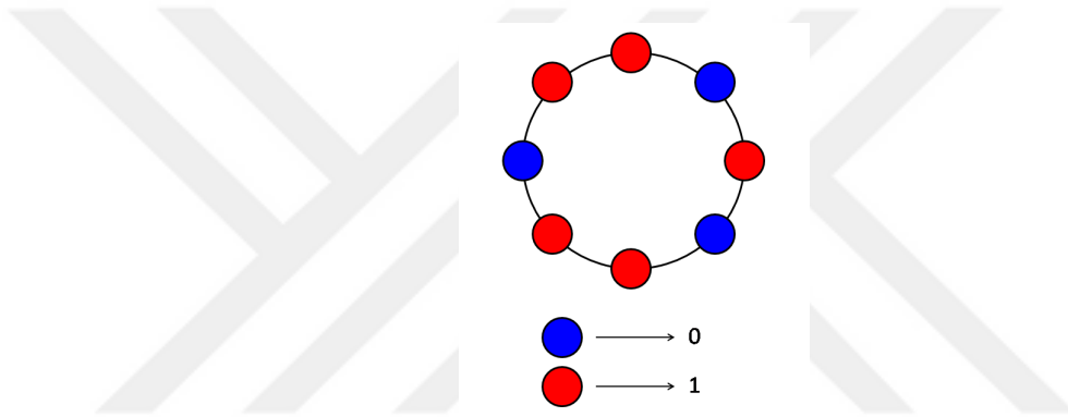
Şekil 2.1. k = 2 ve n = 8 için bir kombinatoriksel kolye
