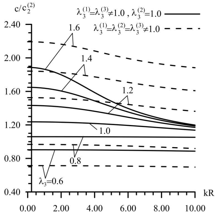
Şekil 3. 28 \mu^{(1)} / \mu^{(2)} = 2 , h^{(1)} / R = h^{(3)} / R = 0.2 , h^{(2)} / R = 0.4 koşulları altında, silindir katmanlarındaki ön şekil değiştirmelerin 1. mod dispersiyon eğrilerine etkisi
