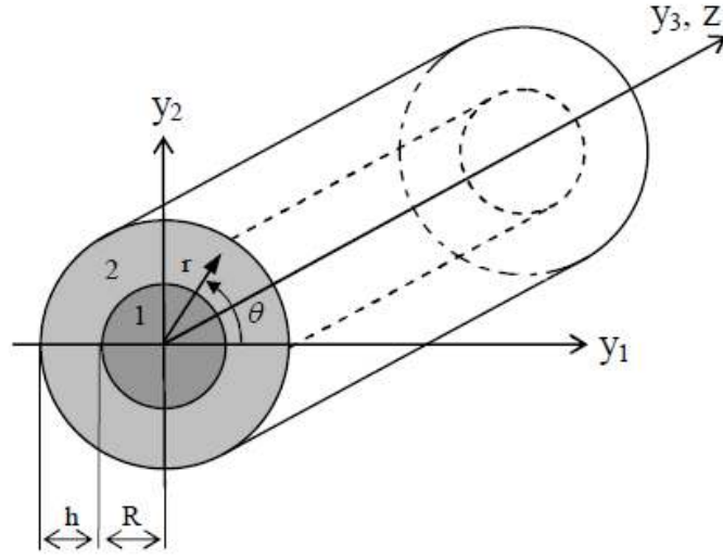
Şekil 2. 1 Bileşik silindir
