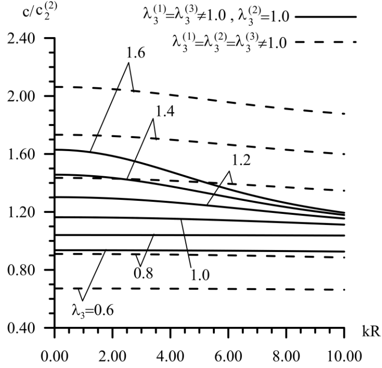
Şekil 3. 26 \mu^{(1)}/\mu^{(2)} = 2 , h^{(1)}/R = h^{(3)}/R = 0.1 , h^{(2)}/R = 0.4 koşulları altında, silindirik katmanlarındaki ön şekil değiştirmelerin 1. mod dispersiyon eğrilerine etkisi
