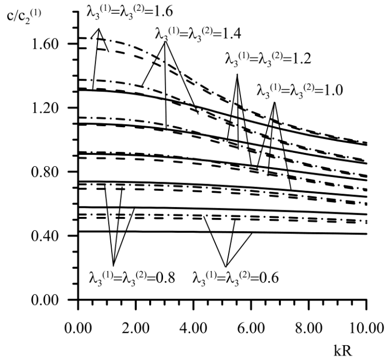
Şekil 2. 18 Farklı h^{(1)} / R değerleri için öngerilmelerin dispersiyon eğrileri üzerindeki etkisi \mu^{(1)} / \mu^{(2)} = 5 , h^{(2)} / R = 0.1 ; — h^{(1)} / R = 0.1 ; - - h^{(1)} / R = 0.5 ; - . - h^{(1)} / R = 1.0
