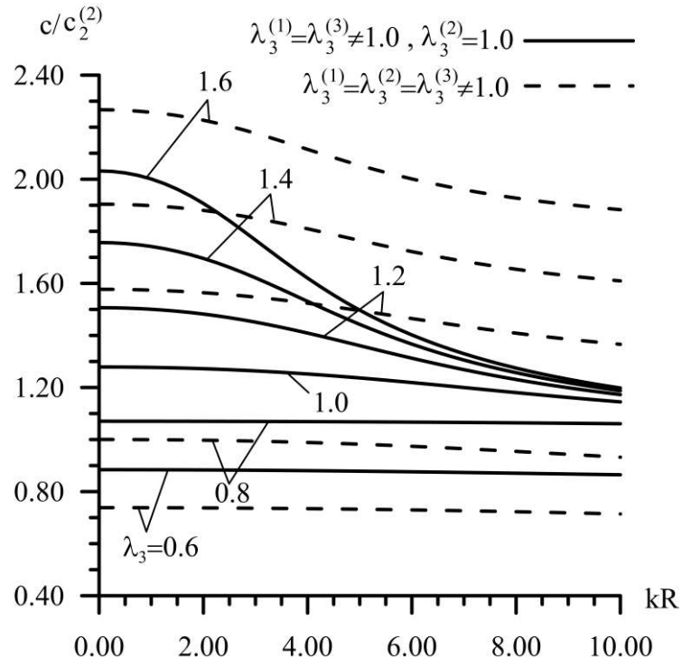
Şekil 3. 29 \mu^{(1)} / \mu^{(2)} = 2 , h^{(1)} / R = h^{(3)} / R = 0.3 , h^{(2)} / R = 0.4 koşulları altında, silindir katmanlarındaki ön şekil değiştirmelerin 1. mod dispersiyon eğrilerine etkisi
