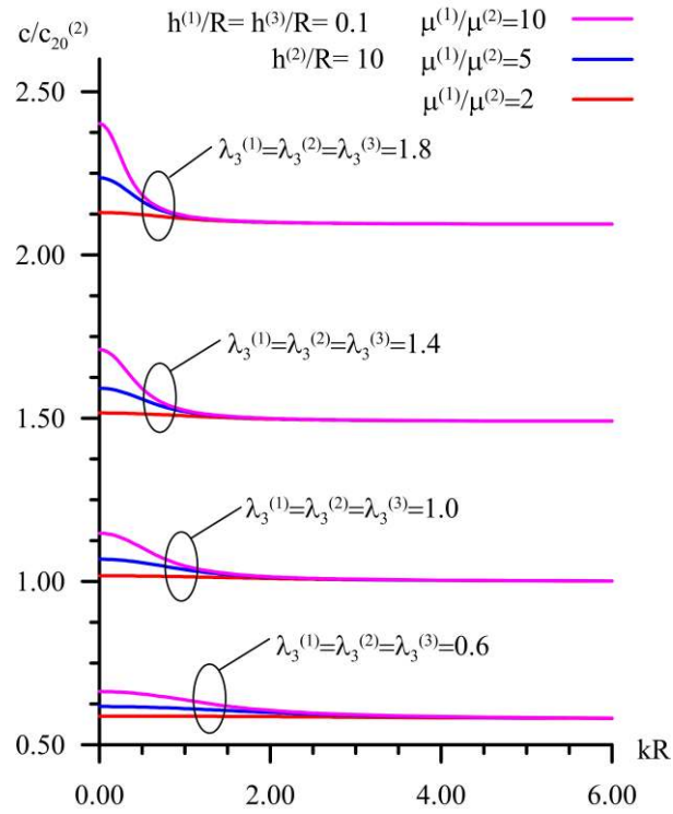
Şekil 3. 18 Ön şekil değiştirmelerin çeşitli \mu^{(1)}/\mu^{(2)} değerleri için h^{(2)}/R=10 koşulu altında, burulma dalgı yayılım hızına etkisi
