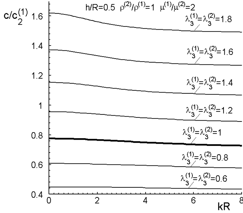
Şekil 2. 10 1. modda, öngerilmelerin dispersiyon eğrileri üzerindeki etkisi ( \mu^{(1)}/\mu^{(2)} = 2 )
