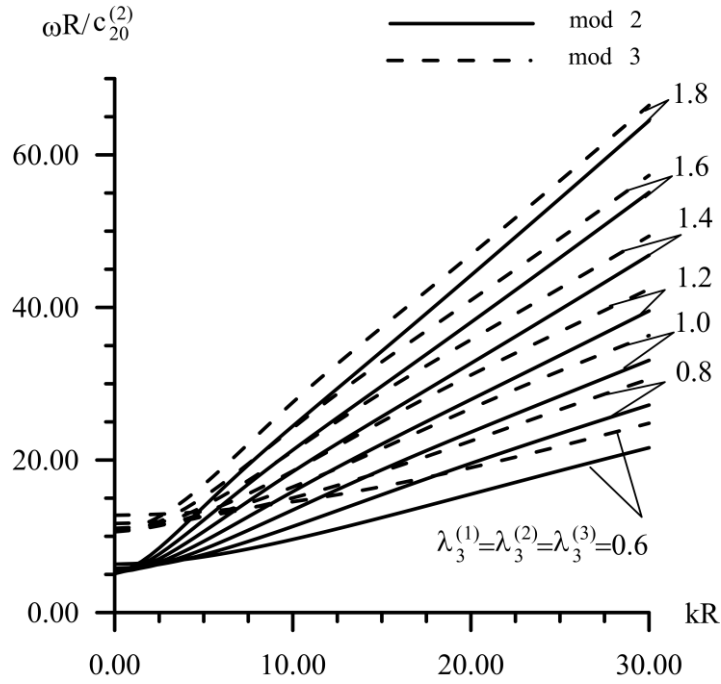
Şekil 3. 25 \mu^{(2)}/\mu^{(1)}=\mu^{(2)}/\mu^{(3)}=0.5 durumunda ve h^{(1)}/R=h^{(3)}/R=0.1 , h^{(2)}/R=0.4 koşulları altında, silindir katmanlarındaki ön şekil değiştirmelerin 2. ve 3. modların dispersiyon eğrilerine etkisi
