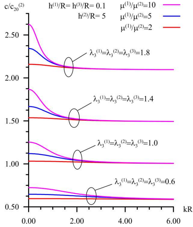
Şekil 3. 17 Ön şekil değiştirmelerin çeşitli \mu^{(1)}/\mu^{(2)} değerleri için h^{(2)}/R=5 koşulu altında, burulma dalgı yayılım hızına etkisi
