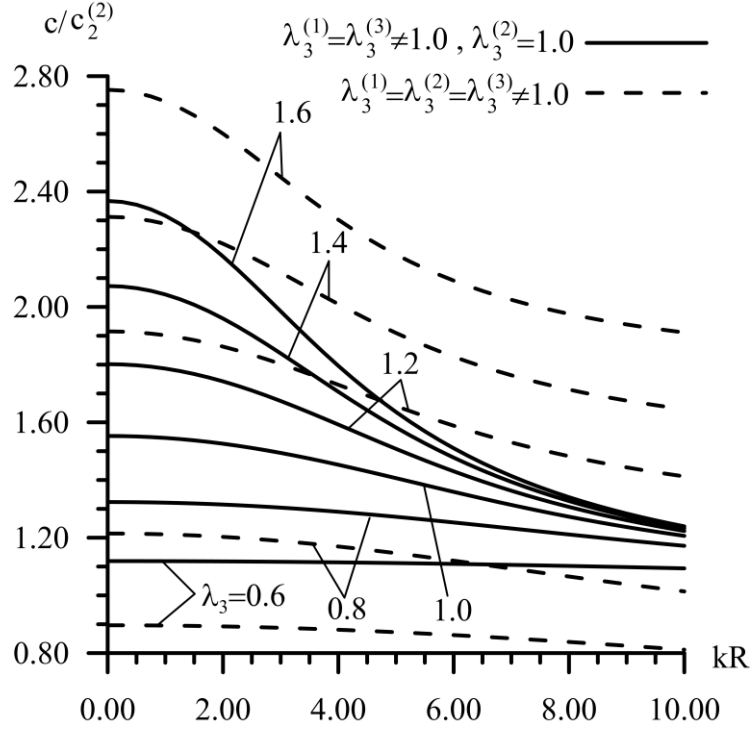
Şekil 3. 27 \mu^{(1)}/\mu^{(2)} = 5 , h^{(1)}/R = h^{(3)}/R = 0.1 , h^{(2)}/R = 0.4 koşulları altında, silindirik katmanlarındaki ön şekil değiştirmelerin 1. mod dispersiyon eğrilerine etkisi
