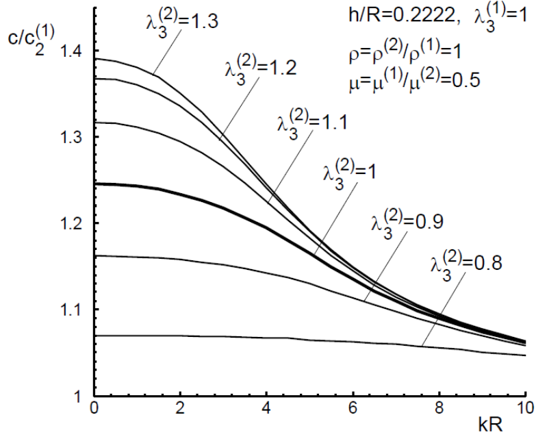
Şekil 2. 4 1. mod için [8] göz önüne alınarak oluşturulan dispersiyon eğrileri (hız, dalga sayısı ilişkisi)
