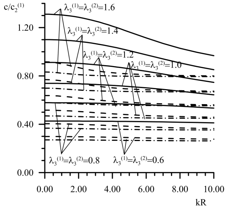
Şekil 2. 17 Farklı h^{(2)}/R değerleri için öngerilmelerin dispersiyon eğrileri üzerindeki etkisi \mu^{(1)}/\mu^{(2)} = 5 , h^{(1)}/R = 0.1 ; — h^{(2)}/R = 0.1 ; - - - h^{(2)}/R = 0.5 ; - . - . h^{(2)}/R = 1.0
