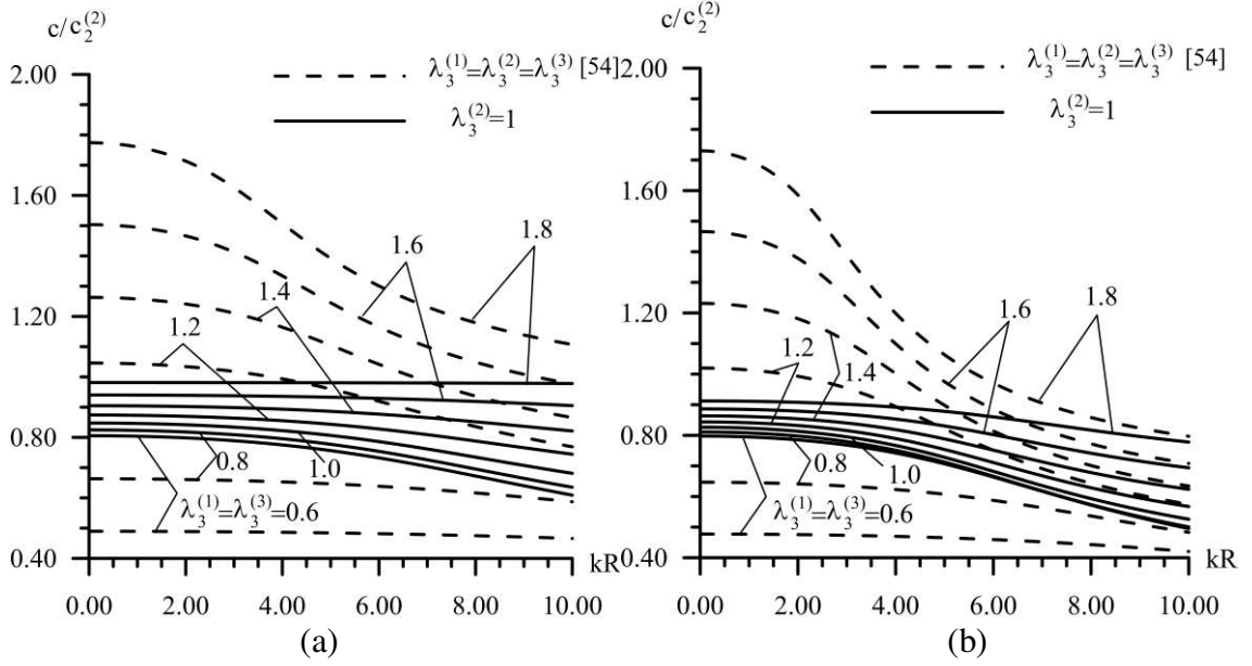
Şekil 3. 14 1. mod ve \mu^{(2)}/\mu^{(1)} = \mu^{(2)}/\mu^{(3)} = 5 (a) ve 10 (b), h^{(1)}/R = h^{(3)}/R = 0.1 , h^{(2)}/R = 0.4 koşulları altında oluşturulmuş dispersiyon eğrileri
