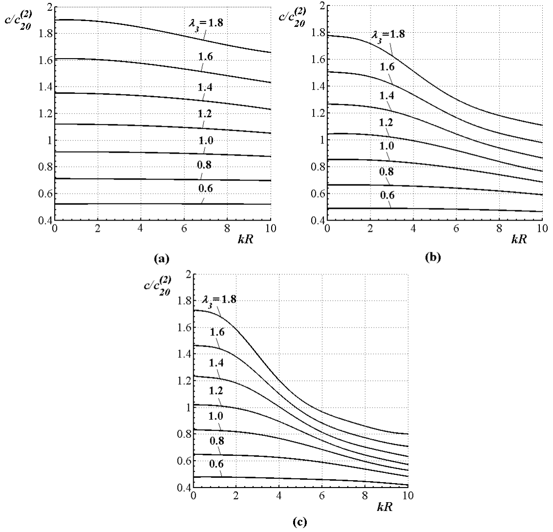
Şekil 3.4 1. mod ve (\mu^{(2)}/\mu^{(1)}) = (\mu^{(2)}/\mu^{(3)}) = 2(a), 5(b), 10(c) , h^{(2)}/R = 0.4 , h^{(1)}/R = h^{(3)}/R = 0.1 koşulları altında, ön şekil değiştirmelerin dispersiyon eğrilerine etkisi.
