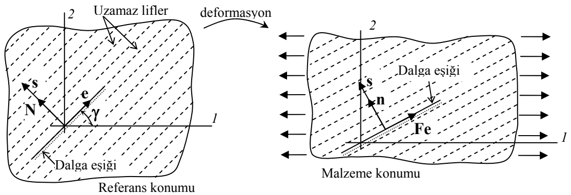
Şekil 5.9. Uzamaz liflerle kuvvetlendirilmiş olan cisimde boyuna şok dalgası yayılımı
