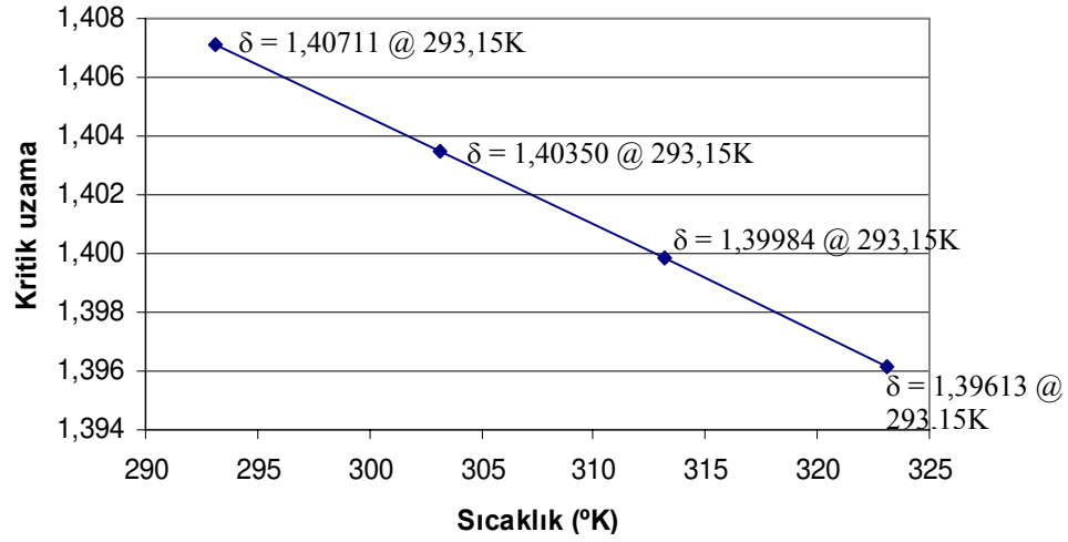
Şekil 5.12. Kayma bandı oluşturacak kritik uzama değerleri ( \gamma = \pi/4 )
