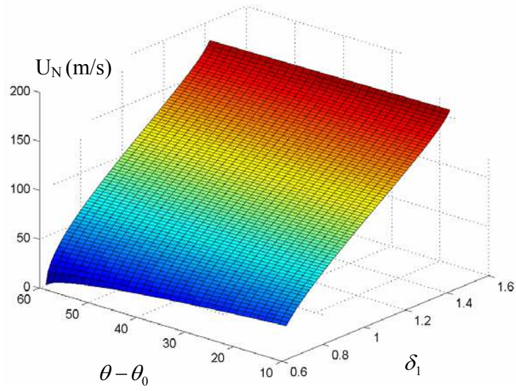
Şekil 4.23. \gamma = \pi/4 için boyuna zayıf şok dalgası hızının l -eksenindeki uzama ve sıcaklık artımıyla değişimi ( \beta = \gamma + \pi/2 )
