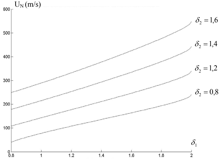
Şekil 4.32. \gamma = \pi/3 için boyuna zayıf şok dalgası hızının I -eksenindeki uzama ve sıcaklık artımıyla değişimi, (\beta = \gamma + \pi/2) ve \theta - \theta_0 = 10^\circ K
