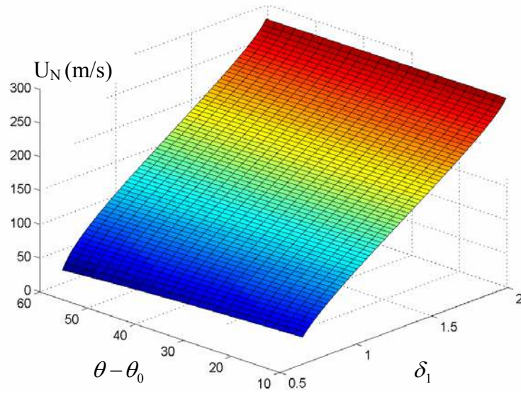
Şekil 4.24. \gamma = \pi/3 için boyuna zayıf şok dalgası hızının l -eksenindeki uzama ve sıcaklık artımıyla değişimi ( \beta = \gamma + \pi/2 )
