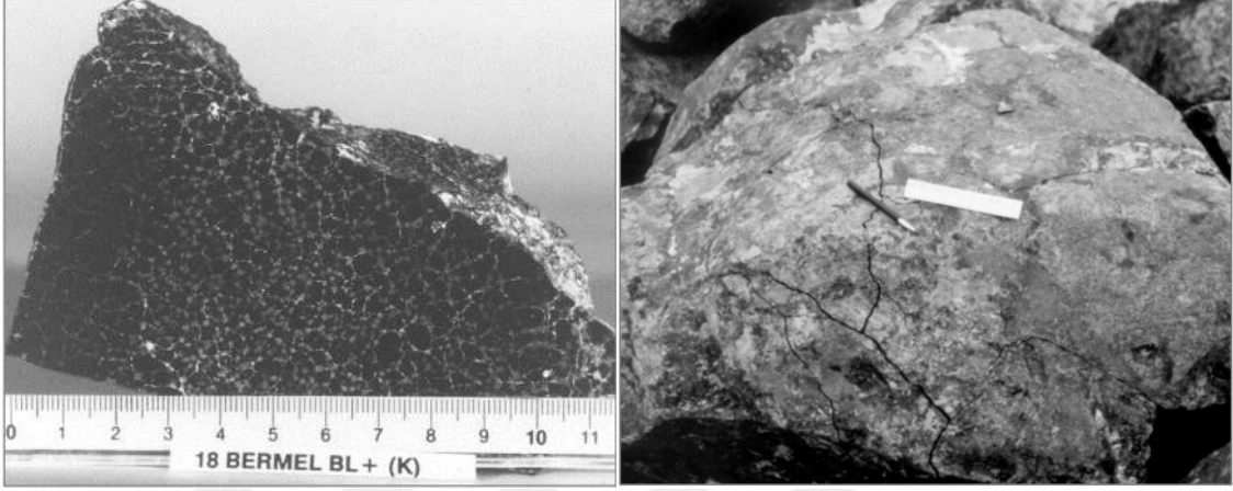
Şekil 1.1. Sonnenbrand etkisi ile basalt kayaçlarında yıldız şekilli/bir noktadan yayılarak uzayan çatlaklar (Ciria/Cur C683, (2007))
