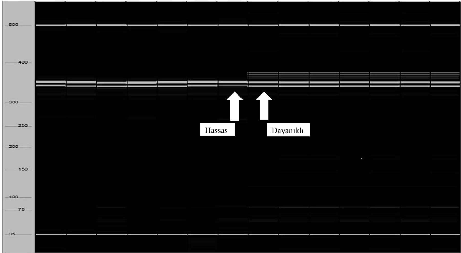
Şekil 4.4. Fragment Analyzer™ ile yapılan analiz sonrasında afıt zararlısına karşı belirlenen dayanıklı ve hassas genotiplere ait kapıları elektroferaz görüntüsü
