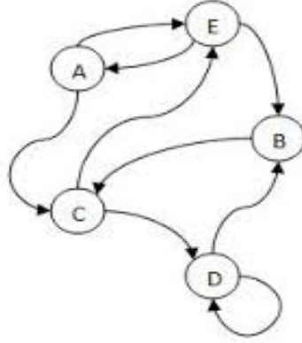
Şekil 4.3 Yönlü graf
