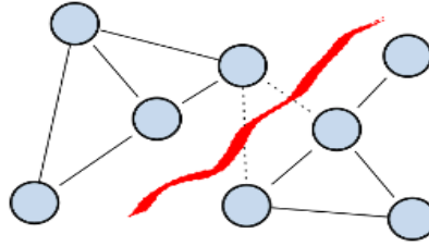
Şekil 5.1 Graf Bölütleme
