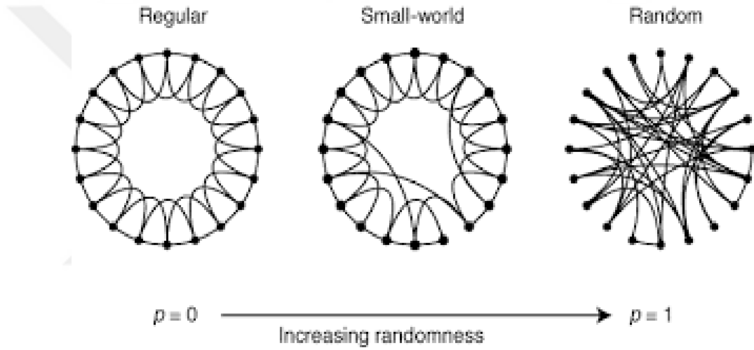
Şekil 3.3. Küçük dünya ağının oluşum süreci [24]
