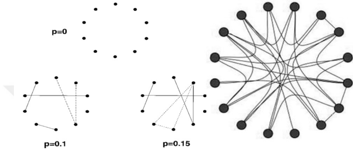
Şekil 3.2. Rassal Ağ'ın oluşum süreci & Rassal Ağ'ın görünümü [22]
