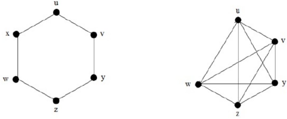
Şekil 2.15. Alt graf örnekleri [9]
