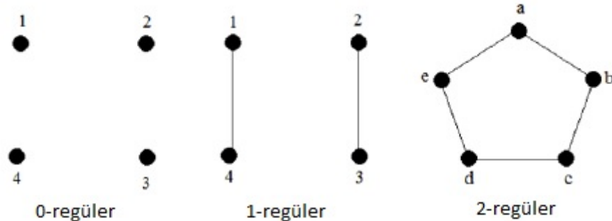
Şekil 2.16. Regüler graflar
