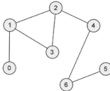
Şekil 4.2 Yönsüz graf
