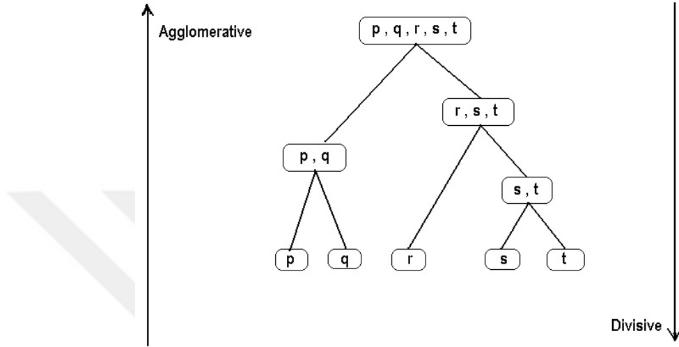
Şekil 5.2 Hiyerarşik Bölütleme
