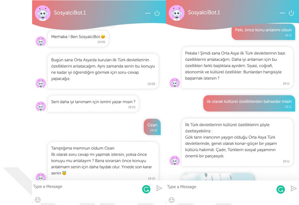
Görsel 2.7. Örnek sohbet akışları.1
