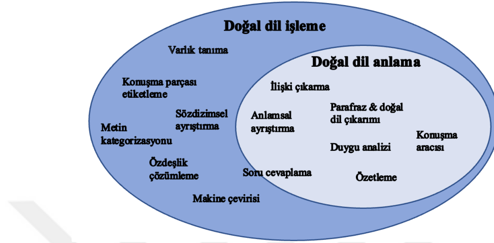
Şekil 2.3. Doğal dil işleme ve doğal dil anlama ilişkisi
