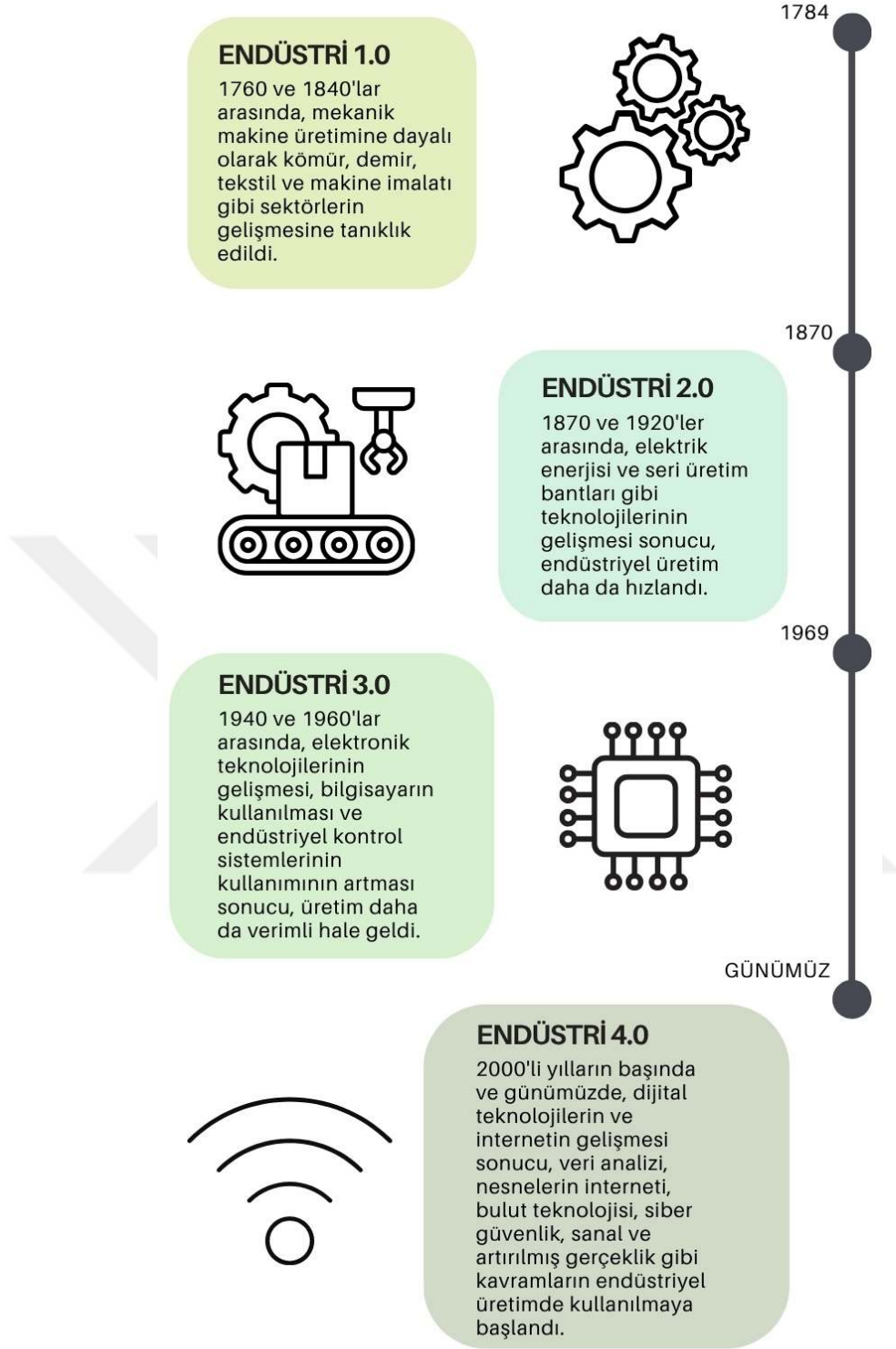
Şekil 2.3: Sanayi Devrimleri.
