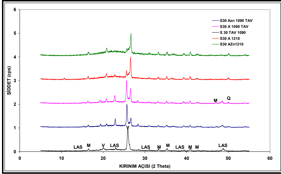
Şekil 3.108. d. 1090 °C de tavllanmış S 30 - S30A-Zn - S30A bünyelerine ait XRD grafiği (Q: kuvars, M: müllit, LAS: lityum alümina silikat)
