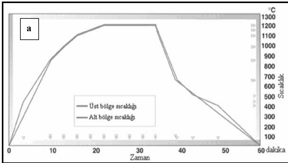
Şekil 1.6.a. Rulolu tünel fırınlarında sıcaklık eğrisinin gösterimi [12]
