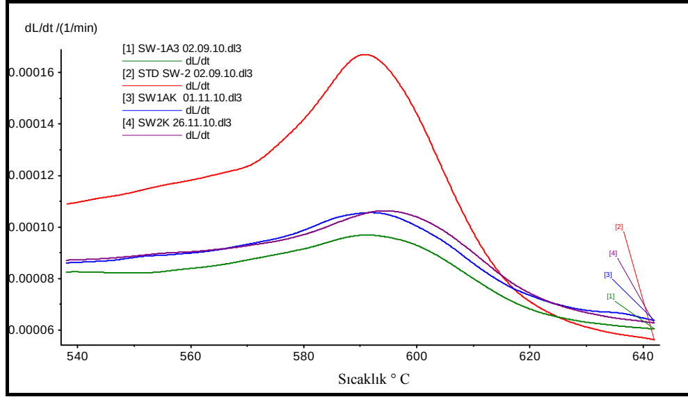
Şekil 3.24. 4. seri numunelere ait kuvars dönüşümünün olduğu sıcaklıklarda ısı genleşme eğrileri
