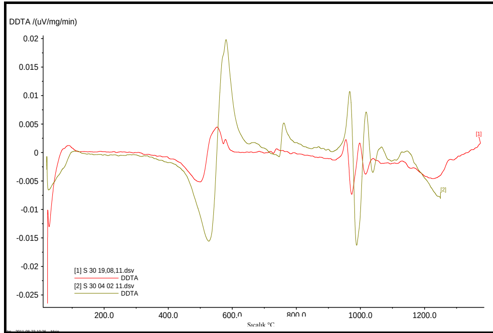
Şekil 3.108.ı. Endüstriyel şartlarda hazırlanmış bünyelerin DDTA eğrileri
