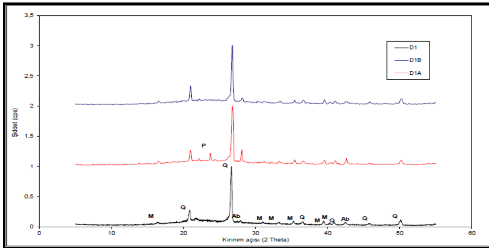
Şekil 3.16. 2. seri numunelere ait XRD grafiği, (M: müllit, Q: kuvars, Ab: albit, P: petalit)
