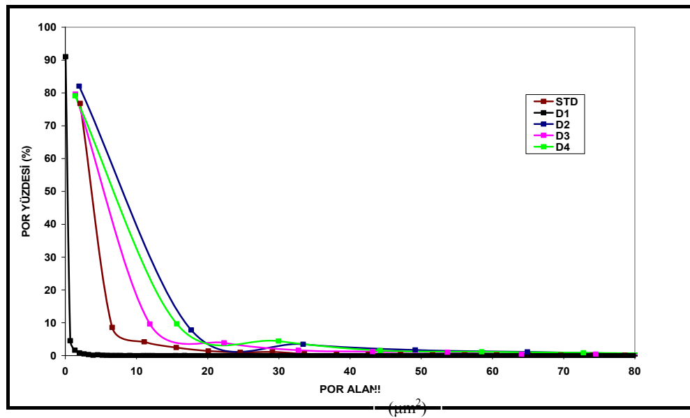
Şekil 3.40. 1.seri numuneler için por alanı- por yüzdesi
