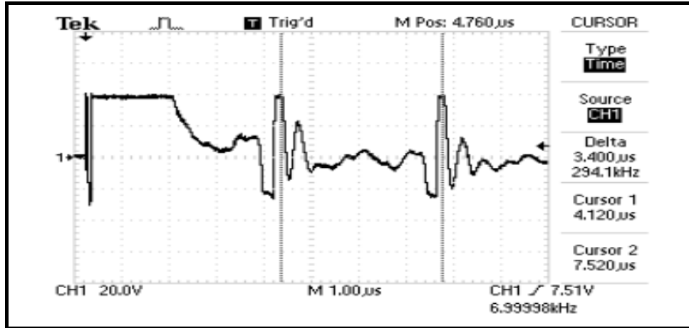
Şekil 3.67.b. MDAK bünyesine ait enine ses hızı grafiği
