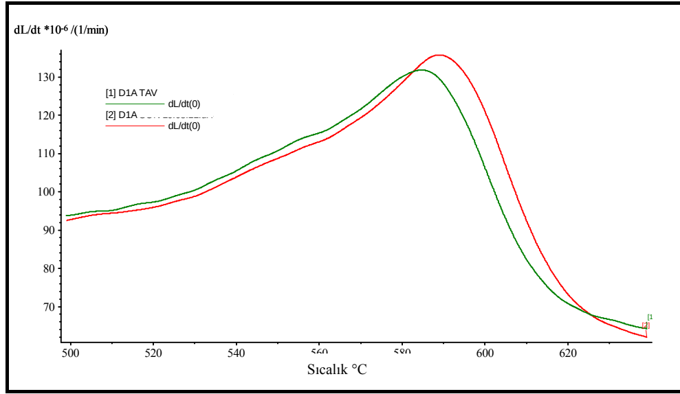
Şekil 3.108.f. Endüstriyel şartlarda hazırlanmış 5x11 boyutlu ve 1090 °C de tavlanmış bünyelerin kuvars dönüşümünün olduğu sıcaklıklarda ısı genleşme eğrileri
