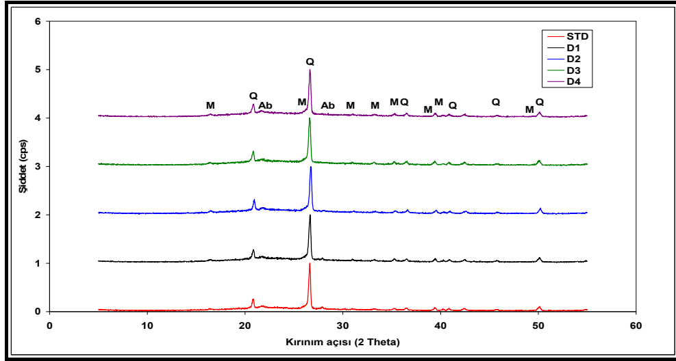
Şekil 3.15. 1. seri numunelere ait XRD grafiği, (M: müllit, Q: kuvars, Ab: albit)
