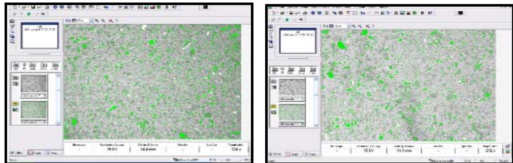
Şekil 3.64. D2A-1 ve D2A-2 bünyelerinin por dağılımı
