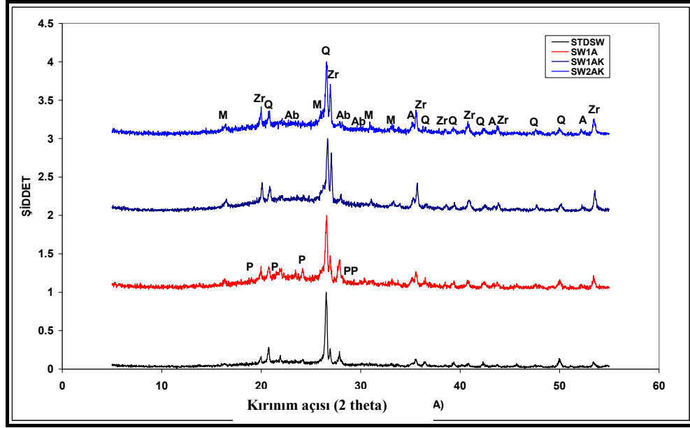
Şekil 3.18. 4. seri numunelere ait XRD grafiği, (M: müllit, Q: kuvars, Ab: albit, P: petalit, A: alümina, Zr: zirkon)
