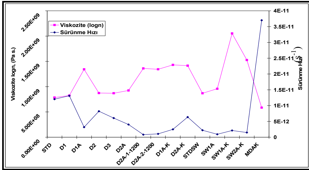
Şekil 3.37. İncelenen bünnyelere ait viskozite değişimine bağlı olarak yüksek sıcaklık sürünme hızı değişimini gösteren eğri
