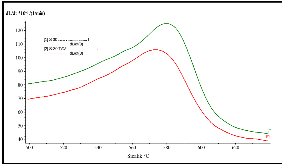
Şekil 3.108.g. Endüstriyel şartlarda hazırlanmış 5x11 boyutlu ve 1090 °C de tavlanmış bünyelerin kuvars dönüşümünün olduğu sıcaklıklarda ısı genleşme eğrileri
