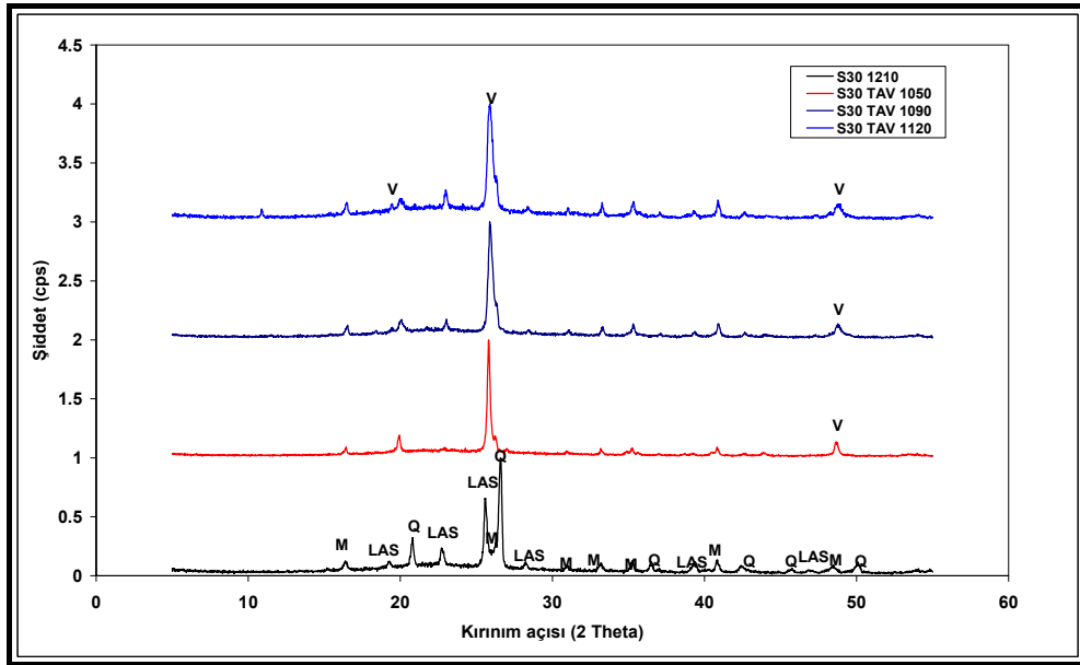
Şekil 3.104. Farklı sıcaklıklarda ısıtılma işlemi görmüş S30 bünyesine ait X ışınları kırınım grafiği, (LAS: lityum alümina silikat, M: müllit, Q. Kuvars)
