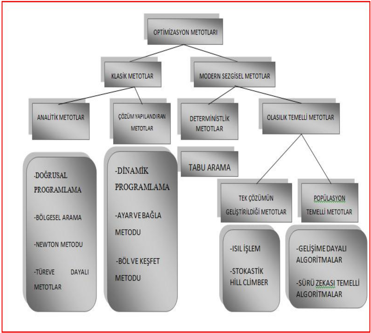
Şekil 5.1 Optimizasyon problemlerinin sınıflandırılması (Akay [52])
