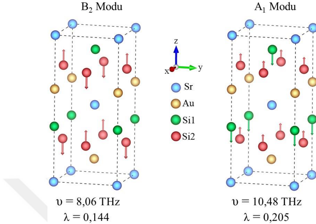
Şekil 4.4. SrAuSi 3 'ün bazı fonon modların öz uzanım vektörlerinin gösterimi
