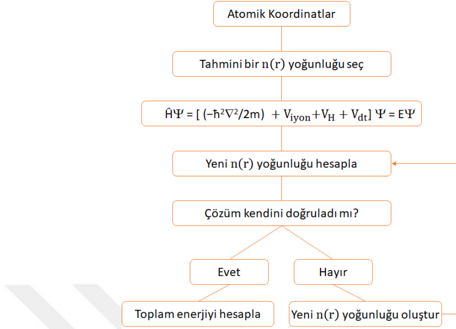
Şekil 3.1. Bir kristalin toplam enerjisini kendini doğrulama metodunu kullanarak hesaplayan bir bilgisayar programının akış çizelgesi
