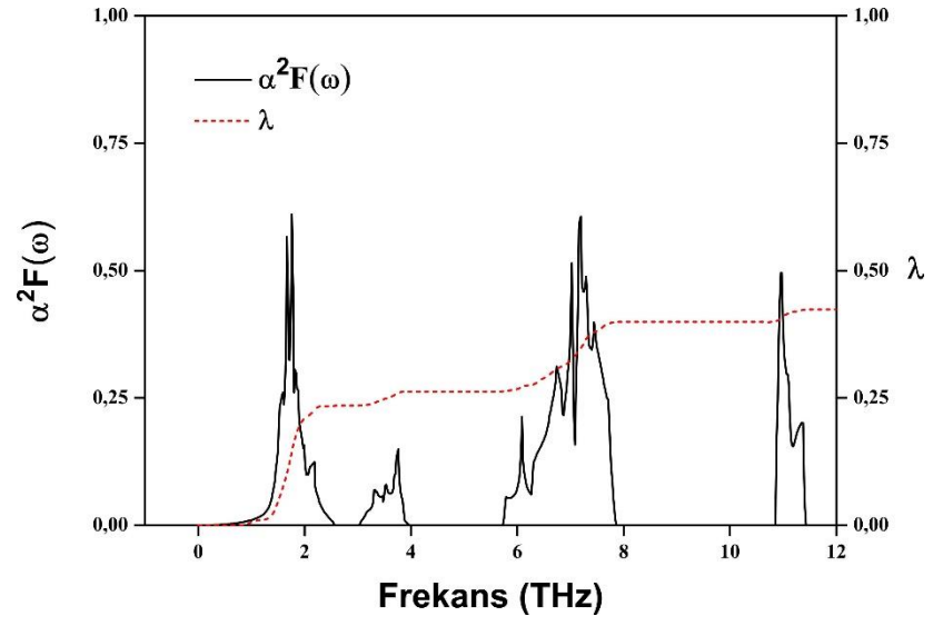
Şekil 4.14. \text{SrAu}_2\text{Si}_2 için Eliashberg Spektral fonksiyonunun elektron-fonon etkileşim parametresinin \lambda ile değişimi
