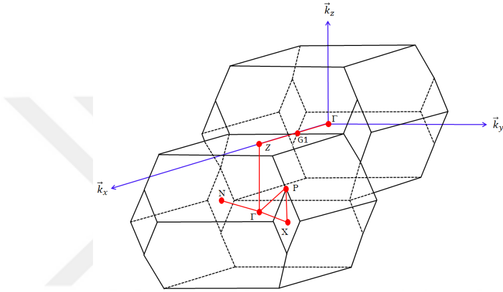
Şekil 2.8. BCT yapının Brillouin bölgesi
