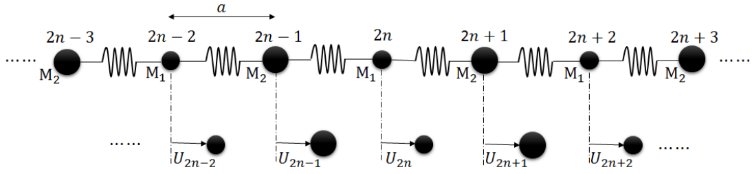
Şekil 2.11. Bir boyutta farklı kütlelere ait atomik örgü titreşimi
