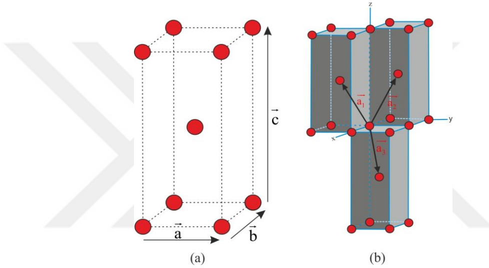
Şekil 2.5. BCT yapı. (a) Birim hücre bravais yapısı, (b) üç boyutta örgü vektörlerinin gösterimi
