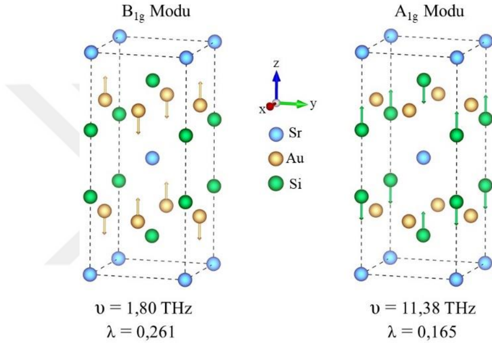
Şekil 4.11. \text{SrAu}_2\text{Si}_2 'nin bazı fonon modların öz uzanım vektörlerinin gösterimi
