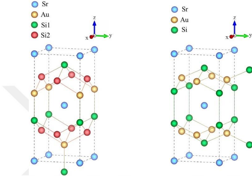
Şekil 2.6. BCT yapıya sahip \text{SrAuSi}_3 (sol tarafta) ve \text{SrAu}_2\text{Si}_2 (sağ tarafta) materyallerinin atomik yapısı
