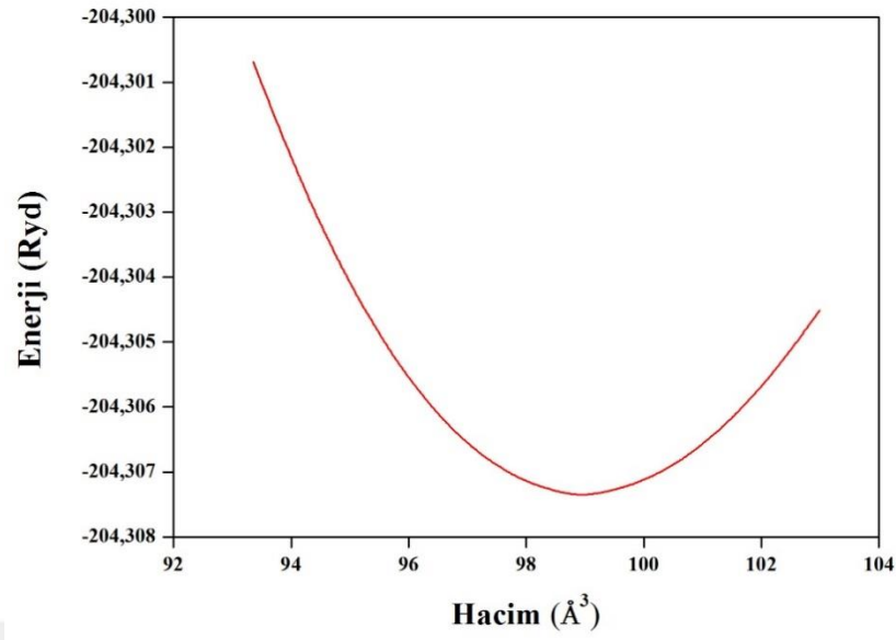
Şekil 4.1. SrAuSi 3 'ün Enerji – Hacim Grafiği
