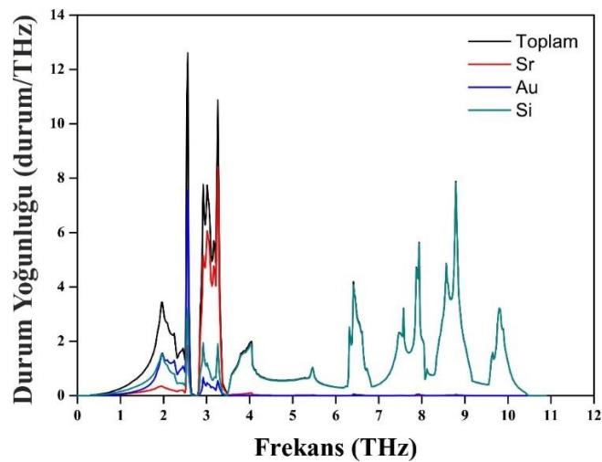
Şekil 4.6. SrAuSi 3 için fonon durum yoğunluğunun gösterimi
