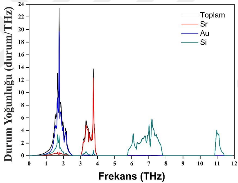
Şekil 4.13. \text{SrAu}_2\text{Si}_2 'nin fonon durum yoğunluğu
