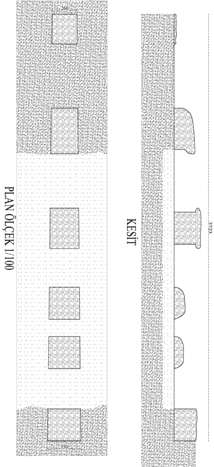
Şekil 4.14. Saklan Köprüsü'nün Mevcut Kalıntılarının (Ayaklarının) Planı
