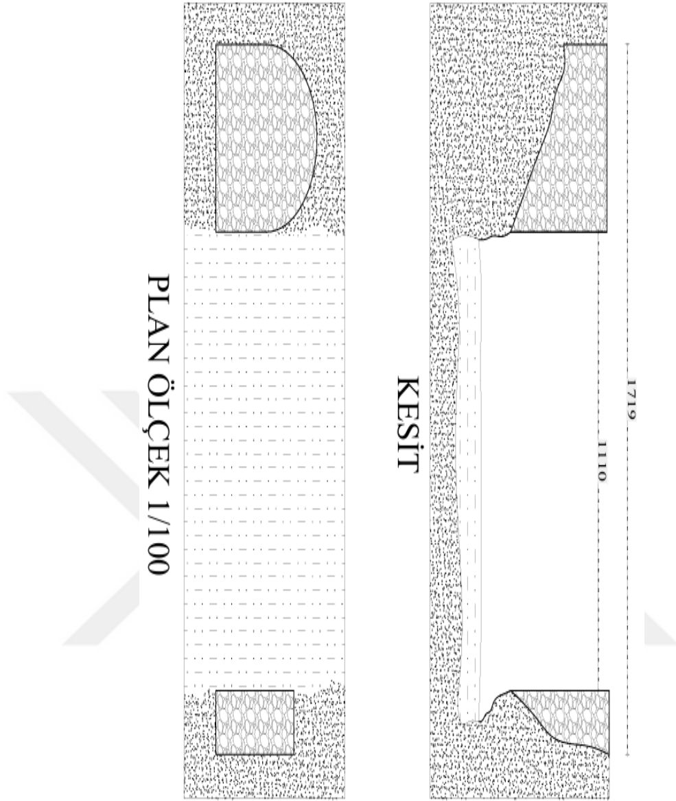
Şekil 4.19. Köprü'nün (Meydan Köprüsü) Planı ve Üstten Görünümü
