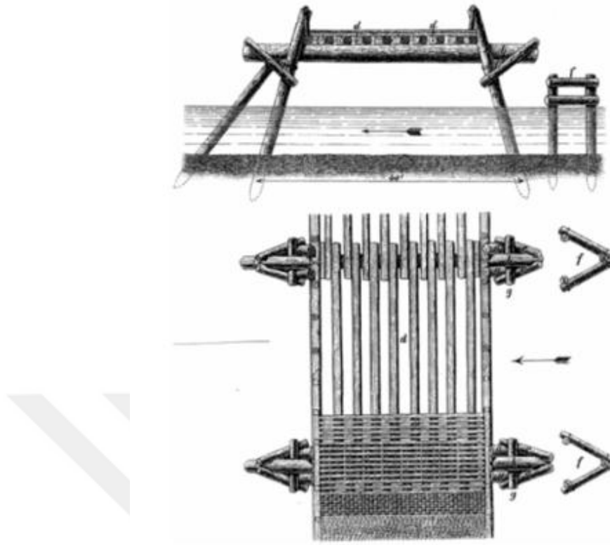
Şekil 3.5. Sezar Köprüsü'nün Kesiti ve Havadan Görünümü
