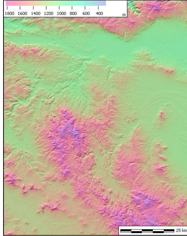
N39E030.hgt SRTM verisi.
