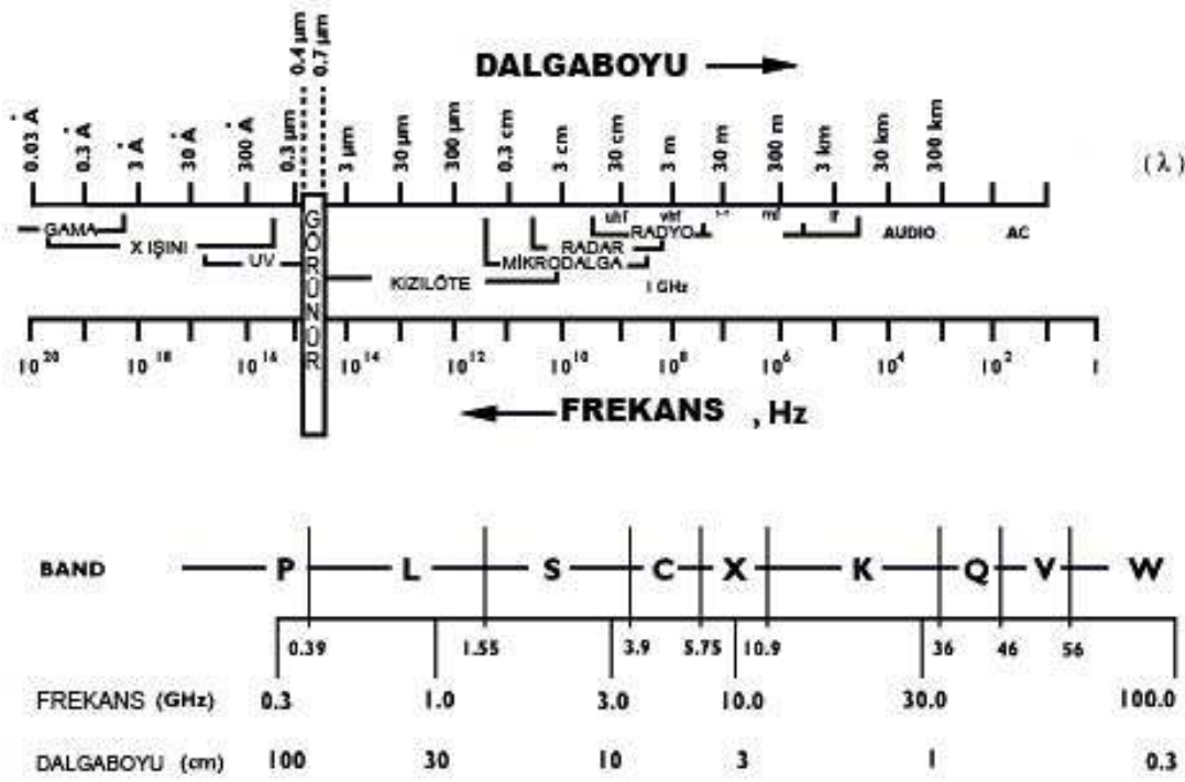
Şekil 3.1 Elektromanyetik spektrum. (Türker, 2004)
