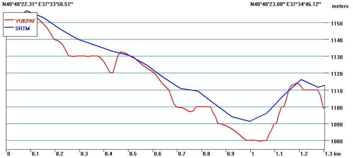
Şekil 4.31 Ormanlık ve dağlık alanda SRTM ile Topografik harita arasındaki farklar
