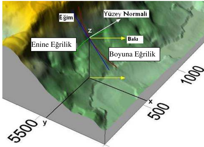
Şekil 2.4 Gradiyent yardımıyla elde edilen parametreler. Mavi çizgi, eğrim; yeşil çizgi, enine eğrilik; kırmızı çizgi boyuna eğrilik.[1]
