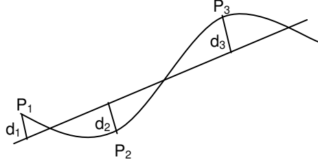
Şekil 2.9 Arazi Yüzeyine uyabilecek düzleme dik doğrultular (Koçak, 1988).
