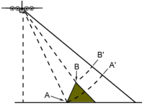
Şekil 3.20 Radar görüntülerindeki bindirme[7].
