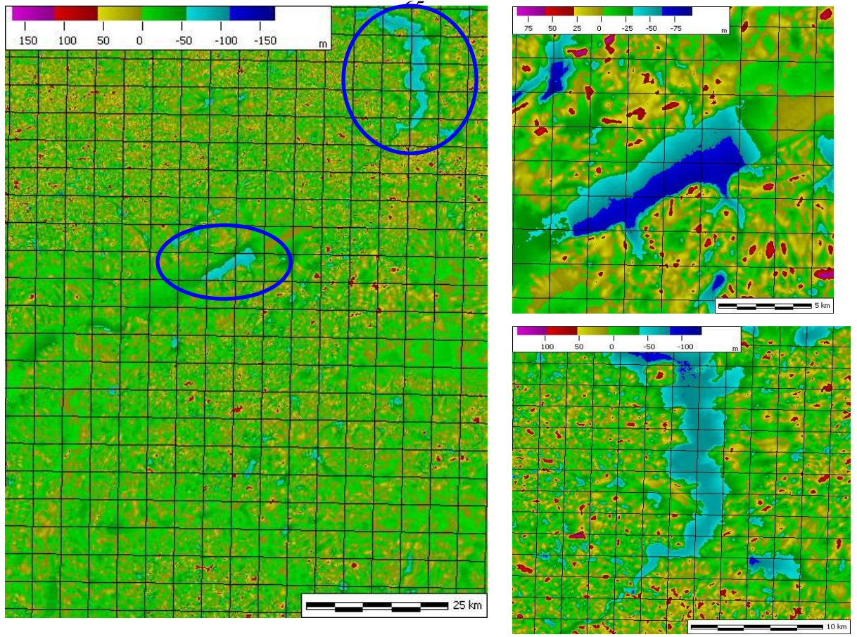
Şekil 4.16 N40E034.hgt ve 3440.dt1 verileri arasındaki yükseklik farkları
