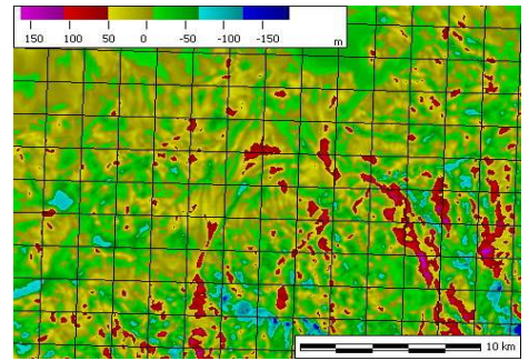
Şekil 4.18 N35E038.hgt ve 3835.dt1 verileri arasındaki yükseklik farkları.
