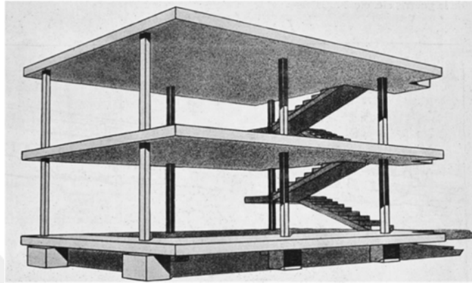
Figure 23. Maison Dom-ino (Corbusier, 2013, p. 234).
