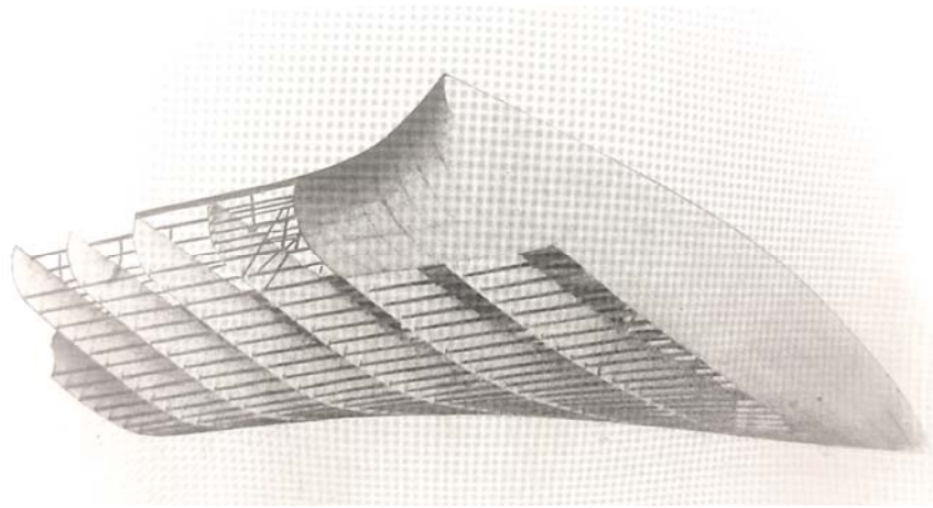
Figure 39. Notre Dame du Haut 's roof construction detail (Ford, 1996, p. 190).
