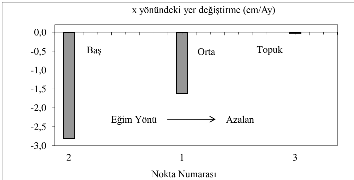
Şekil 6.1. Nisan.2012–Ocak.2014 periyodunda noktaların statik modelle belirlenmiş x yönündeki hareketleri
