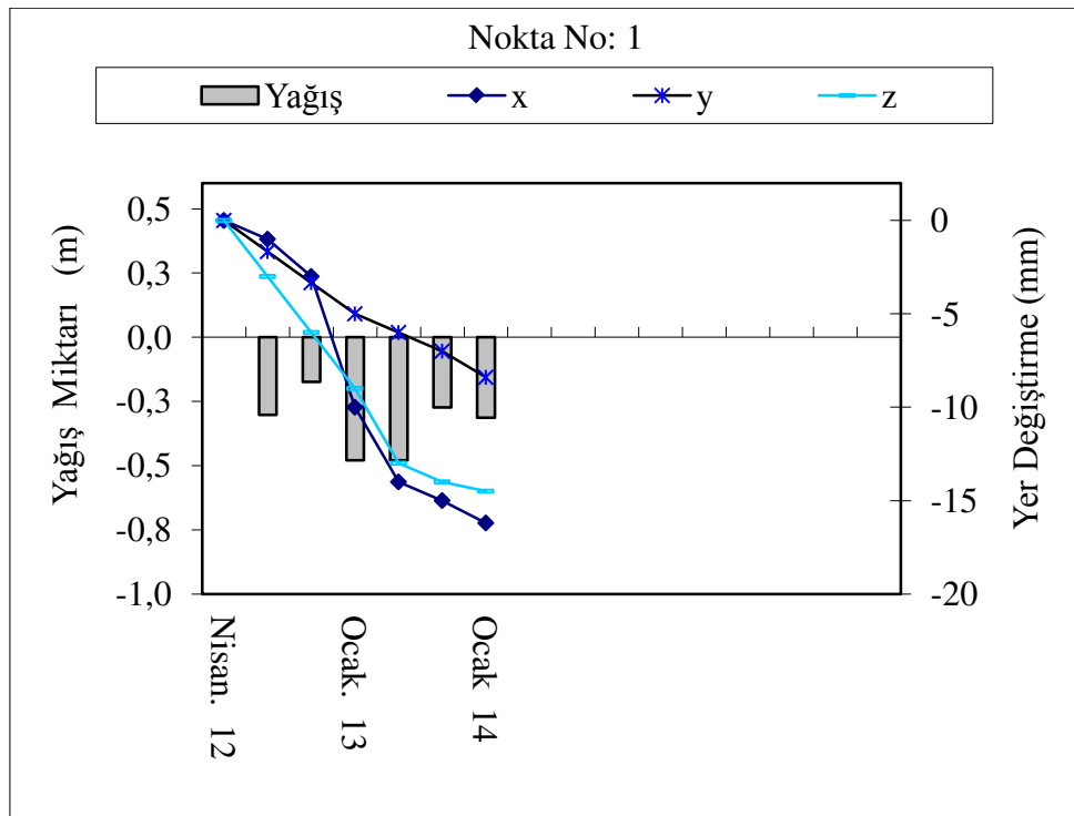
Şekil 6.7. 1 nolu noktanın statik modelle hesaplanmış yer değiştirme-yağış ilişkisi
