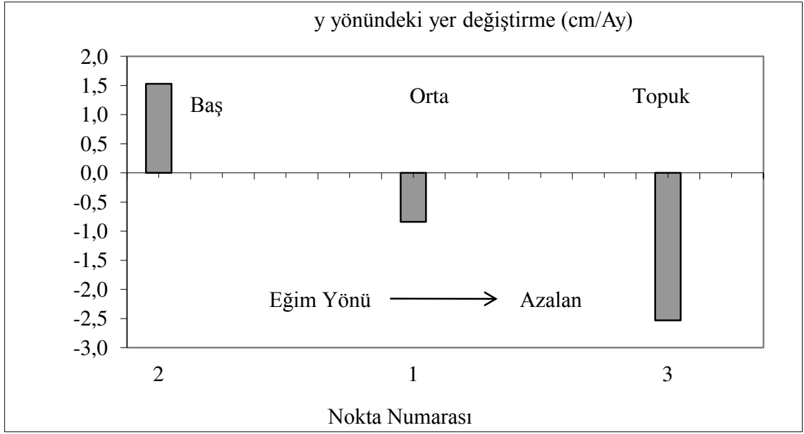
Şekil 6.2. Nisan.2012–Ocak.2014 periyodunda noktaların statik modelle belirlenmiş y yönündeki hareketleri
