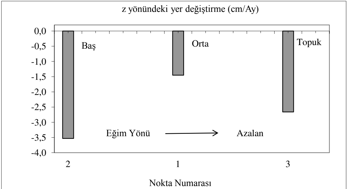
Şekil 6.3. Nisan.2012–Ocak.2014 periyodunda noktaların statik modelle belirlenmiş z yönündeki hareketleri
