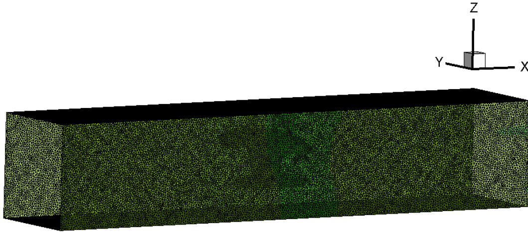
Şekil 2.5 : Çözüm alanının ağ sıklığı.
