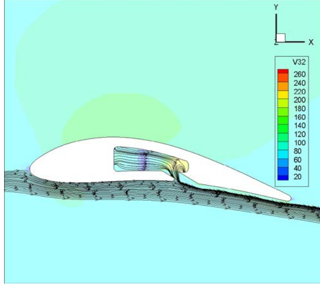
řekil 3.43 : 1,7mm yarıaplı pah, durum 1 – gerek, k-ε analizinin akım izgileri.
