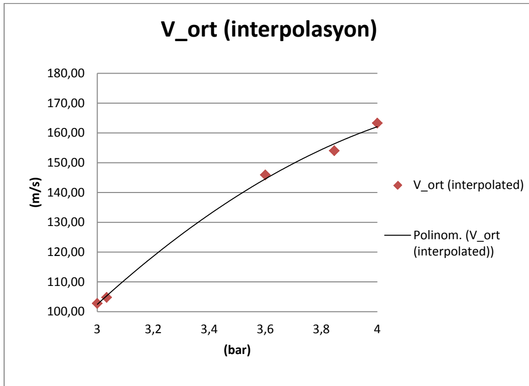
Şekil 4.22 : Interpole edilmiş basınç-hız değerleri.
