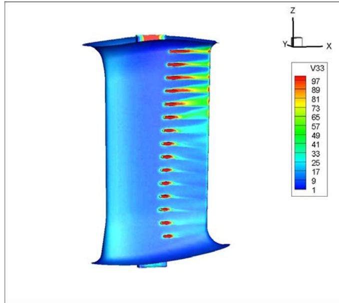
řekil 3.44 : 1,7mm yarıaplı pah, durum 1 – gerek, k-ε analizinde kanatık zerindeki yzey kayma gerilmesi.
