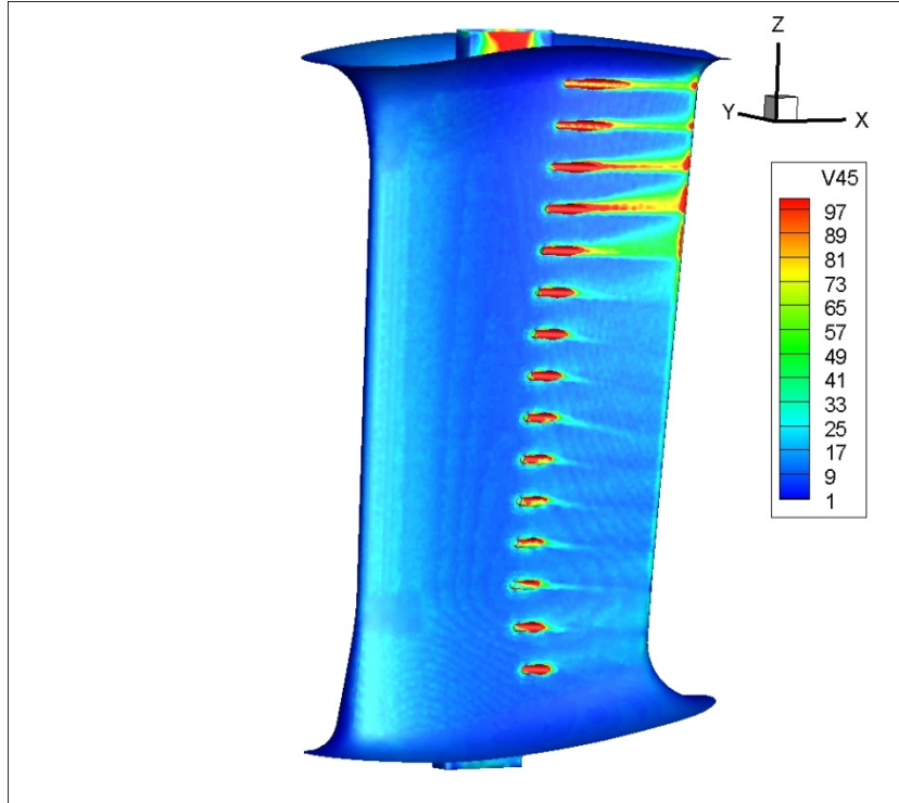
Şekil 3.87 : 2mm yarıçaplı pah, durum 2 – R", LES analizinde kanatçık üzerindeki yüzey kayma gerilmesi.
