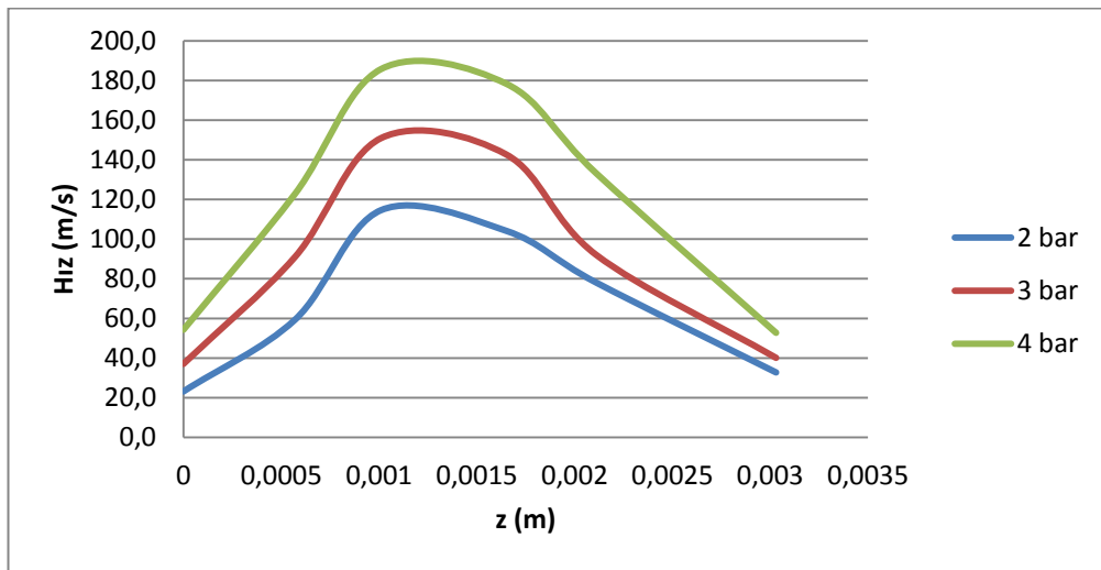
Şekil 4.17 : Hız profili (z ekseninde).
