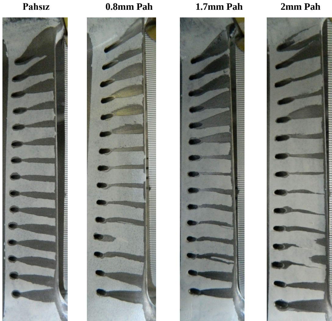
Şekil 4.29 : Durum-1 için farklı pah yarıçaplarındaki deney sonuçları.
