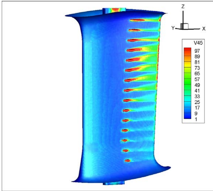
Şekil 3.27 : 0,8mm yarıçaplı pah, durum 2 – R", LES analizinde kanatçık üzerindeki yüzey kayma gerilmesi.
