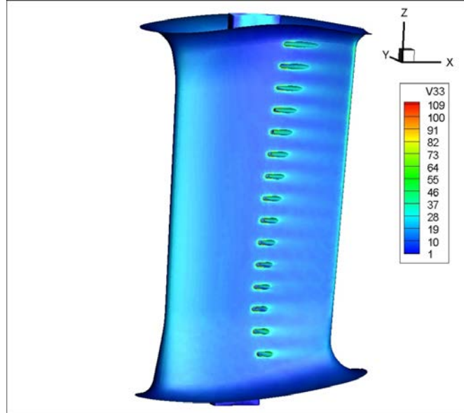
Şekil 3.89 : 2mm yarıçaplı pah, durum 2 – gerçek, k- \epsilon analizinde kanatçık üzerindeki yüzey kayma gerilmesi.
