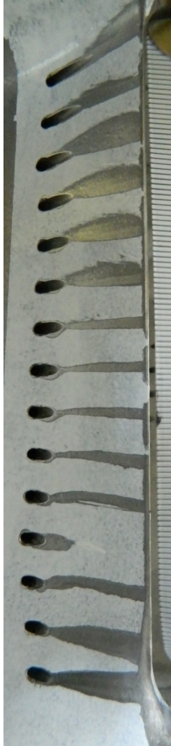
Şekil 4.26 : 0,8 mm yarıçaplı paha sahip kanatçık için farklı jet hızlarındaki deney sonuçları.
