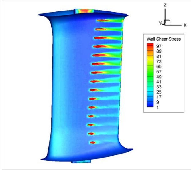
Şekil 3.5 : 0,8 mm pah, Durum 1 - R', k- \epsilon analizinde kanatçık üzerindeki yüzey kayma gerilmesi.
