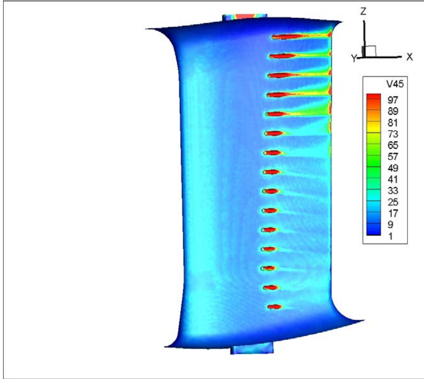
Şekil 3.57 : 1,7mm yarıçaplı pah, durum 2– R", LES kanatçık üzerindeki yüzey kayma gerilmesi.
