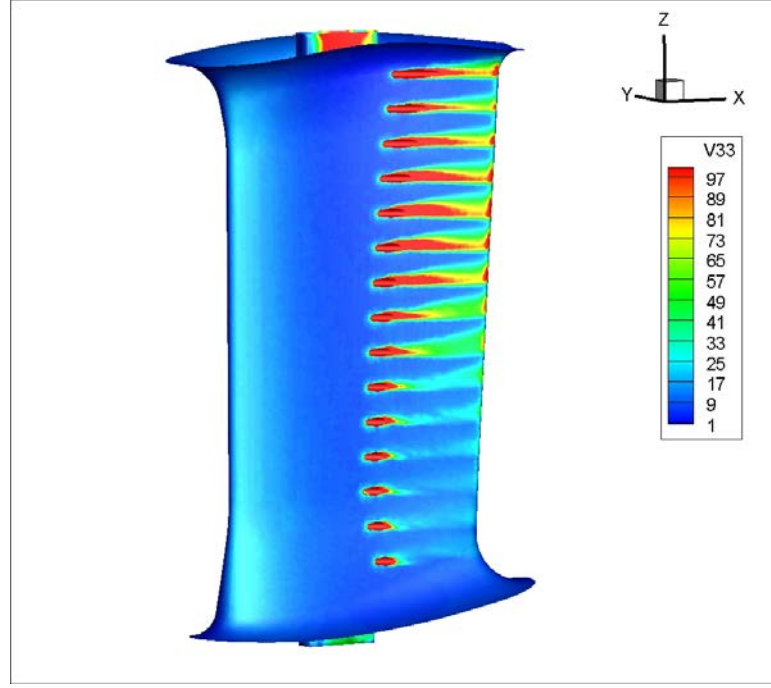
Şekil 3.11 : 0,8mm yarıçaplı pah, durum 1 - R", k-ε analizinde kanatçık üzerindeki yüzey kayma gerilmesi.
