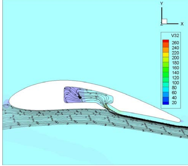
Şekil 3.28 : 0,8mm yarıçaplı pah, durum 2 – gerçek, k-ε analizinin akım çizgileri.
