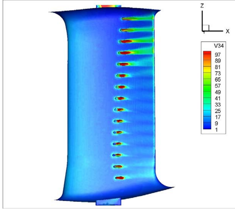
Şekil 3.80 : 2mm yarıçaplı pah, durum 2 – R', k-ε analizinde kanatçık üzerindeki yüzey kayma gerilmesi.
