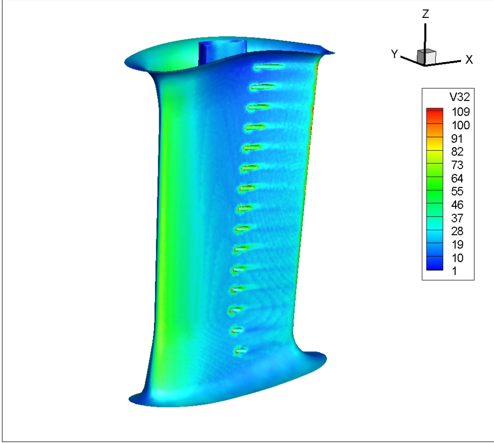
Şekil 3.15 : 0,8mm yarıçaplı pah, durum 1 – gerçek, k-ε analizinde kanatçık üzerindeki yüzey kayma gerilmesi.
