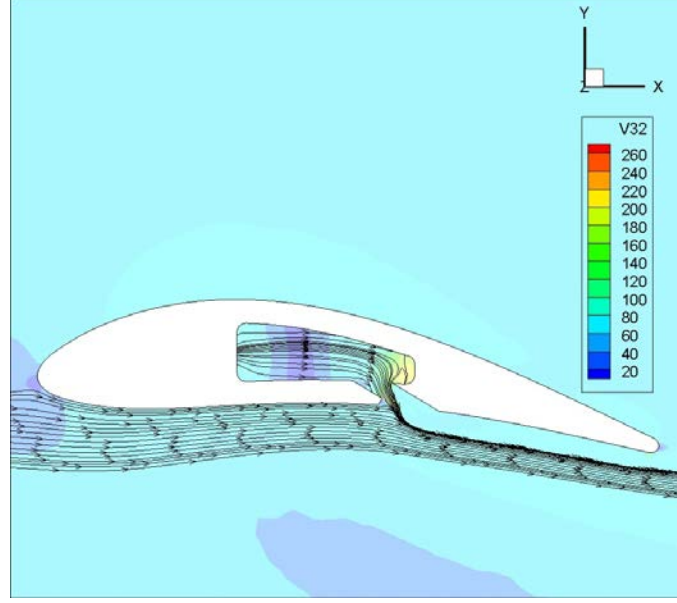
Şekil 3.58 : 1,7mm yarıçaplı pah, durum 2 – gerçek, k-ε analizinin akım çizgileri.
