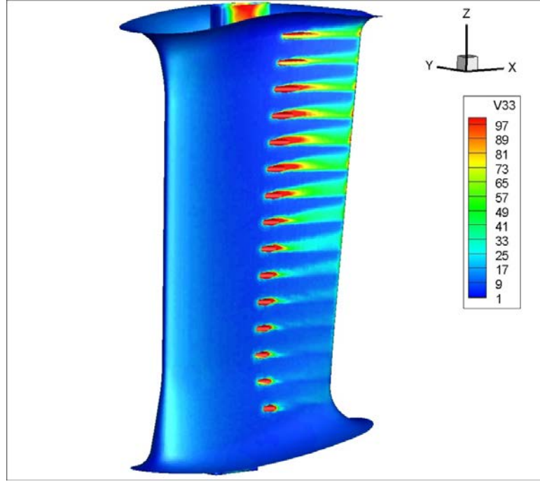
Şekil 3.20 : 0,8mm yarıçaplı pah, durum 2 – R', k-ε analizinde kanatçık üzerindeki yüzey kayma gerilmesi.
