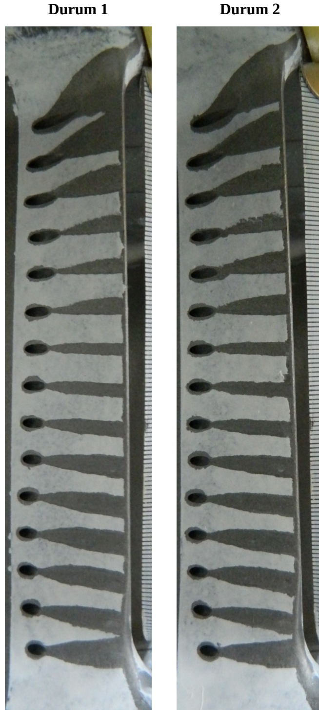
Şekil 4.25 : Pahsız kanatçık için farklı jet hızlarındaki deney sonuçları.
