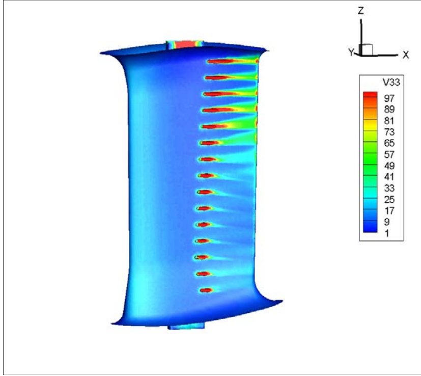
Şekil 3.41 : 1,7mm yarıçaplı pah, durum 1 – R", k-ε analizinde kanatçık üzerindeki yüzey kayma gerilmesi.
