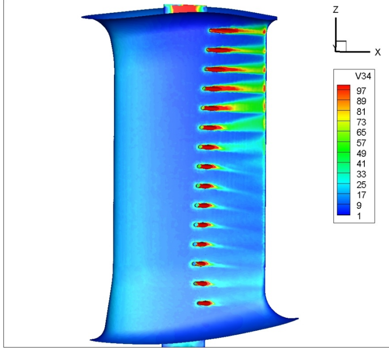
Şekil 3.56 : 1,7mm yarıçaplı pah, durum 2– R", k- \epsilon kanatçık üzerindeki yüzey kayma gerilmesi.
