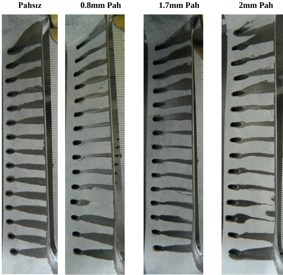
Şekil 4.30 : Durum-2 için farklı pah yarıçaplarındaki deney sonuçları.
