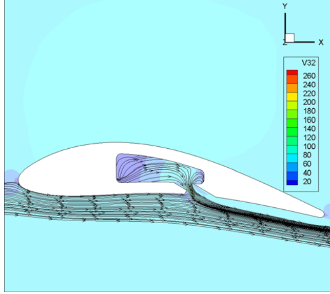
Şekil 3.88 : 2mm yarıçaplı pah, durum 2 – gerçek, k- \epsilon analizinin akım çizgileri.
