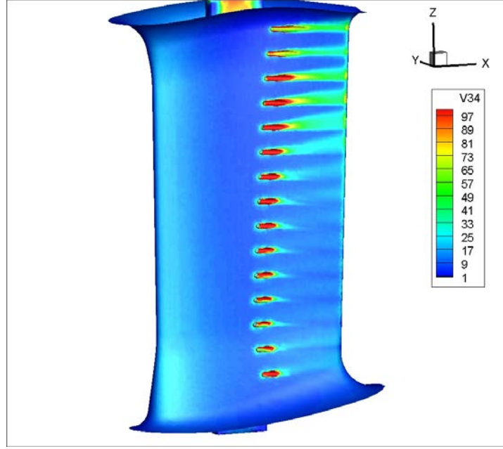
Şekil 3.50 : 1,7mm yarıçaplı pah, durum 2– R', k-ε analizinde kanatçık üzerindeki yüzey kayma gerilmesi.
