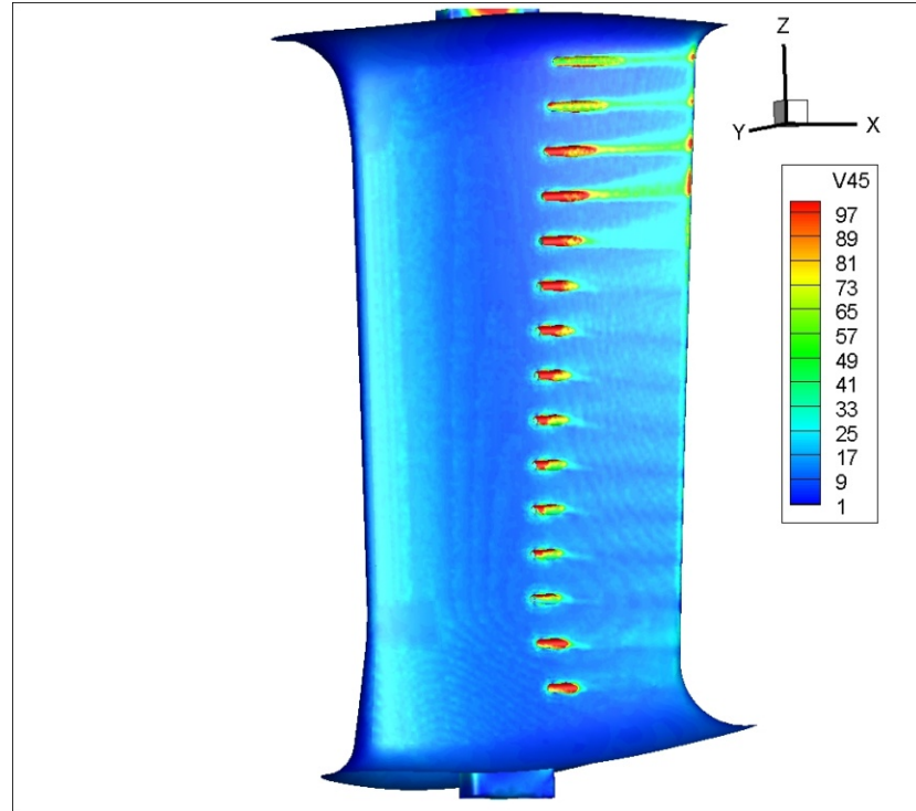
Şekil 3.66 : 2mm yarıçaplı pah, durum 1 – R', LES analizinde kanatçık üzerindeki yüzey kayma gerilmesi.
