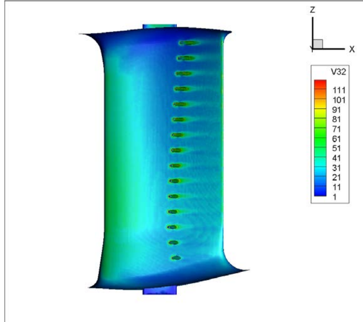
Şekil 3.29 : 0,8mm yarıçaplı pah, durum 2 – gerçek, k-ε analizinde kanatçık üzerindeki yüzey kayma gerilmesi.
