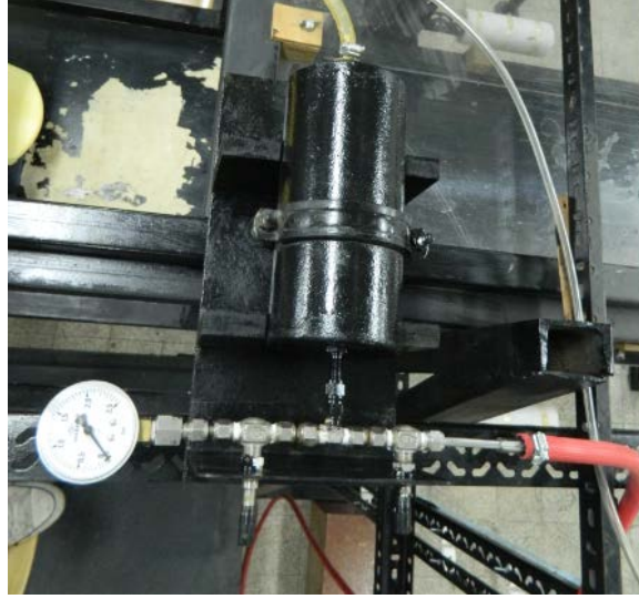
Şekil 4.6 : Regülatör II.
