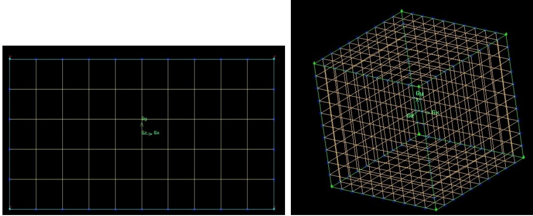
Şekil 2.2 : İki ve üç boyutlu yapılandırılmış (structured) ağ hücreleri [11].
