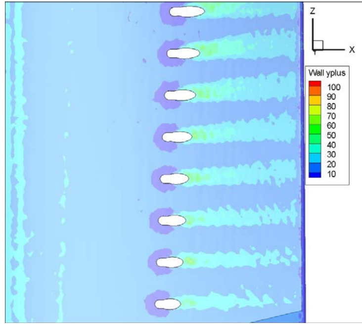
Şekil 2.13 : 0,8 mm yarıçapında pah kırılmış modelin y^+ değerleri.
