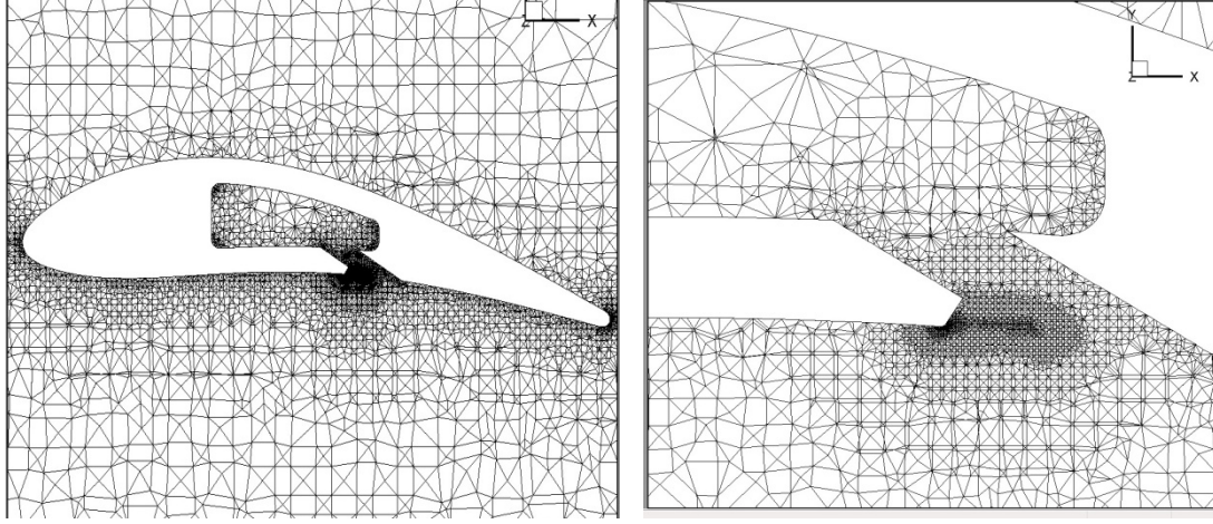
Şekil 2.4 : Pah kırılan bölgedeki ağ sıklığı.
