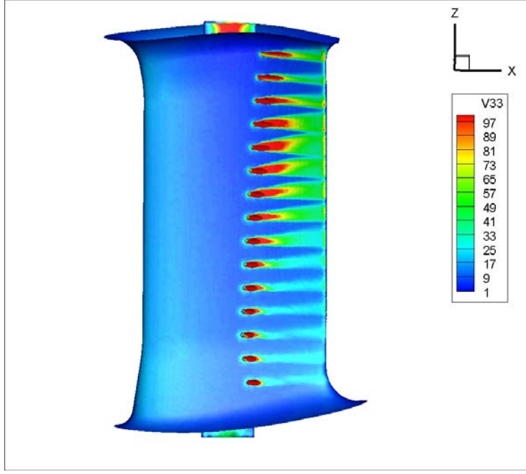
Şekil 3.26 : 0,8mm yarıçaplı pah, durum 2 – R", k-ε analizinde kanatçık üzerindeki yüzey kayma gerilmesi.
