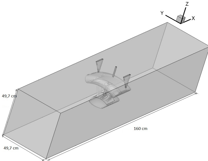
Şekil 2.1 : Çözüm alanı geometrisi.
