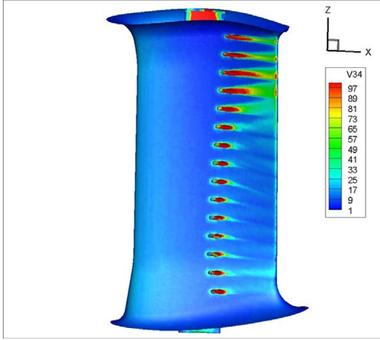
Şekil 3.71 : 2mm yarıçaplı pah, durum 1 – R", k-ε analizinde kanatçık üzerindeki yüzey kayma gerilmesi.
