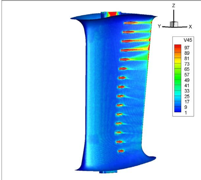
Şekil 3.72 : 2mm yarıçaplı pah, durum 1 – R", LES analizinde kanatçık üzerindeki yüzey kayma gerilmesi.
