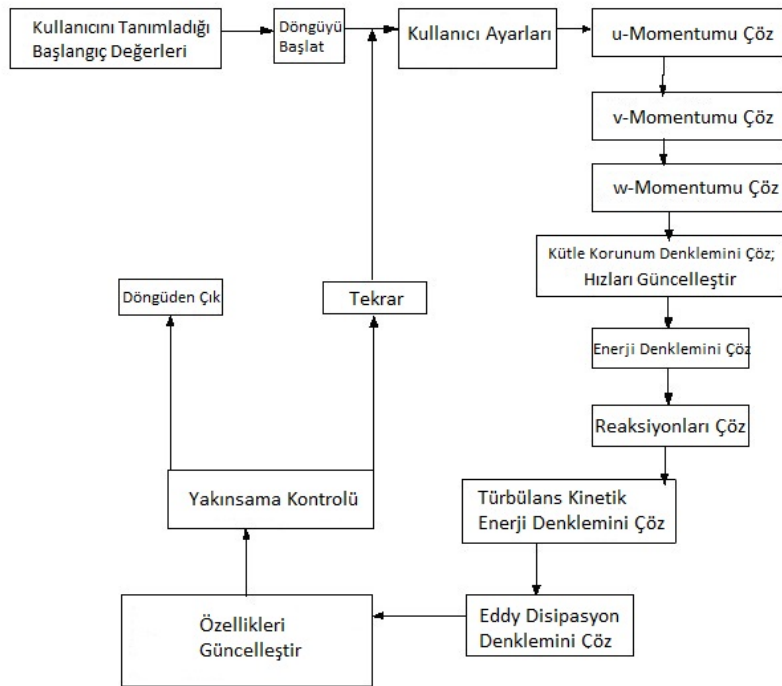
Şekil 2.7 : Basınç temelli çözüm algoritması [11].
