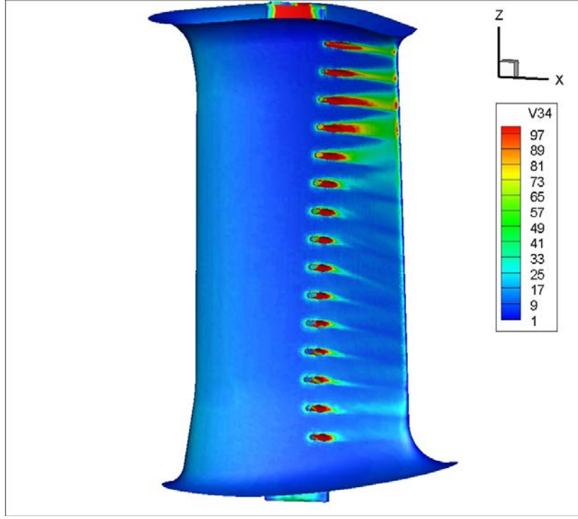
Şekil 3.86 : 2mm yarıçaplı pah, durum 2 – R", k-ε analizinde kanatçık üzerindeki yüzey kayma gerilmesi.
