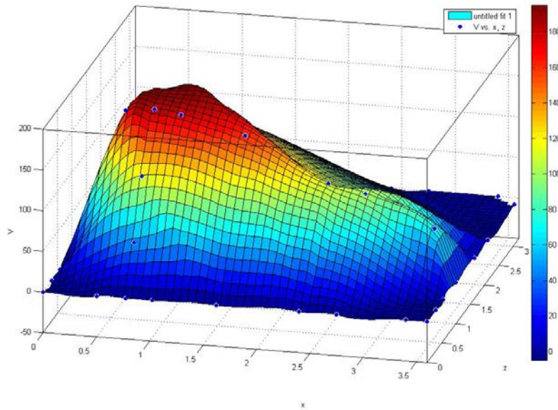
Şekil 4.19 : 3 boyutlu hız profili.
