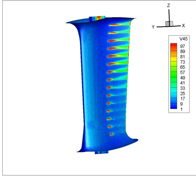
Şekil 3.6 : 0,8 mm pah, Durum 1 - R', LES analizinde kanatçık üzerindeki yüzey kayma gerilmesi.
