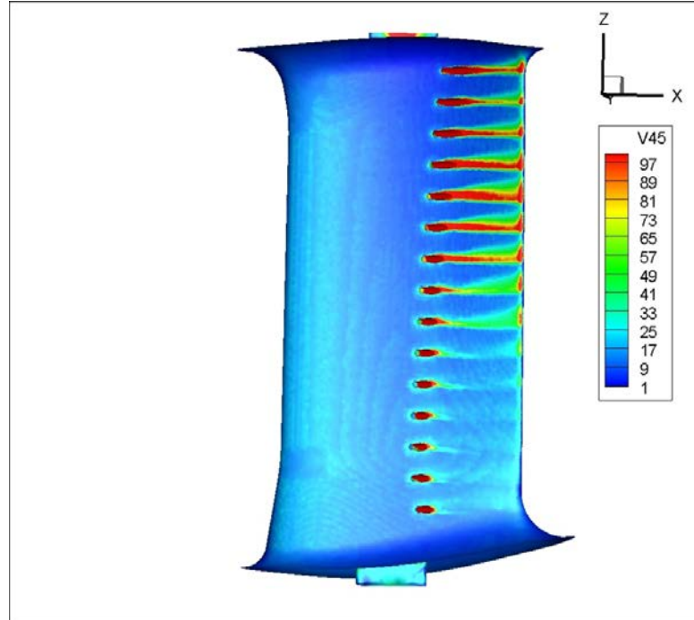
Şekil 3.12 : 0,8mm yarıçaplı pah, durum 1 - R", LES analizinde kanatçık üzerindeki yüzey kayma gerilmesi.
