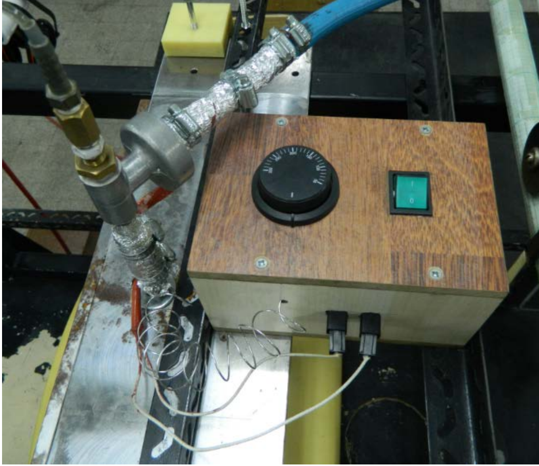
Şekil 4.8 : Isıtıcı sistem.
