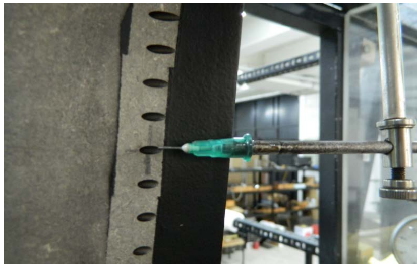
Şekil 4.13 : İğne pitot tübü.
