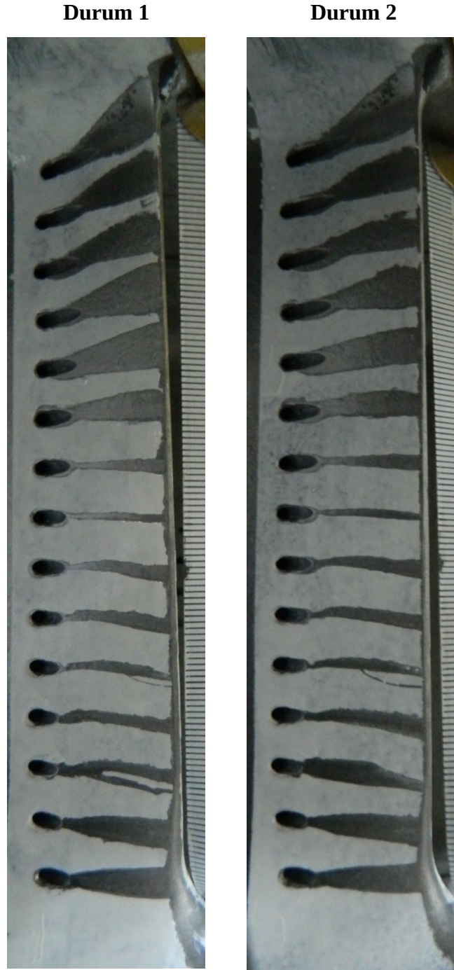
Şekil 4.27 : 1,7 mm yarıçaplı paha sahip kanatçık için farklı jet hızlarındaki deney sonuçları.
