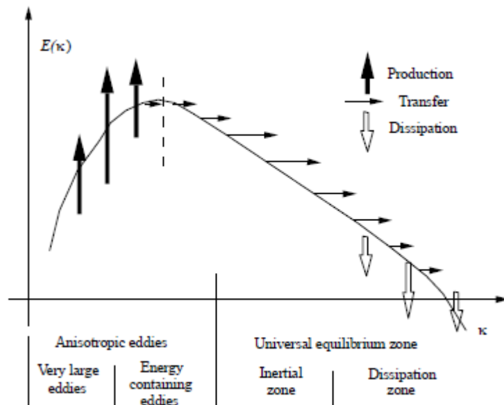
Şekil 1.3 : Türbülans enerji sepektrumu [8].
