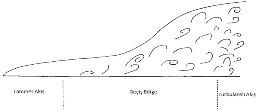
Şekil 2.9 : Düz levhadaki akışta türbülansa geçiş aşamaları [14].
