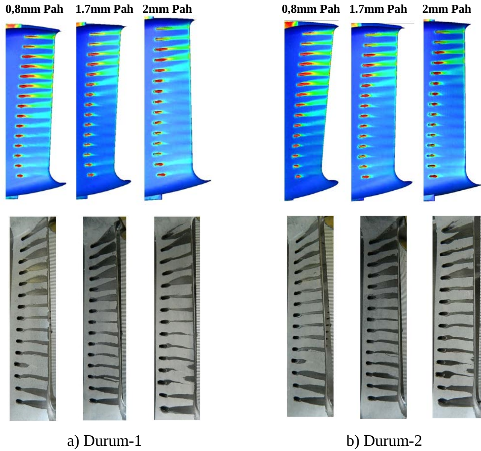
Şekil 5.1 : Sayısal ve deneysel analiz sonuçları.
