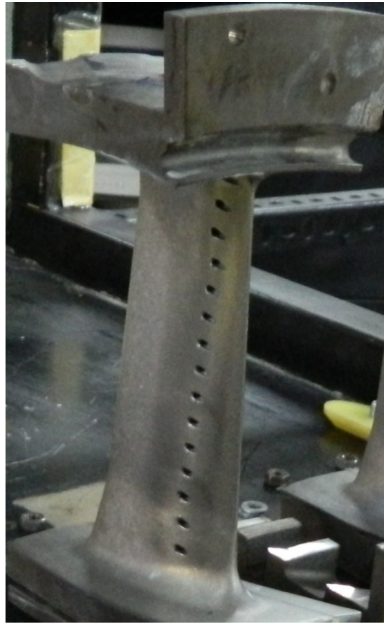
Şekil 1.1 : Kanatçıklara açılan kanallar.
