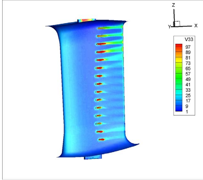
Şekil 3.65 : 2mm yarıçaplı pah, durum 1 – R', k-ε analizinde kanatçık üzerindeki yüzey kayma gerilmesi.
