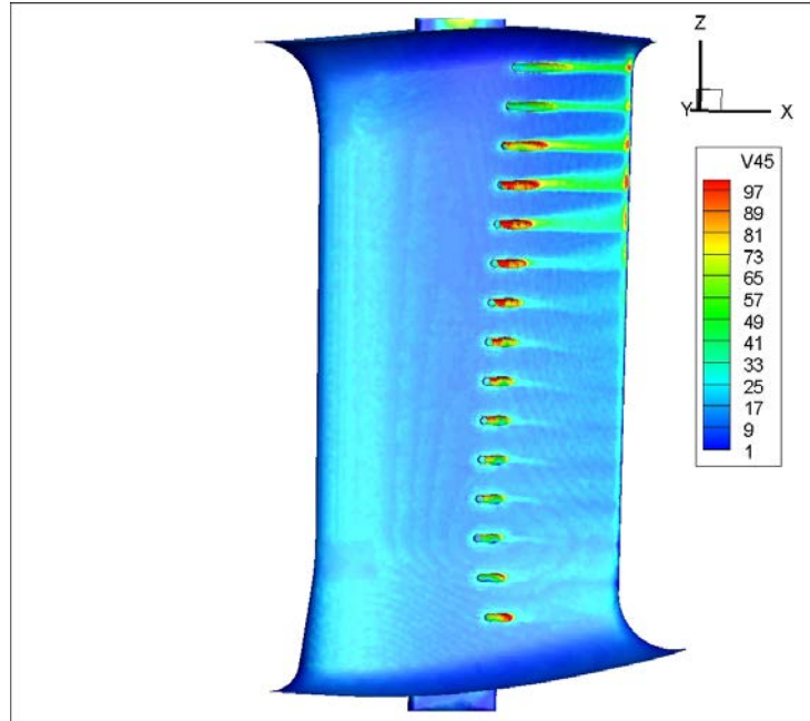
Şekil 3.51 : 1,7mm yarıçaplı pah, durum 2– R', LES analizinde kanatçık üzerindeki yüzey kayma gerilmesi.
