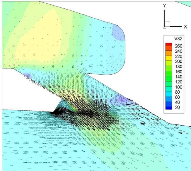
Şekil 3.75 : 2mm yarıçaplı pah, durum 1 – gerçek, k-ε analizinin hız vektörleri.
