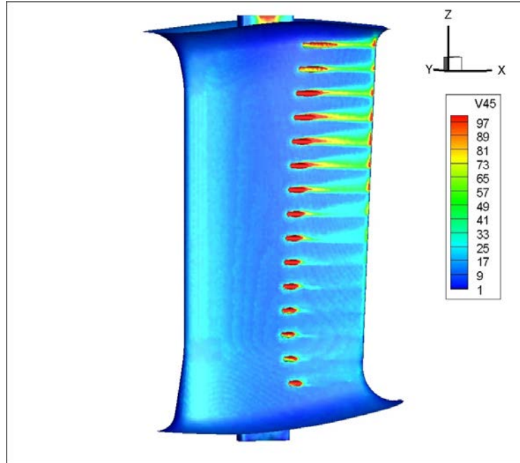
Şekil 3.21 : 0,8mm yarıçaplı pah, durum 2 – R', LES analizinde kanatçık üzerindeki yüzey kayma gerilmesi.
