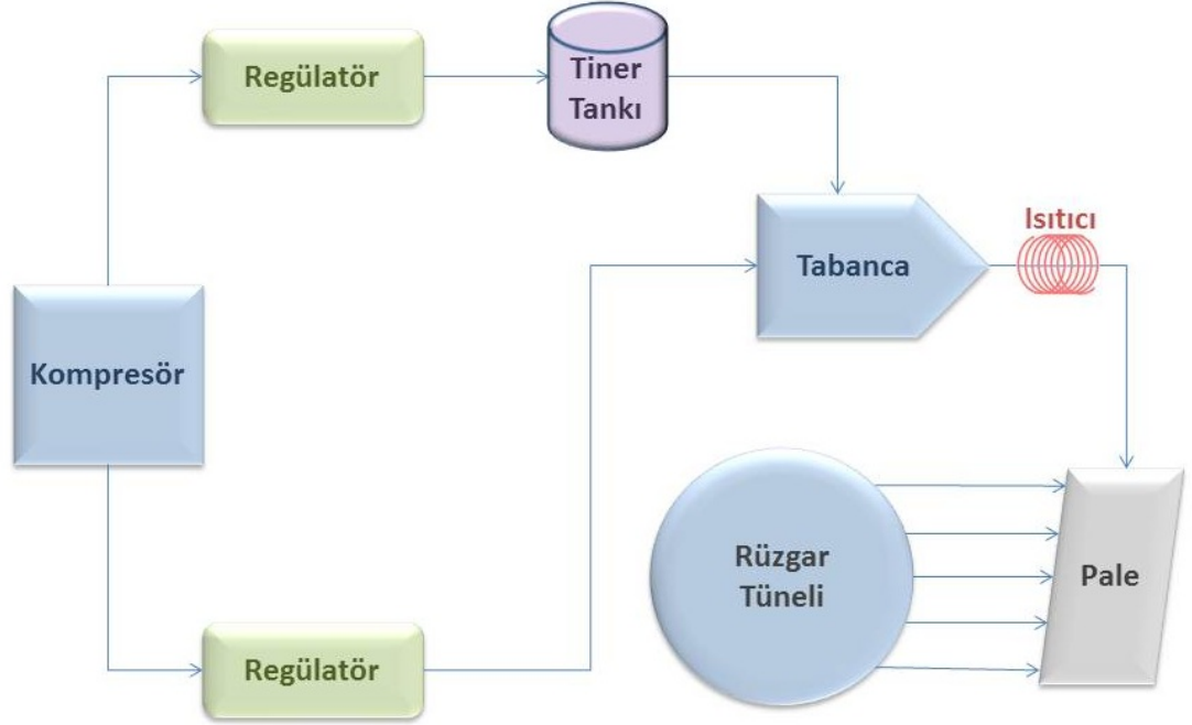
Şekil 4.23 : Deney şeması.
