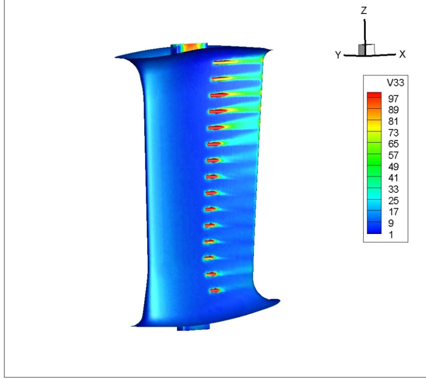
Şekil 3.35 : 1,7mm yarıçaplı pah, durum 1 – R', k-ε analizinde kanatçık üzerindeki yüzey kayma gerilmesi.
