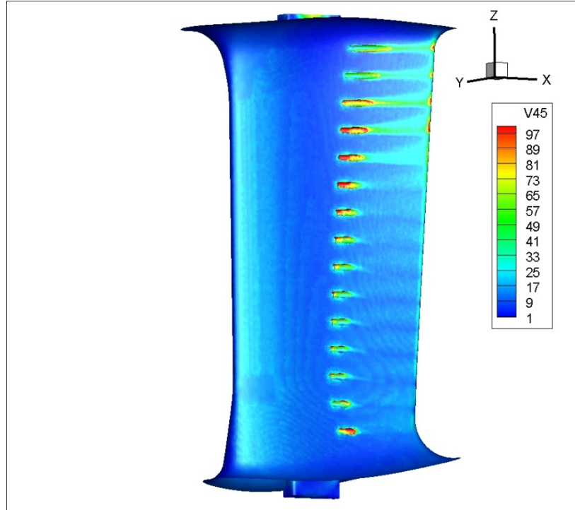
Şekil 3.81 : 2mm yarıçaplı pah, durum 2 – R', LES analizinde kanatçık üzerindeki yüzey kayma gerilmesi.
