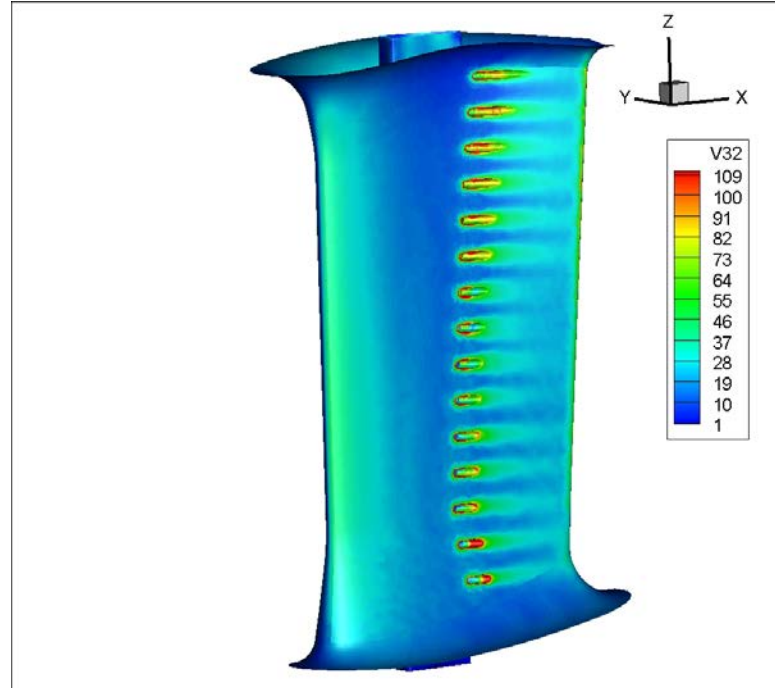
řekil 3.74 : 2mm yarıaplı pah, durum 1 – gerek, k-ε analizinde kanatık zerindeki yzey kayma gerilmesi.
