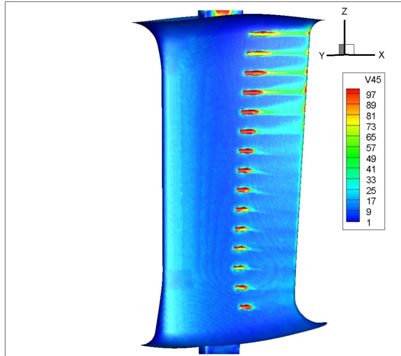
Şekil 3.36 : 1,7mm yarıçaplı pah, durum 1 – R', LES analizinde kanatçık üzerindeki yüzey kayma gerilmesi.
