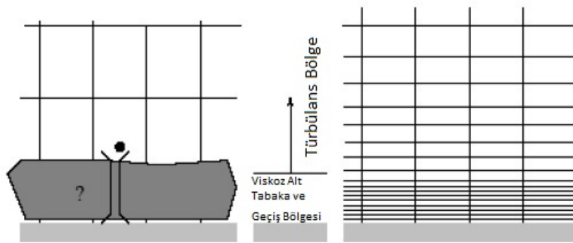
a) Yüzey fonksiyonu yaklaşımı b) Yüzey modelleme yaklaşımı
