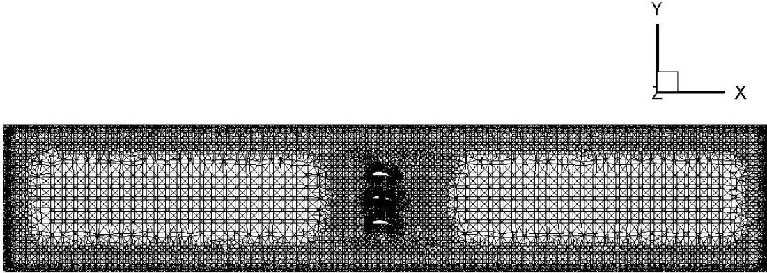
Şekil 2.6 : Yüzeylere yakın bölgelerdeki ağ sıklığı.
