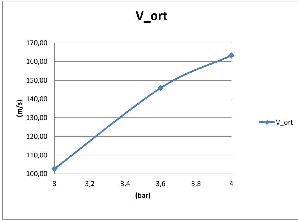
Şekil 4.21 : Kompresör basıncına göre ölçülen hız değerleri.
