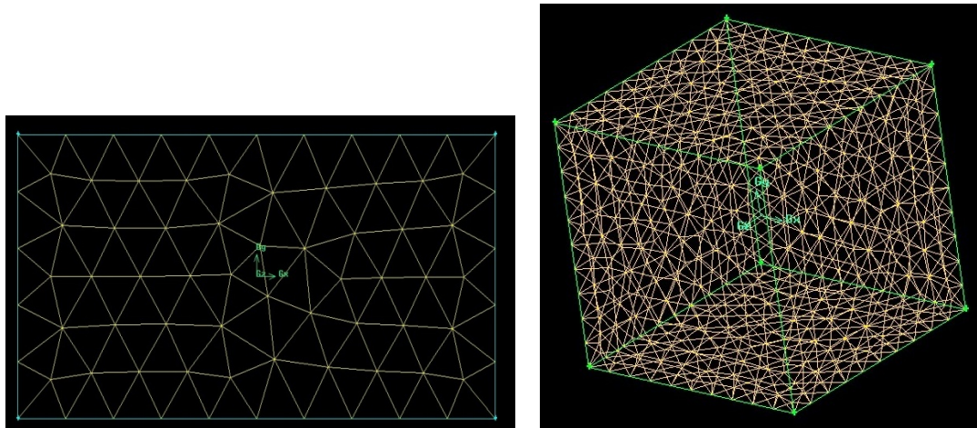
Şekil 2.3 : İki ve üç boyutlu yapılandırılmamış (unstructured) ağ hücreleri [11].
