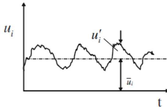
Şekil 2.10 : Türbülanslı akışta bir noktadaki hızın zamanla değişimi [15].
