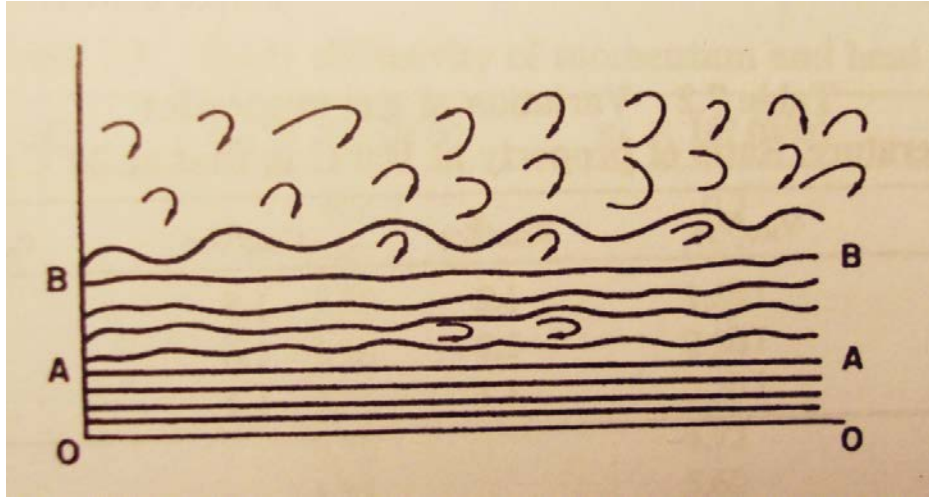
Şekil 2.11 : Yüzeye yakın akış bölgeleri [13].
