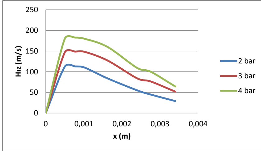
Şekil 4.18 : Hız profili (x ekseninde).
