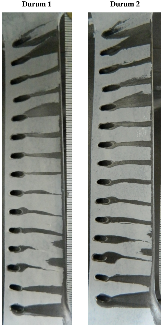
Şekil 4.28 : 2 mm Yarıçaplı paha sahip kanatçık için farklı jet hızlarındaki deney sonuçları.
