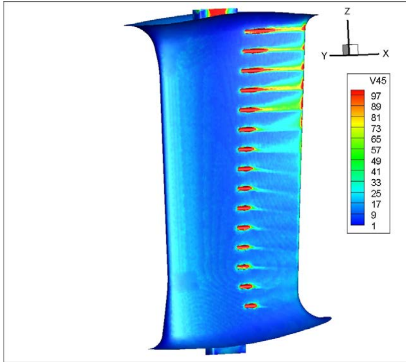
Şekil 3.42 : 1,7mm yarıçaplı pah, durum 1 – R", LES analizinde kanatçık üzerindeki yüzey kayma gerilmesi.
