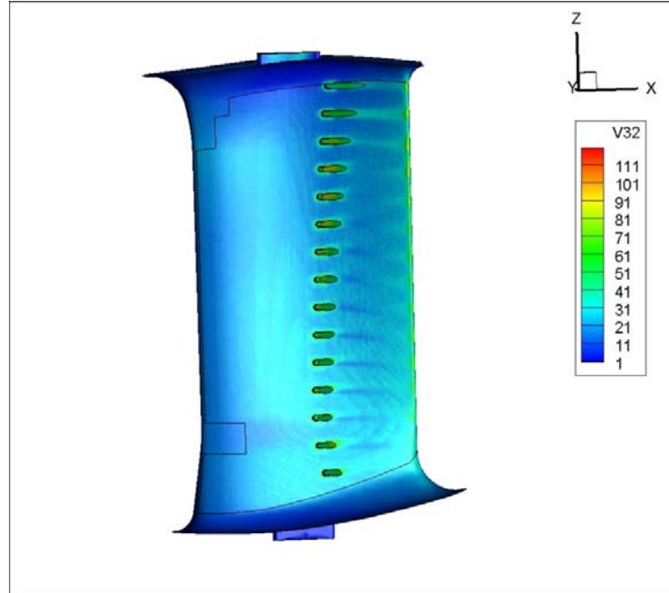
Şekil 3.59 : 1,7mm yarıçaplı pah, durum 2 – gerçek, k-ε analizinde kanatçık üzerindeki yüzey kayma gerilmesi.
