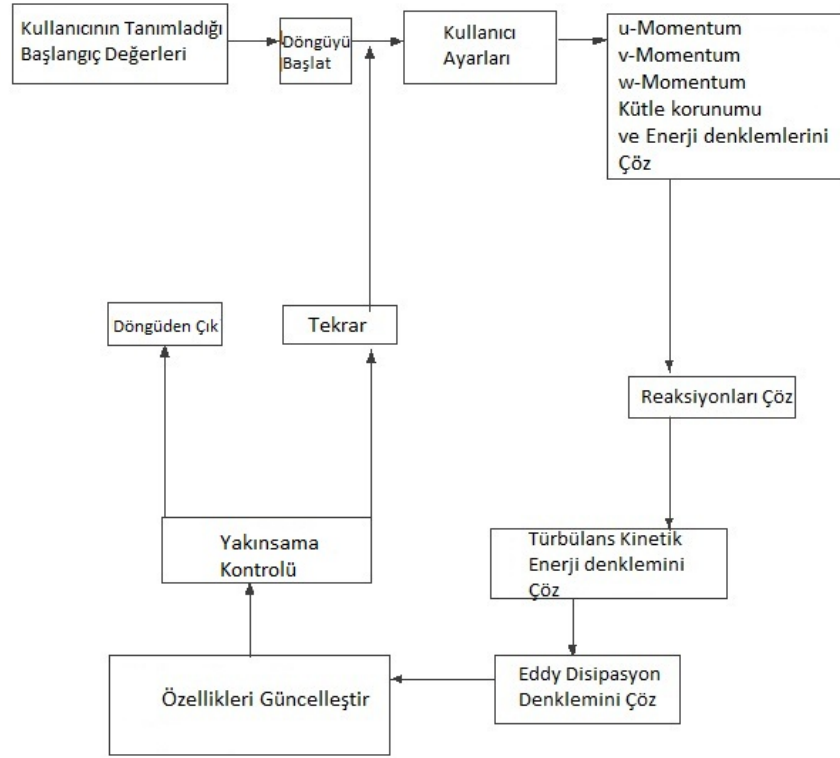
Şekil 2.8 : Yoğunluk temelli çözüm algoritması [11].
