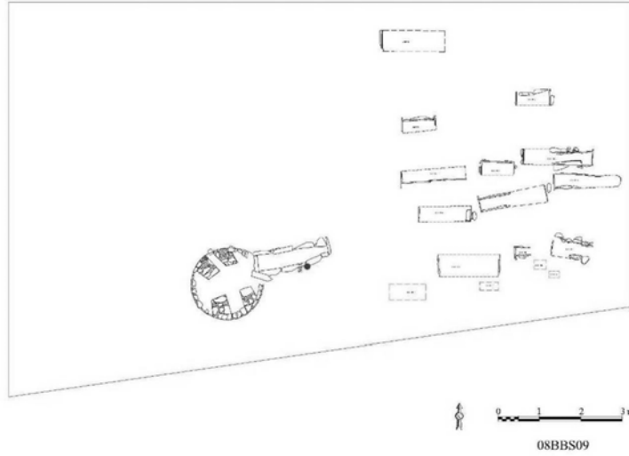
Şekil 31. Beybağ 08BBS09 no.lu sondaj planı
