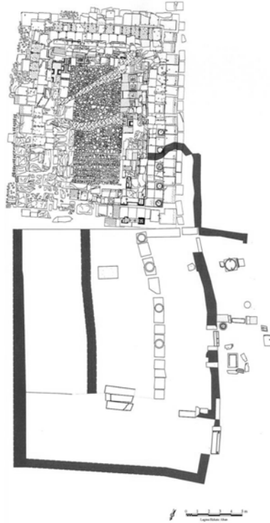
Şekil 12. Lagina Kutsal Alanı'ndaki Bizans Dönemi kilisesi planı
