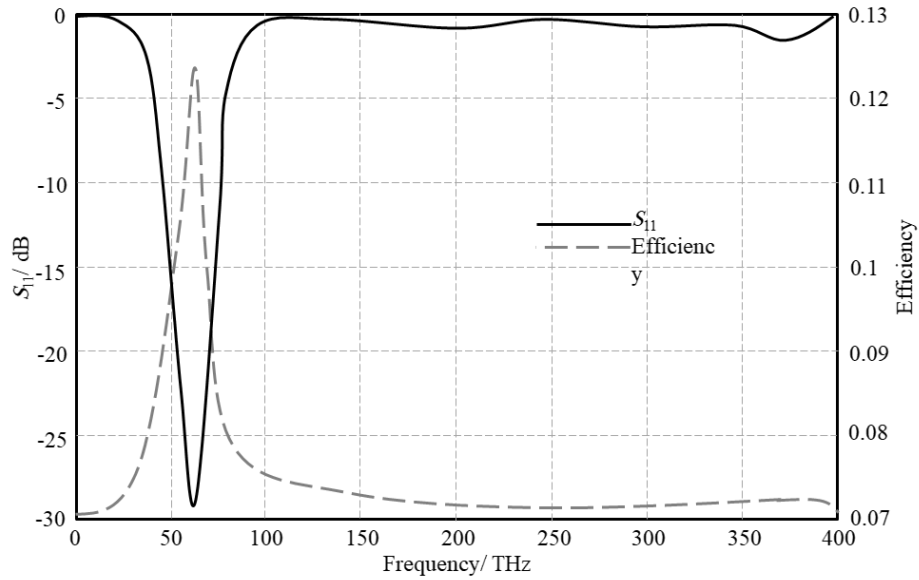
Şekil 4.7. SILICON_2 anteni için S_{11} ve \eta_r spektrumları
