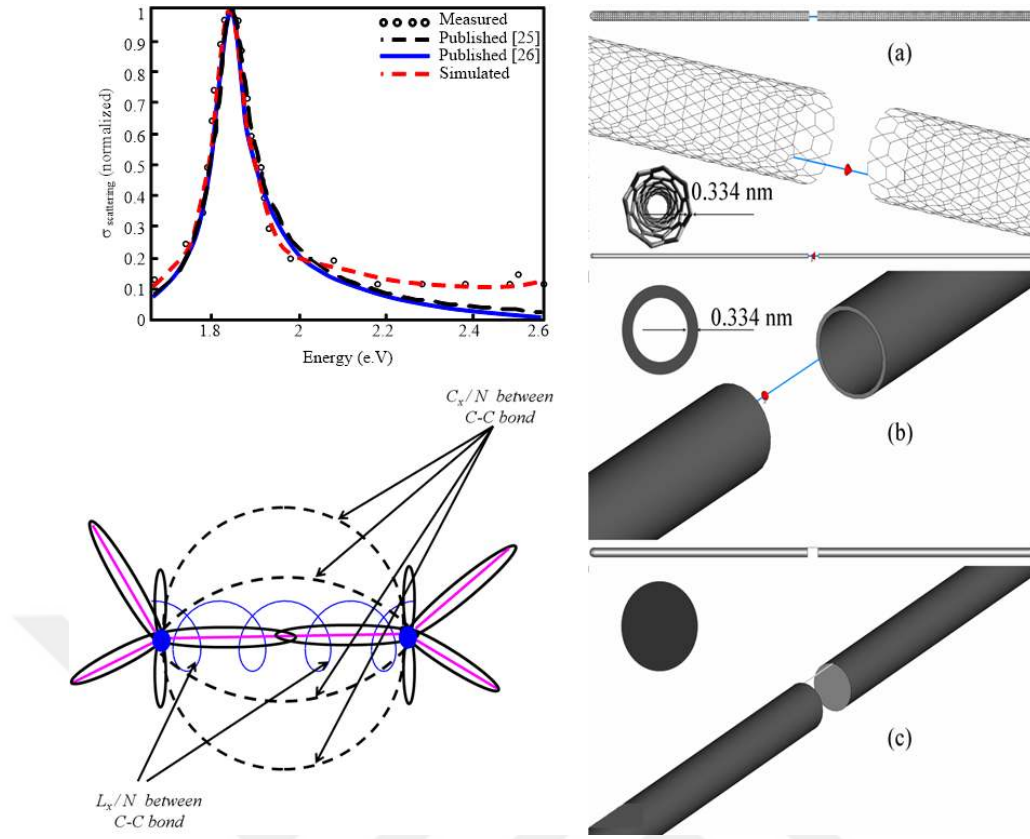
Şekil 2.2. Plazmonik etkiler: (a) spektroskopi, (b) anten modeli ve (c) CC bağ elektron hareketi
