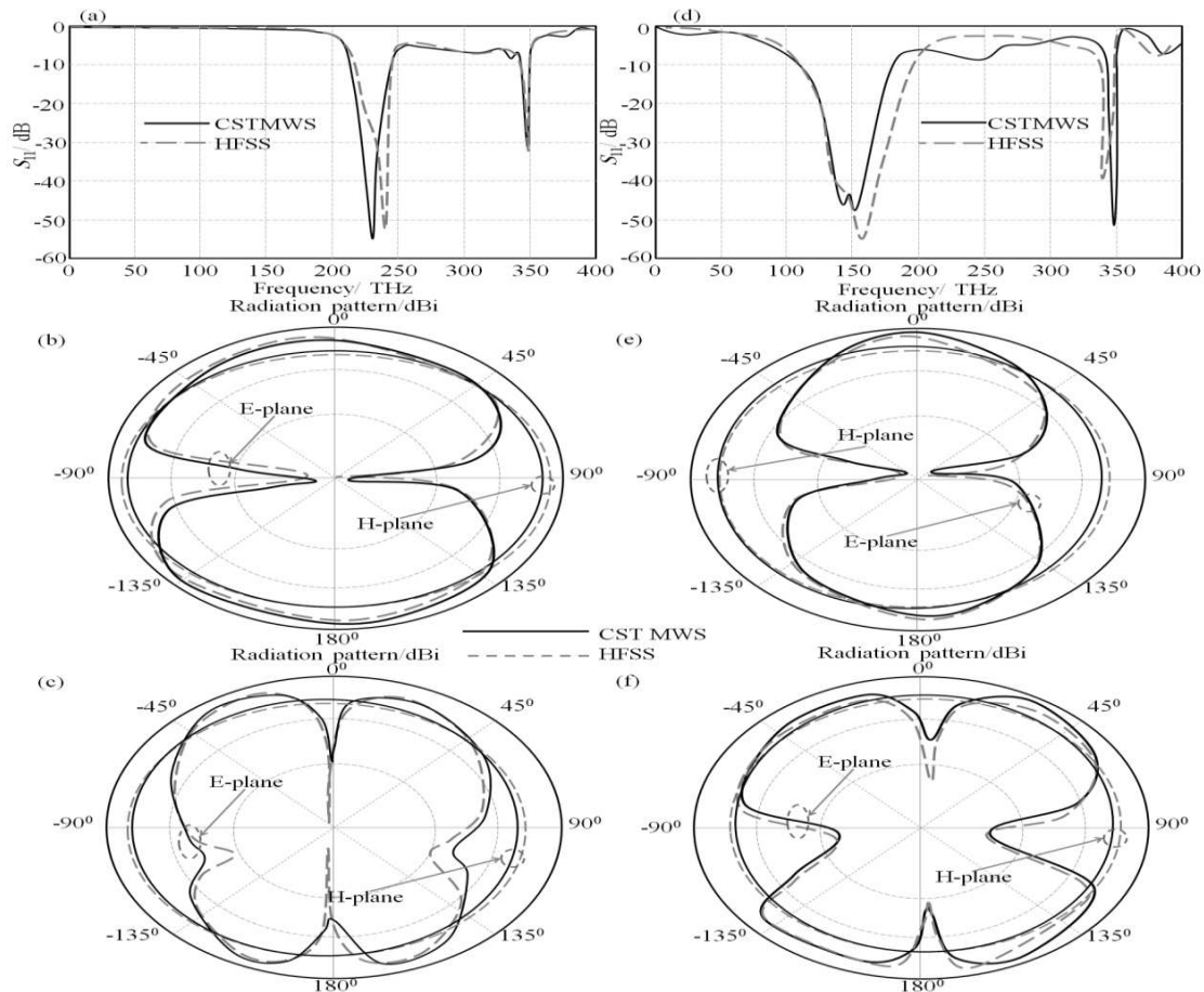
Şekil 3.11. Önerilen SWCNT antenlerinin doğrulama sonuçları; (a) SWCNT_{(10,10)} için S_{11} ve (d) SWCNT_{(21,21)} için S_{11} . (b) ve (c) SWCNT_{(10,10)} için sırasıyla 230THz ve 347THz'de ışınlım
