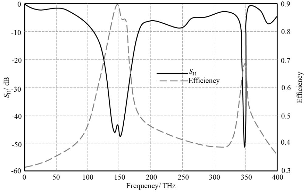
Şekil 4.5. SILICON_1 anteni için S_{11} ve \eta_r spektrumları
