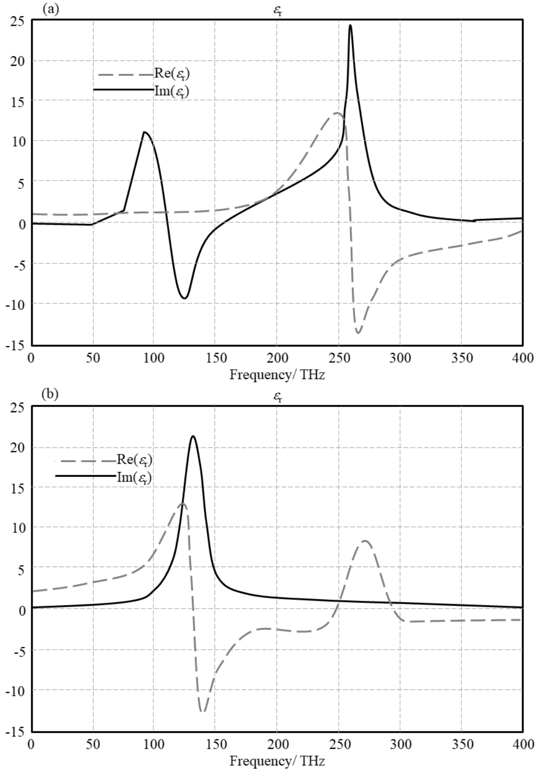
Şekil 3.1. Değiştirilmiş Slepian modeline göre değerlendirilen karmaşık bağlı geçirgenlik: (a) SWCNT (10,10) ve (b) SWCNT (21,21)
