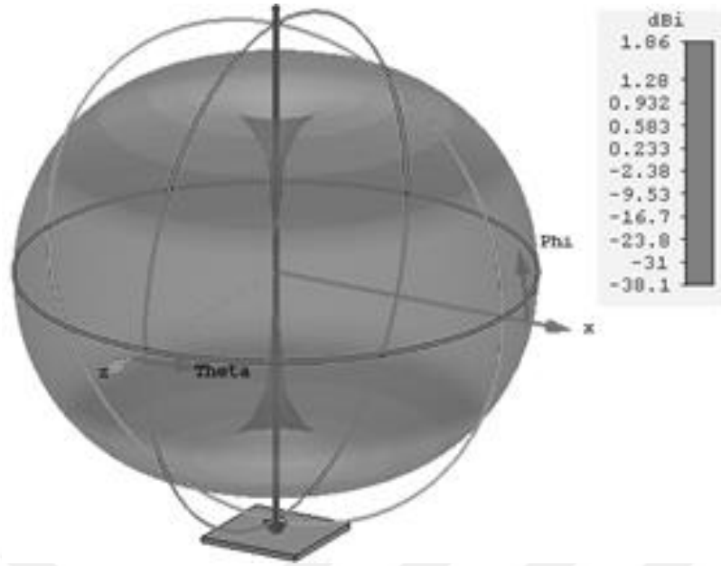
Şekil 4.6. SILICON_1 için 3D radyasyon modeli
