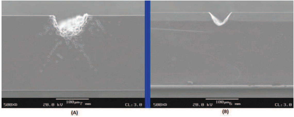
Şekil 4.12. A) Geleneksel yöntemde meydana gelen geniş ısıdan etkilenen bölge, B) Su jeti güdümlü lazer yönteminde meydana gelen dar ısıdan etkilenen bölge [42]
