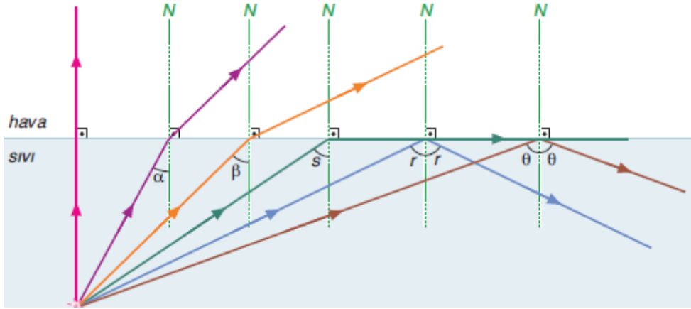
Şekil 3.7. Kritik açı ve tam yansıma [40]
