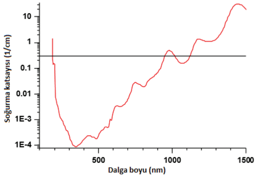
Şekil 4.3. Suyun farklı dalga boylarında lazer ışınına soğurma miktarı [46]
