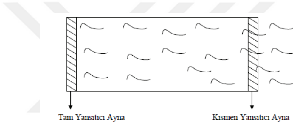
Şekil 2.2. Lazer tüpünün yapısı [5]
