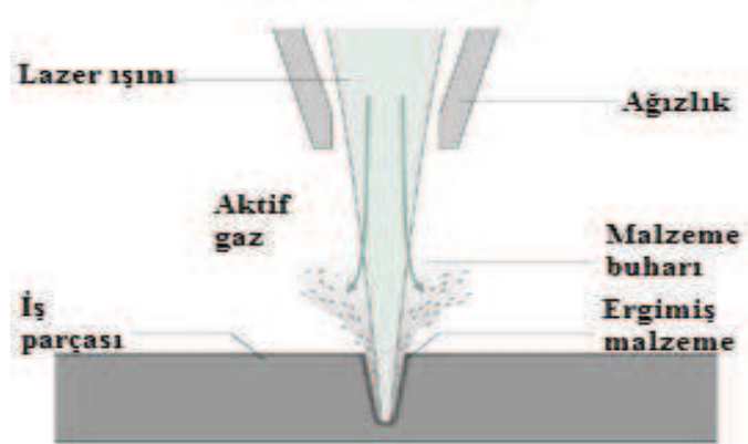
Şekil 2.7. Lazer ışını ile malzeme delme işlemi [20]
