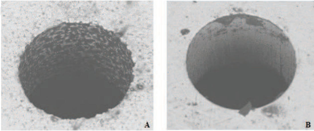
Şekil 4.10. A) Elektro erozyon yöntemi ile delinmiş yakıt püskürtme deliği, B) Su jeti destekli lazer ile delinmiş yakıt püskürtme deliği [42]
