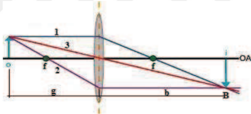
Şekil 3.2. Konveks mercek ile ışın taşınımı, 1: paralel ışın, 2: odak noktası ışını, 3: orta nokta ışını, f:odak noktası, g:sanal uzaklık, b:cismin uzaklığı, B:cismin büyüklüğü
