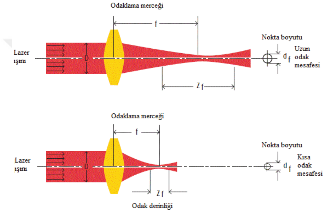
Şekil 3.3. Lazer ışığının odaklanması [37]
