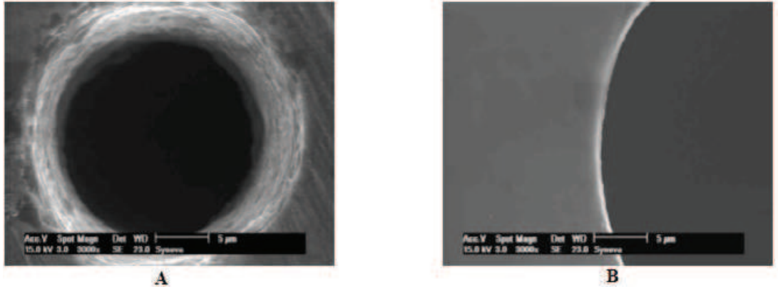
Şekil 4.5. A) Çap ölçüsü: 20μm, kenar kalitesi zayıf, yüzey pürüzlülüğü yüksek delik görüntüsü, B) Çap ölçüsü: 50 μm, keskin kenarlı, yüzey pürüzlülüğü düşük delik görüntüsü [46]
