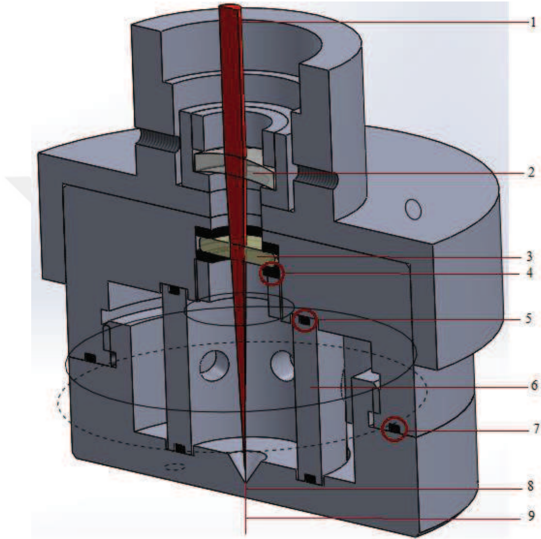
Şekil 5.6. Su jeti başlığı kesit görünüşü
