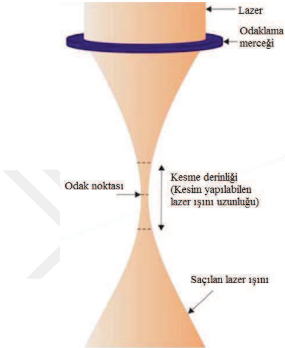
Şekil 5.1. Lazer ışınının odaklanması ve saçılması [44]
