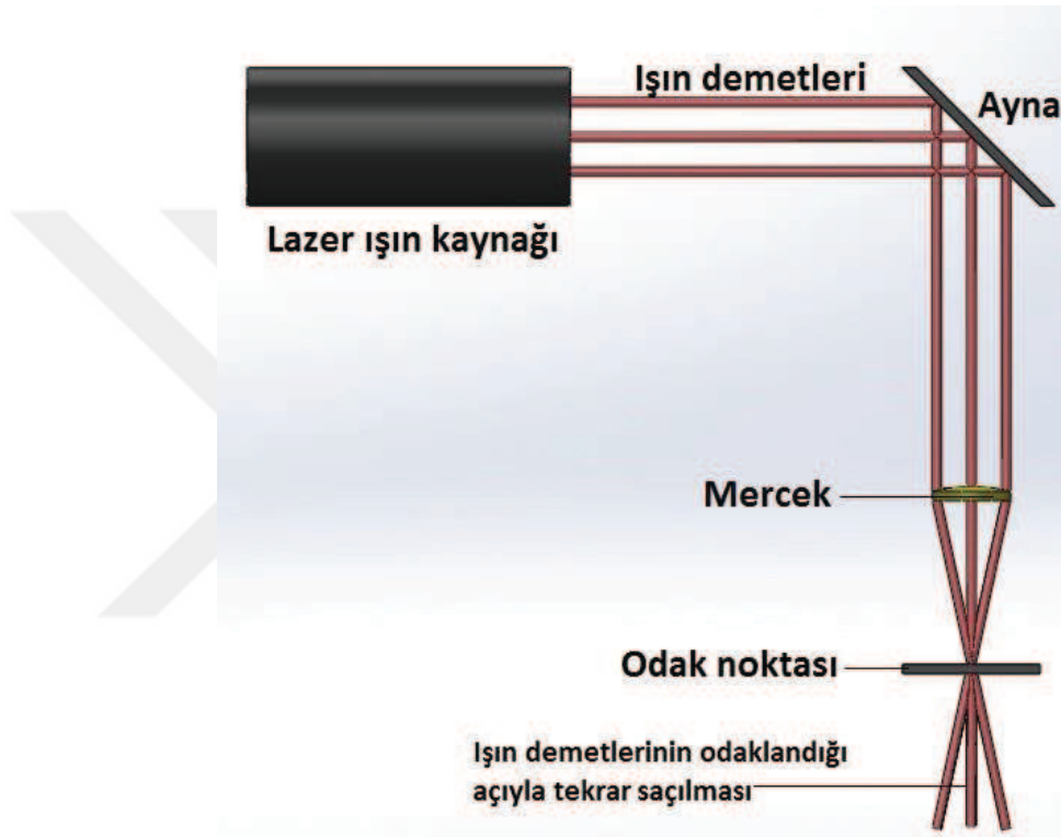
Şekil 1.1. Lazer ışın demetlerinin odaklama işlemindeki davranışı
