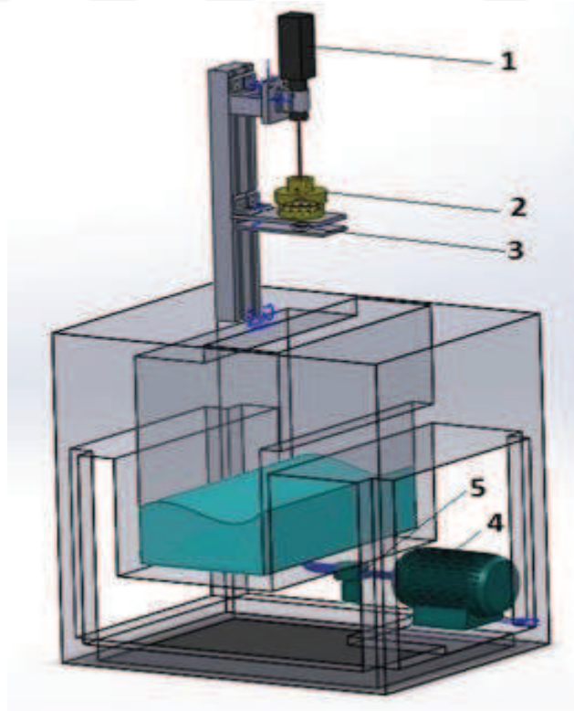
Şekil 5.3. Deney düzeneği şematik görünüm
