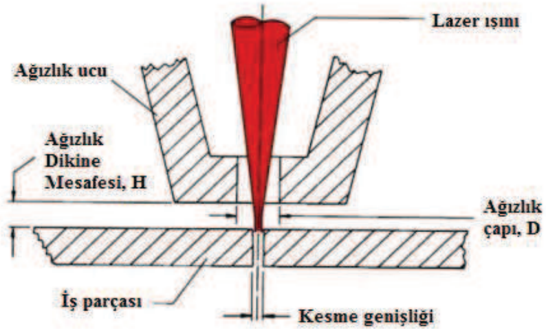
Şekil 2.12. Ağızlık geometrisi ve tanımlamaları [25]
