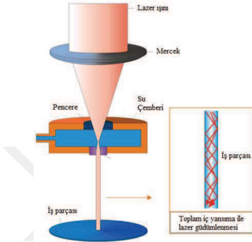
Şekil 4.2. Su jeti destekli lazer sisteminin çalışma prensibi [43]
