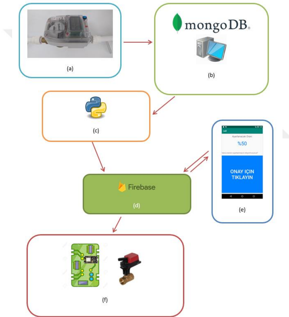
Şekil 3.2. a) Sayaç verileri; b) Sayaç verilerinin server bilgisayardaki veri tabanına iletilmesi; c) Otomasyon programı; d) İnternetteki veri tabanı; e) Android uygulama onayı; f) IOT tabanlı Elektronik Kart ile Oransal Vana Kontrolü
