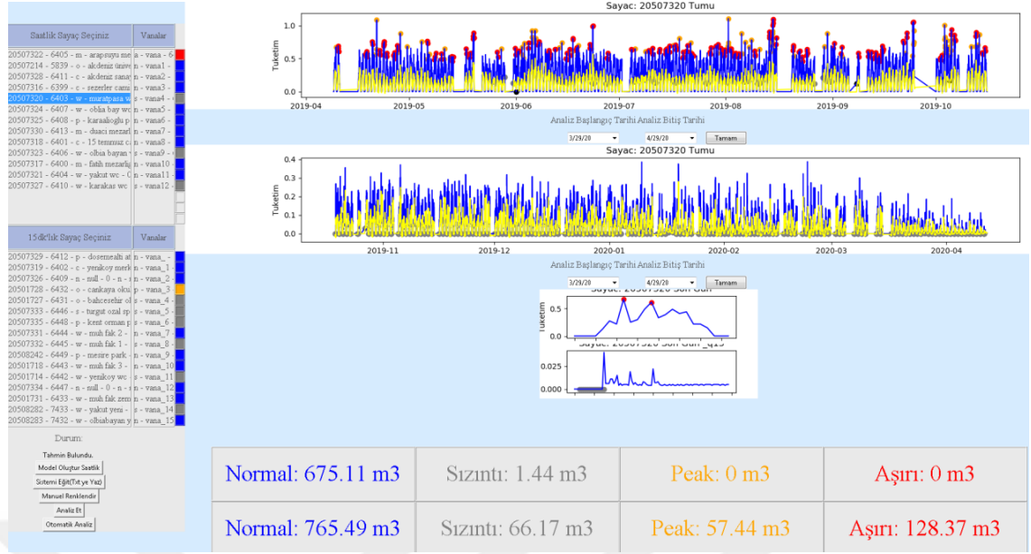
Şekil 4.33. Otomasyon arayüzü
