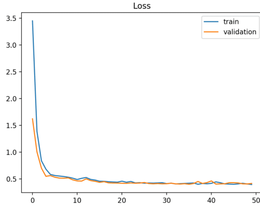
Şekil 3.23. İyi öğrenmeyi gösteren eğitim ve test öğrenme eğrileri örneği
