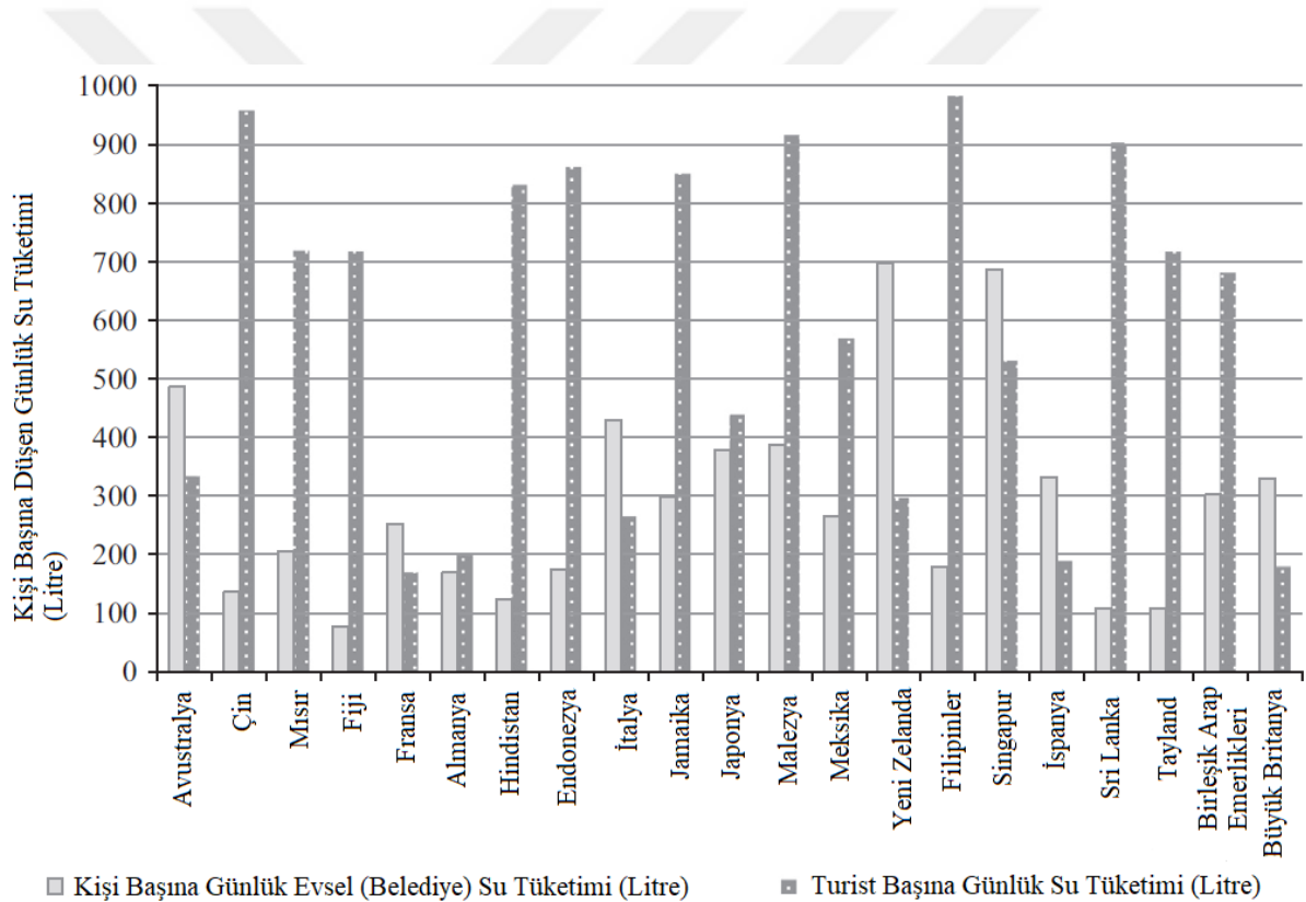
Grafik 1.2 Ükelere Göre Evsel Su Kullanımı ve Turist Su Kullanımı Kıyaslaması
