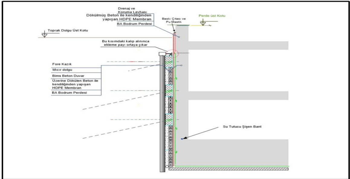
Şekil 4.4. Tek yüz kalıp betonarme perdelerde su yalıtımı detayı
