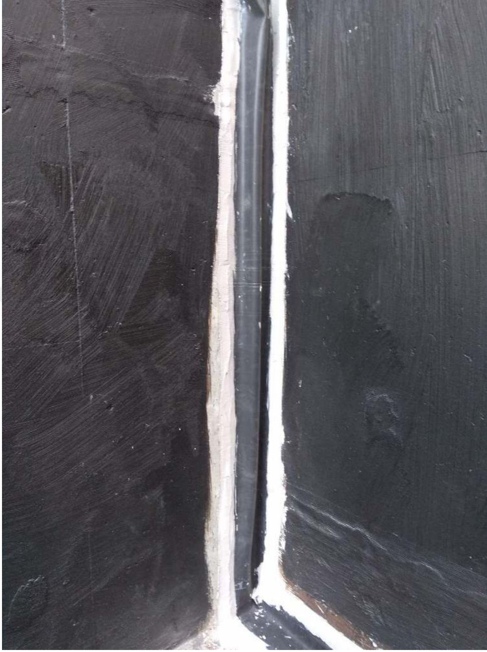
Şekil 4.23. B.A. perdede EPDM bant ile dilatasyon yalıtımı yapılması
