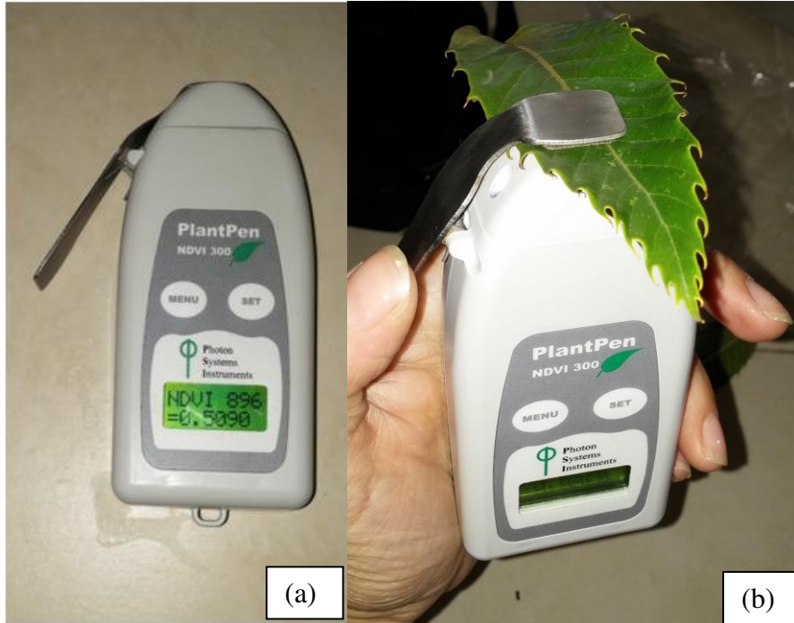
řekil 3.28. (a): PlantPen NDVI 300 cihazı; (b): Kestane yaprađının klorofil yoğunluđunun okunması
