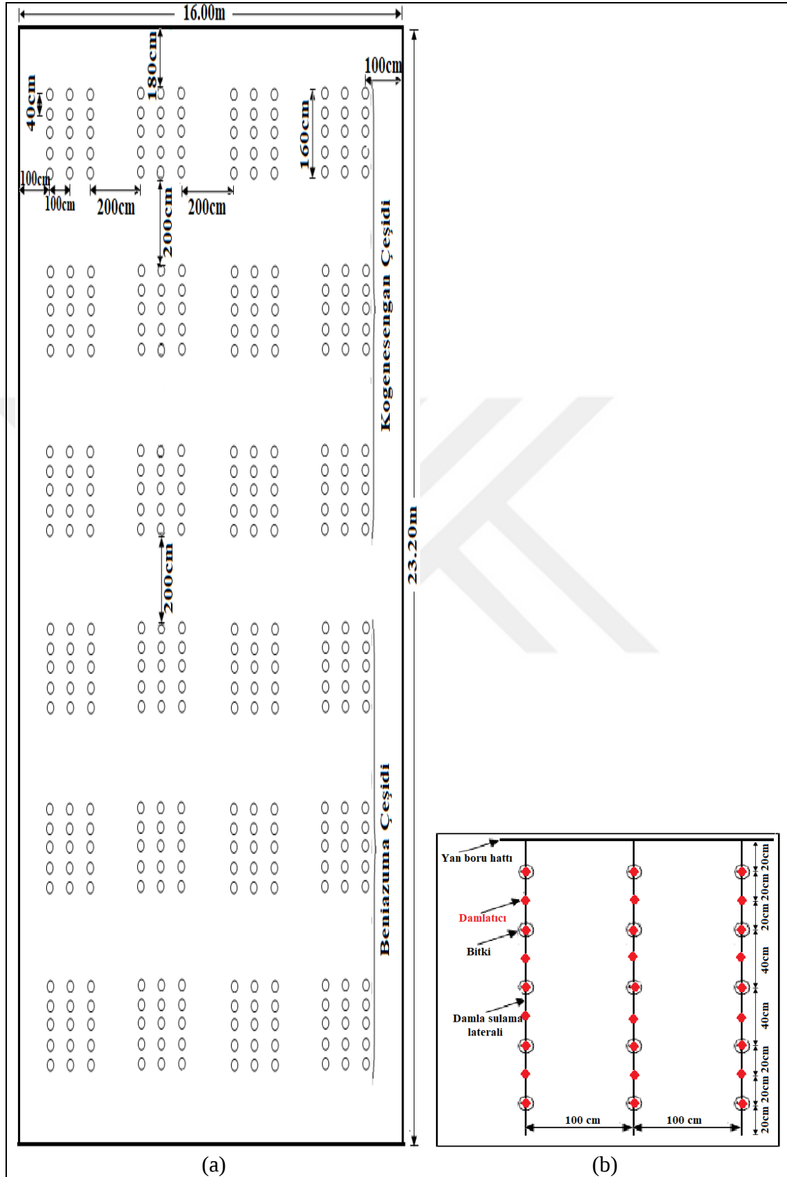
Şekil 3.2. Deneme planı (a) ve bir parseli ait detaylar (b)
