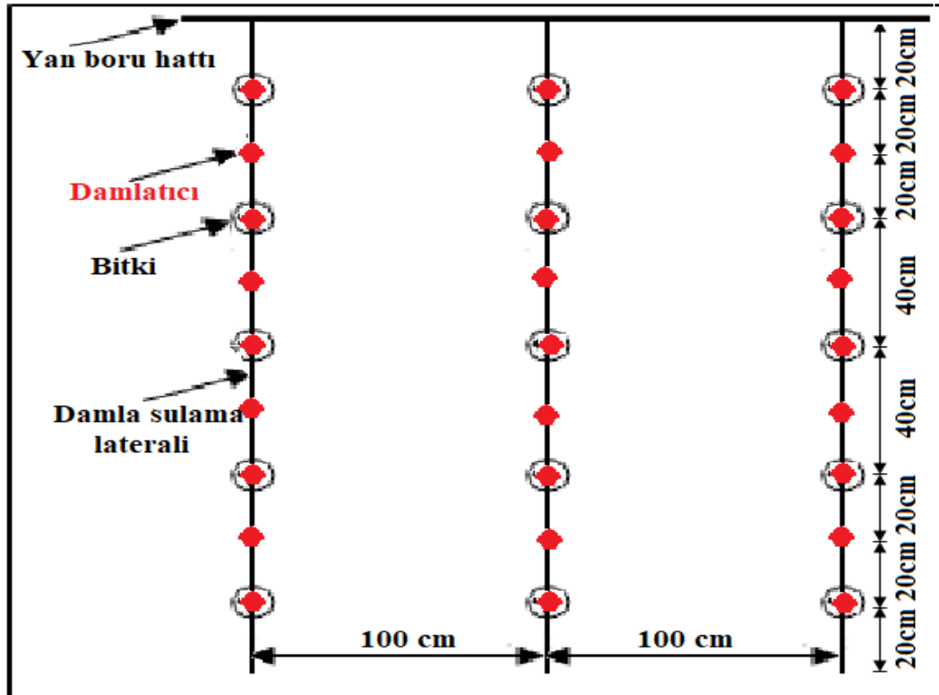
Şekil 3.2. Denemede bir parsele ait detaylar
