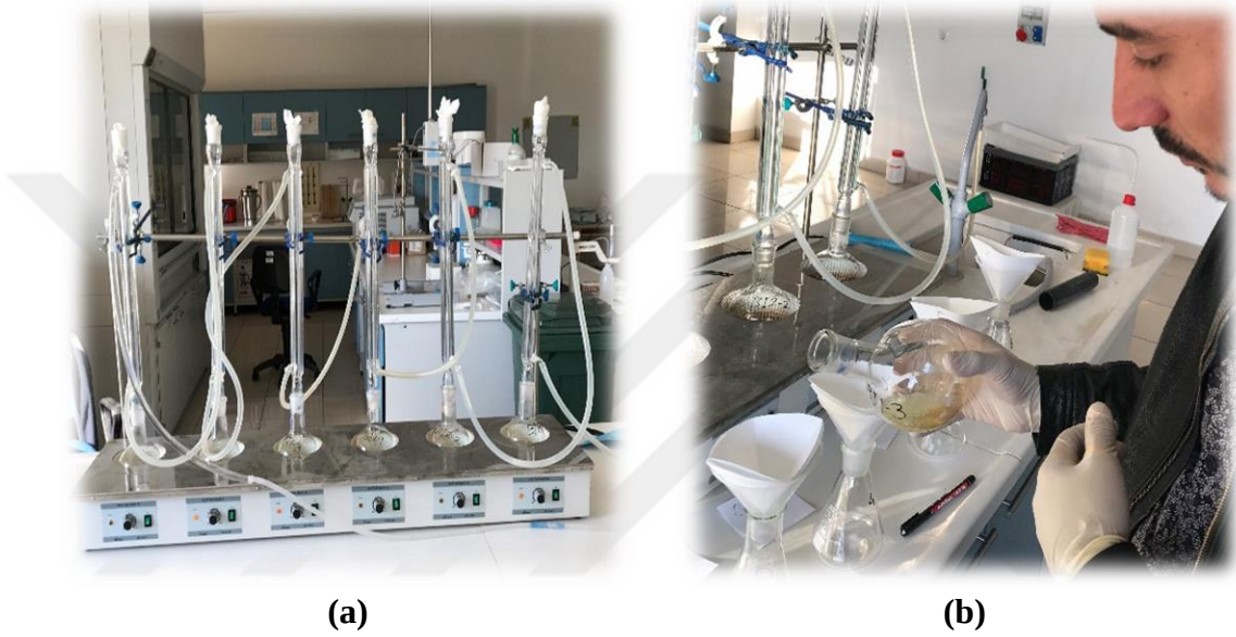
Şekil 3.13. a) Çözeltilerin geri soğutuculu sistemde ısıtılarak kaynaması; b) Kap içeriğinin filtre kâğıtlarına aktarılması
