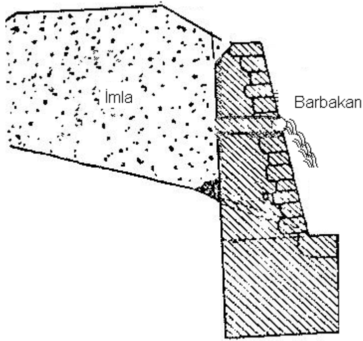
Şekil 7: İstinad duvarı
