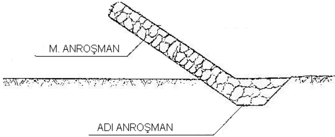
Şekil 11: Muntazam ve Adi Anroşman
