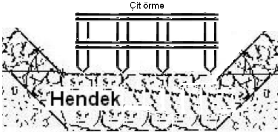
Şekil 9: Çit örülü hendek
