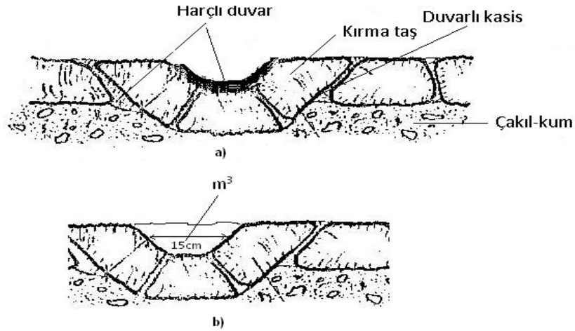
 ekil 6: a) Duvarlı kasis b) Duvarsız kasis
