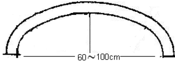
Şekil 3: Basık kemerli menfez
