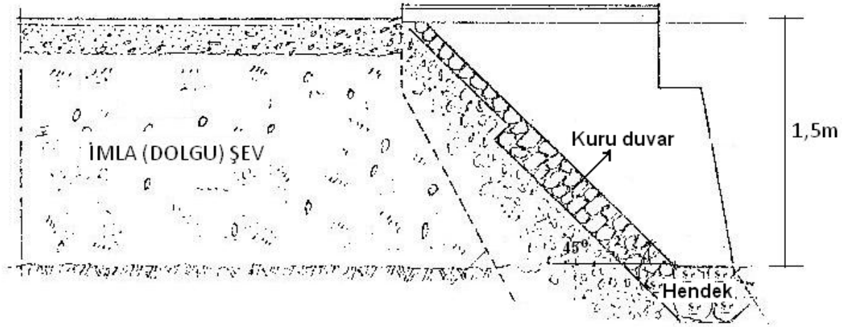
Şekil 5: İmla (Dolgu) Şev
