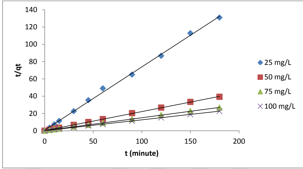
Şekil 5.9.Yalancıİkinci Dereceden Kinetik Model (pH:8)
